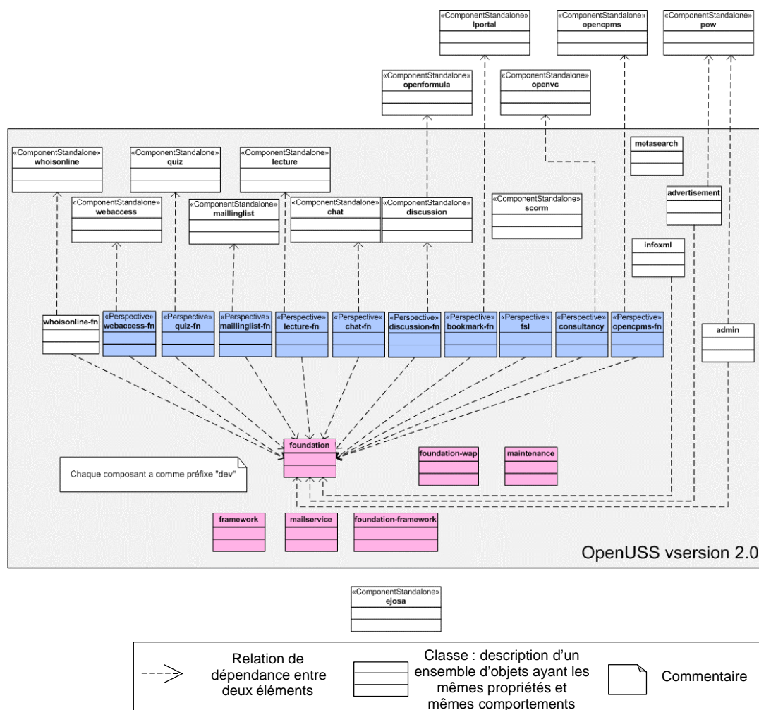
Figure 56 : Diagramme UML de classe des composants d'OpenUSS 51
