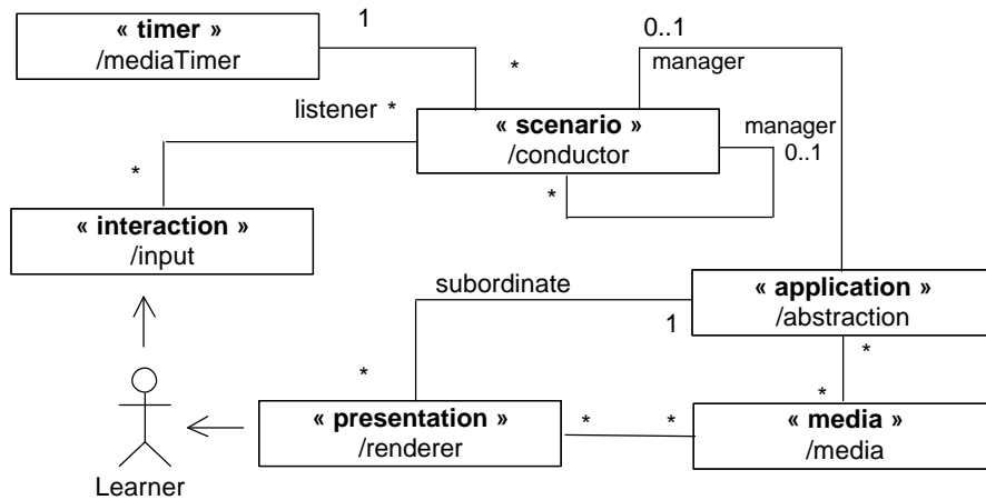
Figure 51 : Diagramme de classe UML représentant le Profil pour les applications multimédias [(Sauer et Engels 2001), figure 3]
