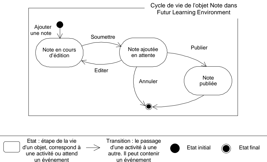
Figure 47 : Diagramme état-transition UML de l'objet considéré pour FLE
