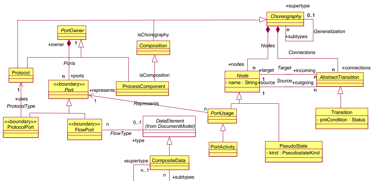
Figure 71 : Eléments extraits de la structure du méta-modèle du profil UML [(OMG/ECA 2004), figures 3-5 et 3-7]
