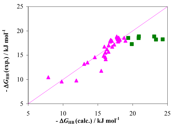
Fig. 5 - Corrélation entre basicité de liaison H expérimentale et calculée par l'équation [6] pour la famille des amines. La droite \Delta G_{\text{HB}}(\text{exp.}) = \Delta G_{\text{HB}}(\text{calc.}) est indiquée. Les amines exclues pour cause de chélation sont montrées (■).
