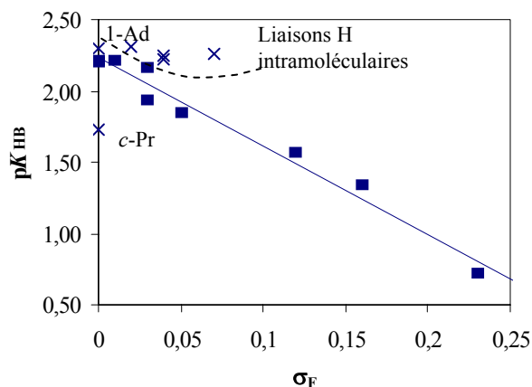
Fig. 3 - Relation entre pK_{\text{HB}} et la constante inductive \sigma_{\text{F}} du substituant X des amines primaires \text{XNH}_2 . La cyclopropylamine 12 (effet de résonance ?), la 1-adamantanamine 2 (effet de polarisabilité), l'éthylènediamine 14 , la 1,3-diaminopropane 13 , la 2-méthoxyéthylamine 17 et la 3-méthoxypropylamine 18 (liaison H intramoléculaire) sont exclues de la corrélation.
