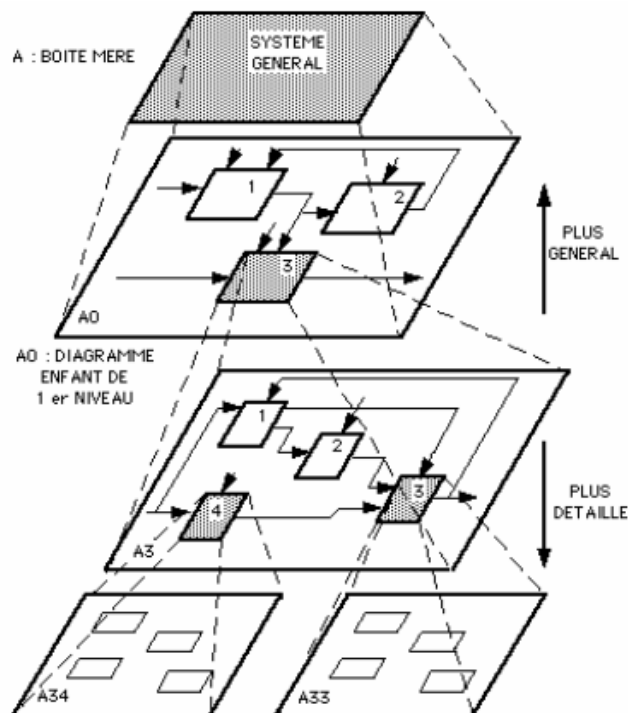
Figure 2.5 : Décomposition d'un processus selon la méthode SADT
