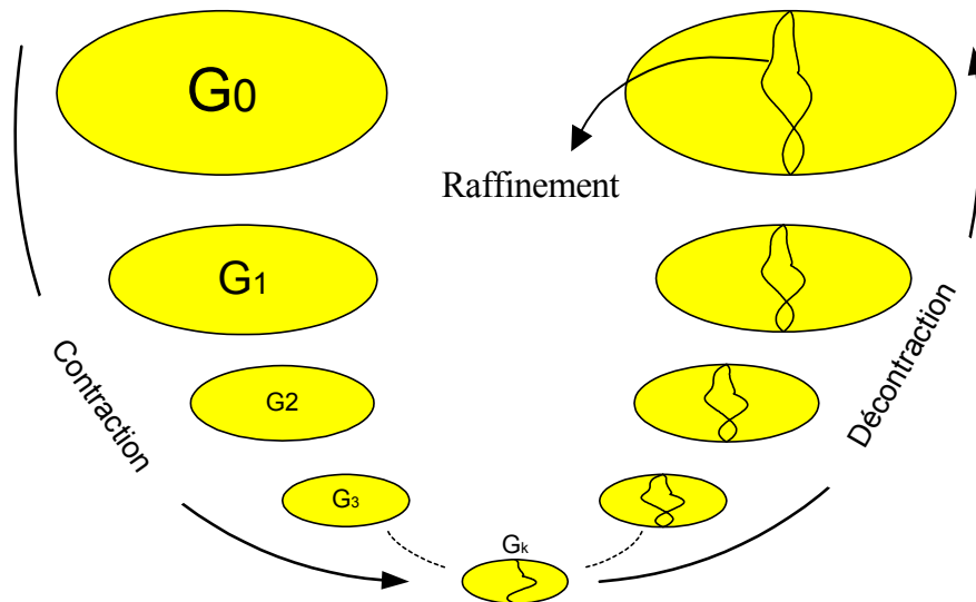
Figure 2.16 : Algorithme multi-niveaux
