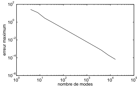
Figure 4.4 – Erreur commise par la troncature
