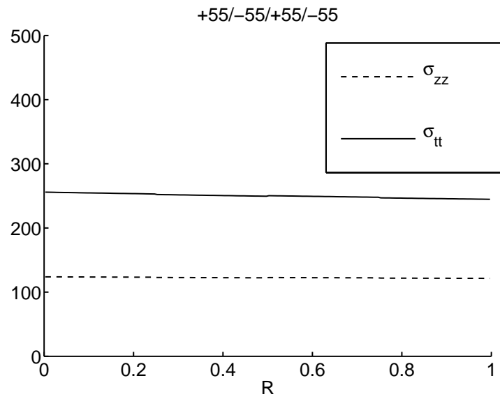
Figure 2.10 – Évolution des contraintes circonférentielle et axiale (en MPa) en fonction de R
