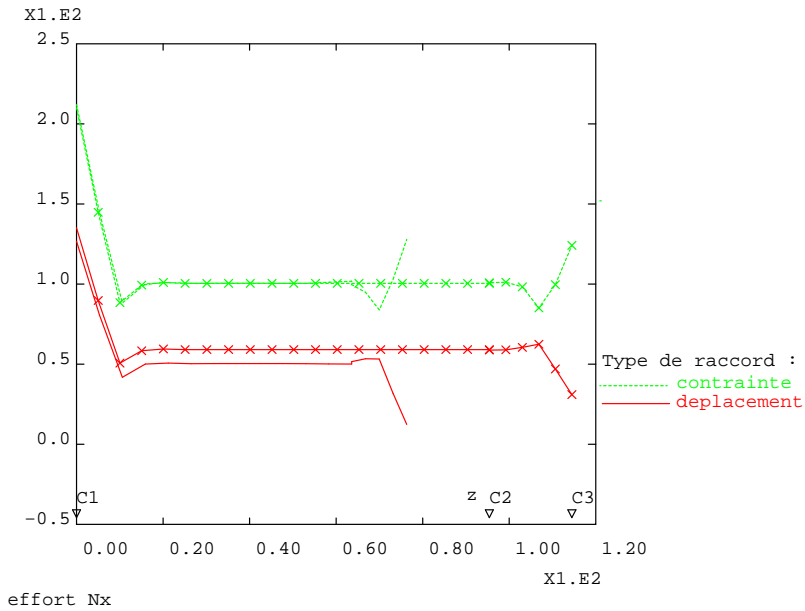
Figure 2.6 – Évolution de T_X suivant l1 : cas homogène isotrope
