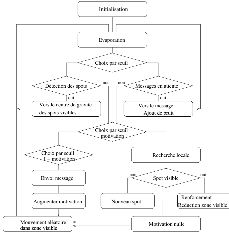
FIG. 3.14 – L’algorithme HCIAC.
