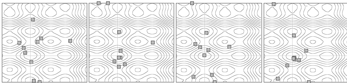
FIG. 3.5 – CIAC optimisant la fonction B_2 uniquement avec le canal “piste”, quatre étapes consécutives sont montrées (après une centaine d’évaluations de la fonction objectif).
