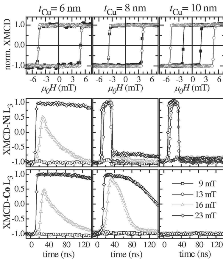
Figure 3.2: Haut: cycles d'hystérésis quasi-statiques et sélectifs mesurés par XMCD pour les couches de \text{Fe}_{20}\text{Ni}_{80} (carrés noirs) et Co (points blancs); (bas) variation temporelle du signal XMCD pour les deux couches ferromagnétiques, mesurée pour les trois vannes de spin pour des impulsions de 30 ns de durée et d'amplitude variable.
