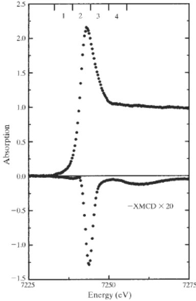
Figure 1.8: Spectre d'absorption et XMCD d'une couche de \text{GdCo}_5 mesuré avec la lame de diamant au seuil L_3 du Gd sur la ligne ID24.
