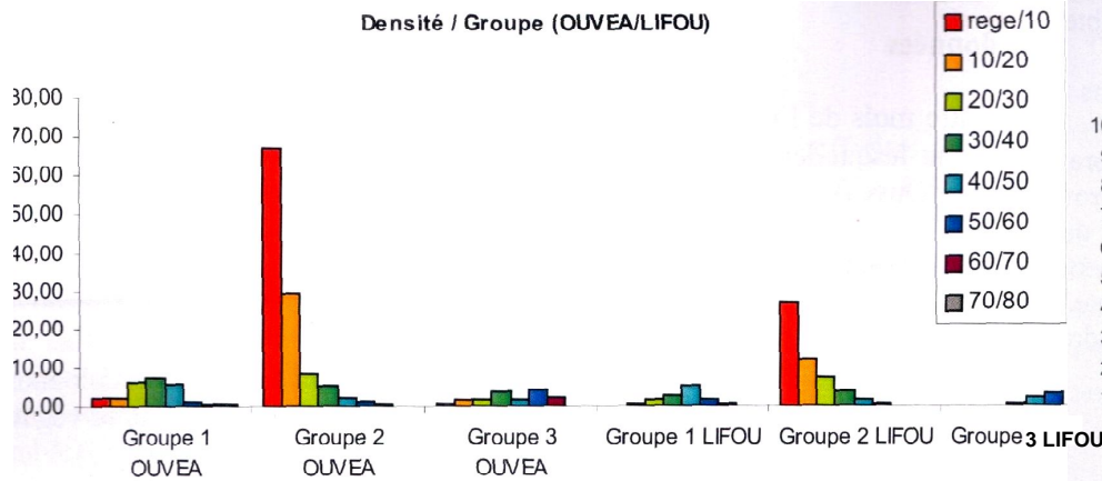
Figure 1.14: Groupes démographiques établis suite aux inventaires de Ouvéa et Lifou (a) (Steierer, 2004), et de Maré (b)(Brinkert, 2003). Répartition de ces groupes de peuplement selon les îles pour Ouvéa et Lifou (c). Distribution relative des placettes inventoriées par groupe de structure au sein de chaque population sur Maré (d).
