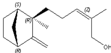
Sesquiterpénoïde \beta -santalol
