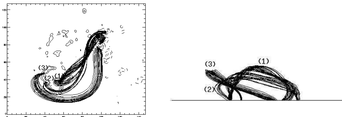
FIG. III.17 – Tubes de flux caractéristiques de la région active 8151 dans l'hypothèse d'un champ sans-force non linéaire : vue de dessus (à gauche), vue de côté (à droite). Les contours en traits pleins (resp. traits pointillés) représentent les valeurs positives (resp. négatives) du champ magnétique.
