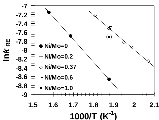
Figure I-11. Droites d'Arrhénius pour la réaction de libération de H 2 S à partir de MoS 2 (16 %pds de MoO 3 ) et NiMoS calculées à partir des résultats d'expériences d'HDS du [ 35 S]DBT. Le point entre parenthèses correspond à un catalyseur possédant un rapport Ni/Mo supérieur au rapport optimal (c-à-d avec des performances en HDS diminuées) [20*].
