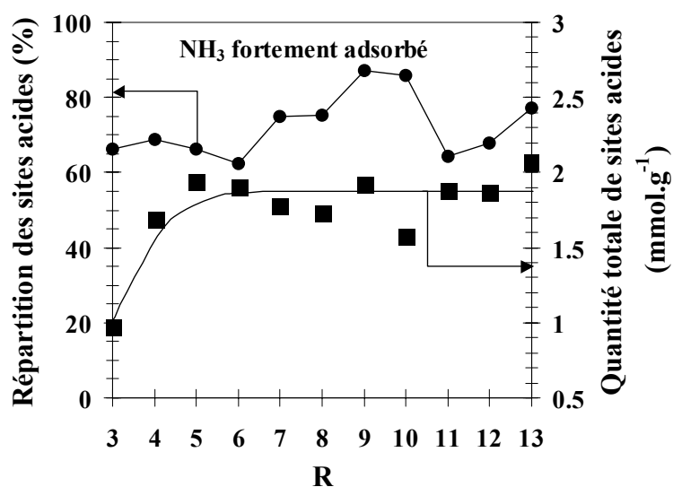
Figure I-4. Quantité totale de sites acides et contribution relative de \text{NH}_3 fortement adsorbé pour toute la gamme des rapports d'hydrolyse R utilisés [39*].
