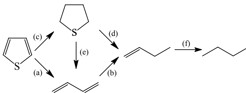
Figure II-1 : Schéma ‘classiquement’ (voir la remarque page précédente) admis de la réaction d’hydrodésulfuration du thiophène. La voie (a) est l’hydrogénolyse directe, la voie (c) correspond à une étape d’hydrogénation suivie par une hydrogénolyse (d) ou (e).
