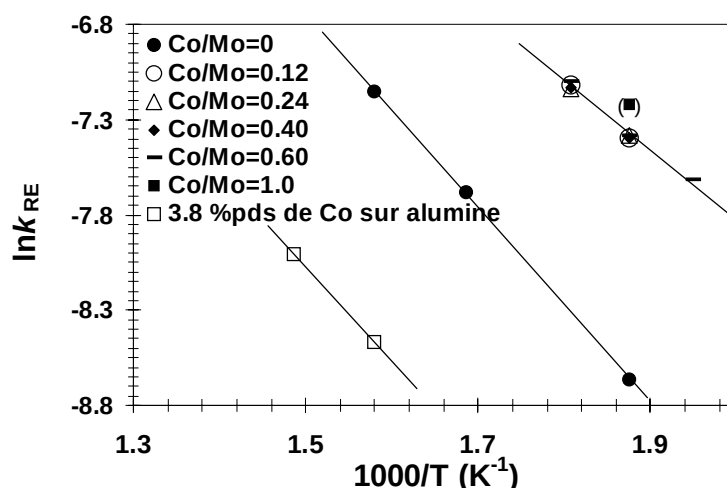
Figure I-10. Droites d'Arrhénus pour la réaction de libération de \text{H}_2\text{S} à partir de \text{MoS}_2 (16 %pds de \text{MoO}_3 ), \text{CoMoS} et \text{Co}_9\text{S}_8 (3,8 %pds Co sur \text{Al}_2\text{O}_3 ) calculées à partir des résultats d'expériences d'HDS du [\text{}^{35}\text{S}]\text{DBT} [20*].
