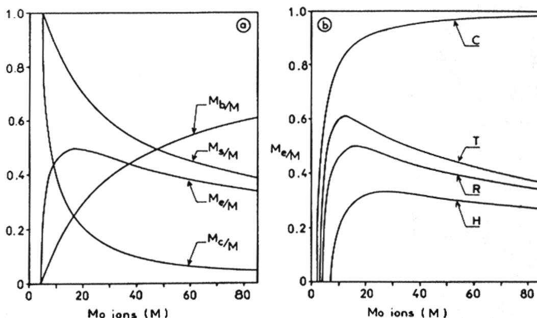
Figure I-3. Rapport \text{Mo}_{\text{bord}} / \text{Mo}_{\text{total}} en fonction du nombre total de Mo dans un feuillet de \text{MoS}_2 [203].
