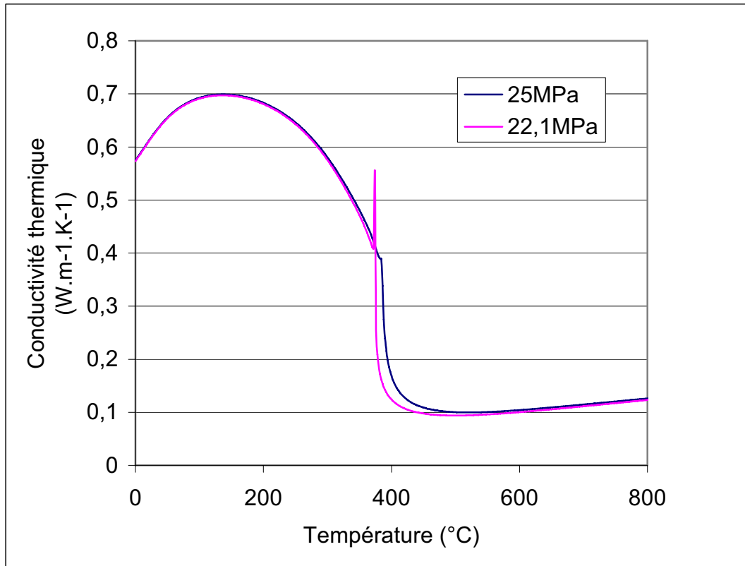
Figure 6 : Variation de la conductivité thermique de l'eau pure en fonction de la température pour P=25\text{MPa} et P=22,1\text{MPa}
