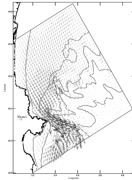
Fig. 5.33 – Champ de courant ( \text{cm s}^{-1} ) de fond simulé pour le 22 février 2004 à 0 h.
