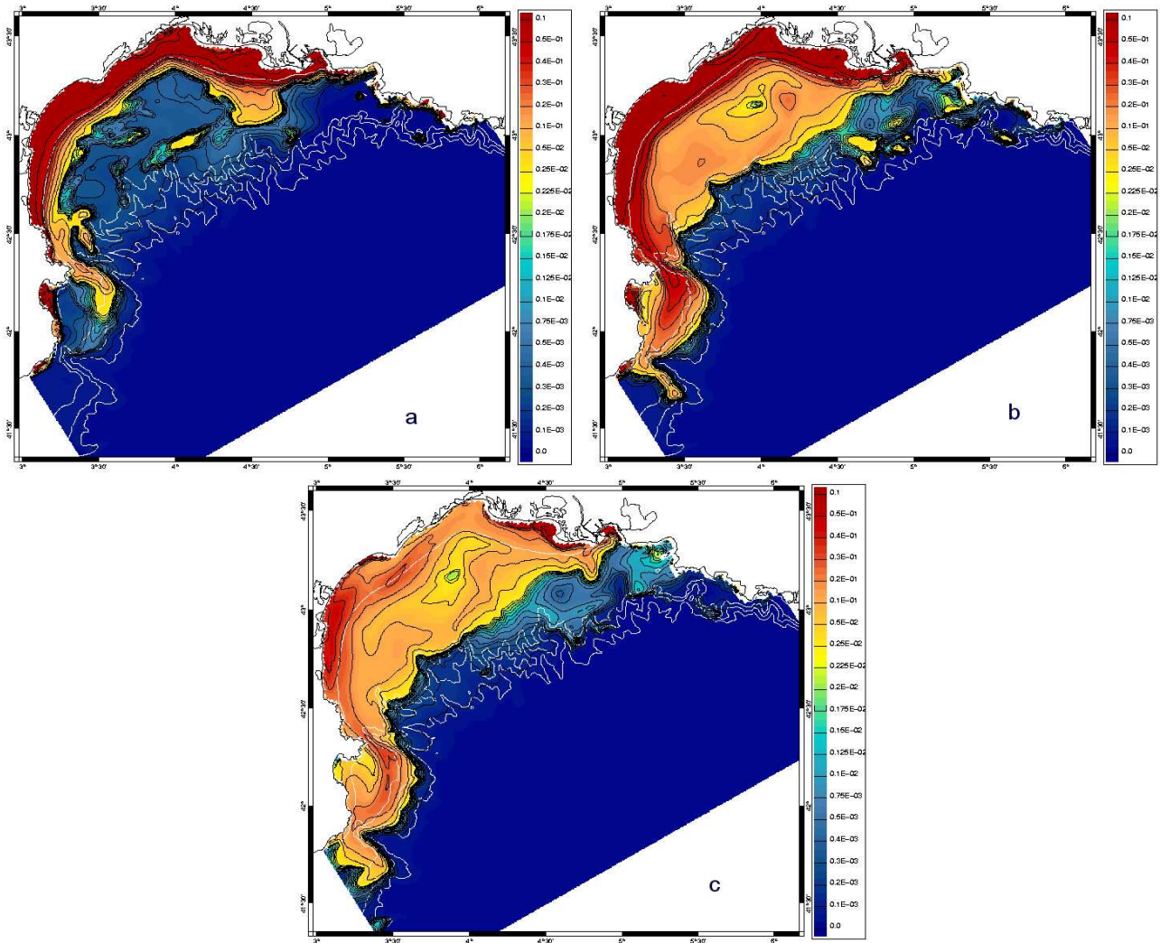
Fig. 6.23 – Champs de concentration de matière en suspension ( \text{g L}^{-1} ) près du fond simulés pour le 21 février (a), le 22 février (b) et le 23 février (c) 2004. Les lignes blanches correspondent aux isobathes 50, 200, 500 et 1000 m.
