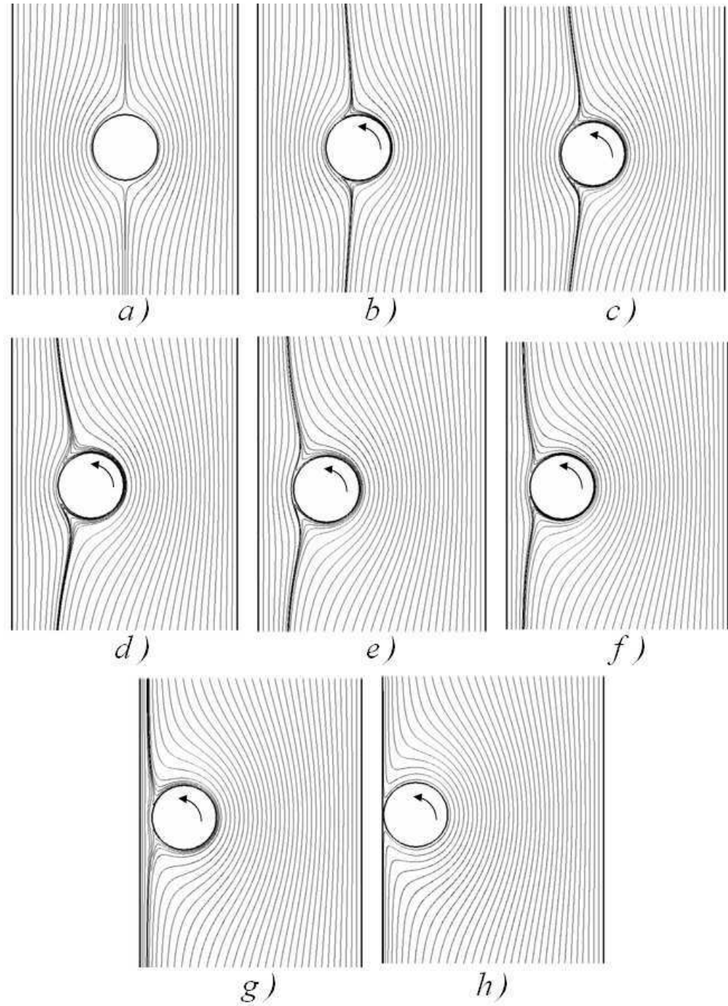
FIG. 5.12 – Lignes de courant autour d'un cylindre libre en sédimentation pour k = 0.29 dans un référentiel lié au cylindre pour e/e_{max} = : a) 0 - b) 0.141 - c) 0.282 - d) 0.423 - e) 0.563 - f) 0.704 - g) 0.845 - h) 0.986. L'accélération de la pesanteur est verticale descendante et le cylindre se déplace vers le bas
