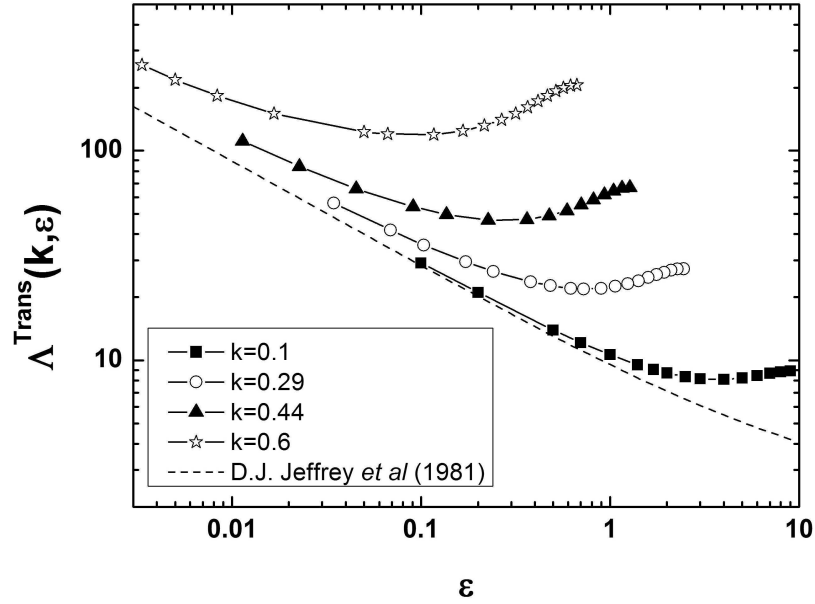
FIG. 4.11 – \Lambda^{Trans}(e/e_{max}) en fonction de h^-/a
