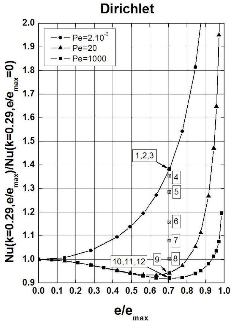
FIG. 3.2 – Flux normalisé en fonction de e/e_{max} pour différents Pe (conditions aux limites de type Dirichlet). Les points ont les mêmes étiquettes que sur la figure 3.3
