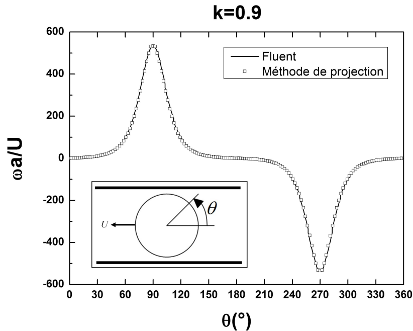
FIG. 2.8 – Comparaison entre différentes approches - Distribution angulaire de la vortécité sur le cylindre pour k = 0.9
