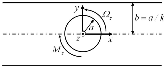
FIG. 3.18 – Schéma du problème du cylindre en rotation
