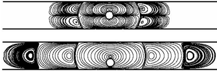
FIG. 4.18 – Lignes de courant autour du cylindre en translation uniforme dans un repère fixe pour k = 0.29 et Re = 0.1 . En-haut : e/e_{max} = 0 - En-bas : e/e_{max} = 0.704
