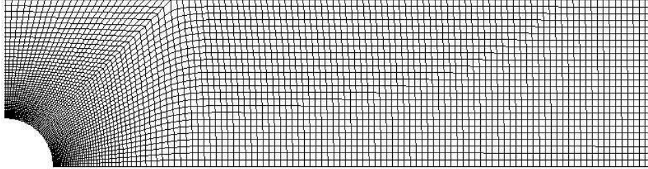
FIG. 2.5 – « Maillage type » obtenu avec Gambit pour k = 0.29
