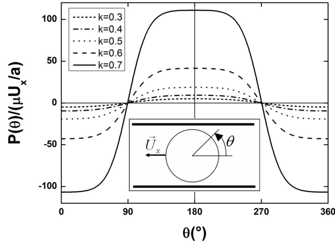
FIG. 3.10 – Répartition angulaire de la pression sur le cylindre
