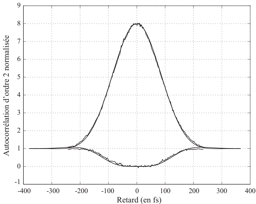
FIG. 4.2 – Exemple d'interpolation d'une trace d'autocorrélation ( \lambda = 780 \text{ nm} ).
