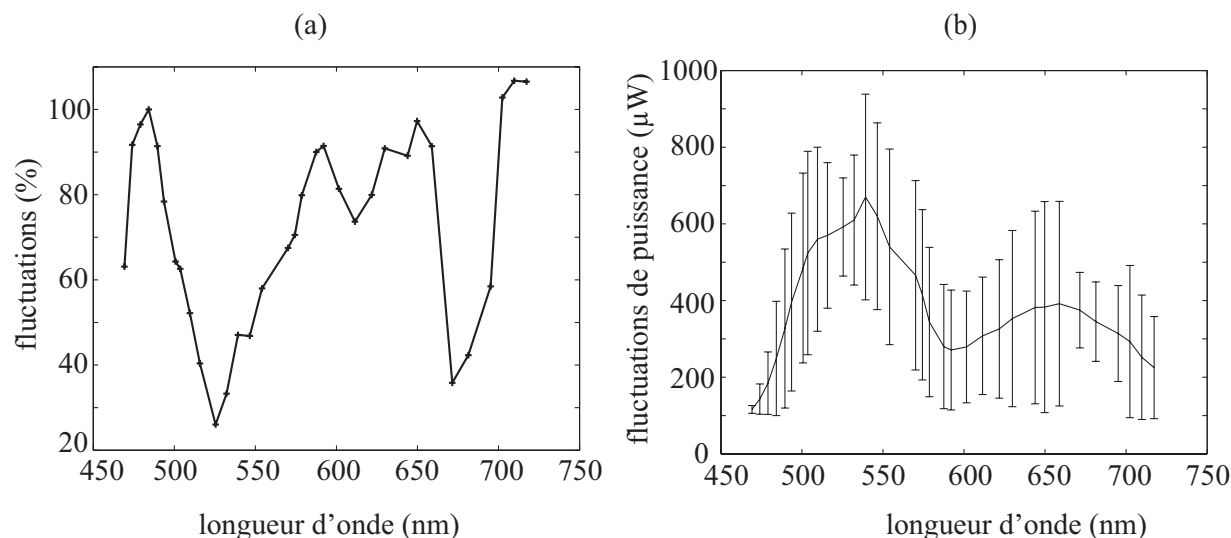
FIG. 1.30 – (a) Spectre des fluctuations de puissance du continuum (en %), (b) Spectre des fluctuations de puissance du continuum (en \mu\text{W} ) et spectre de la puissance moyenne.
