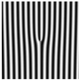
figure d'interférences
