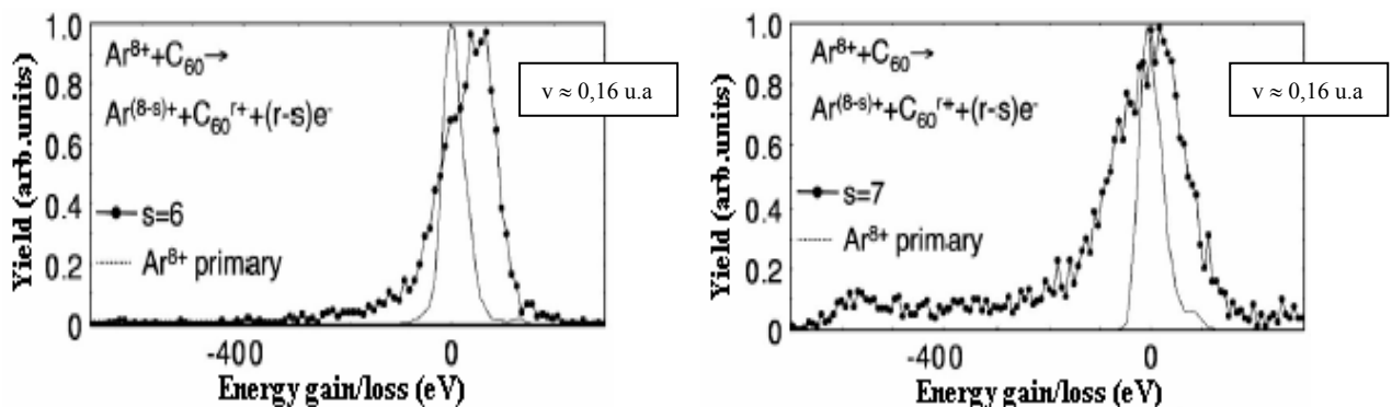
Figure (29) : perte et gain en énergie de l' Ar^{8+} ayant stabilisé 6 et 7 électrons [Cederquist et al] [ref.75]
