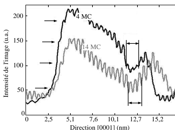
FIG. 5.6 : Profils d'intensité moyenne des images haute résolution TEM en balayage, selon la direction [0001]. Les flèches simples indiquent la transition entre AIN et GaN au dessus des îlots. Les double-flèches mettent en évidence les plans AIN de la couverture d'AIN entre les îlots et le marqueur GaN.
