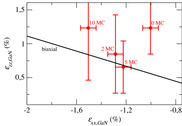
FIG. 6.12 : Déformation dans le plan \varepsilon_{xx, GaN} déterminée par les mesures MAD, en fonction de la déformation hors du plan \varepsilon_{zz, GaN} déterminée par EDAX, pour les échantillons synthétisés sur substrats AlN/saphir. La droite représente le cas d'une couche de GaN en contrainte biaxiale.
