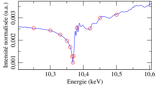
FIG. 2.18 : Intensité diffractée normalisée en fonction de l'énergie, et exemple de choix judicieux d'énergies (cercles)
