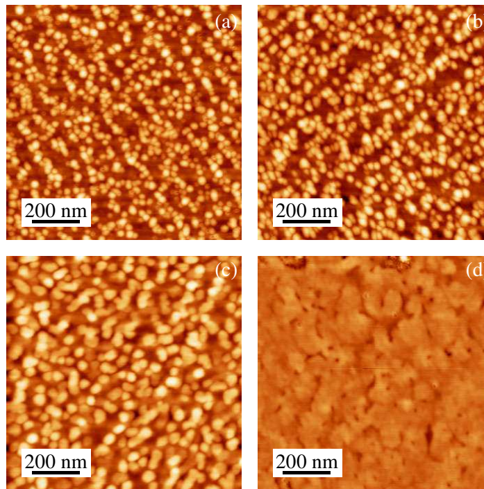
FIG. 5.1 : Topographies AFM de 1 \mu m^2 , d'un plan de boîtes non recouvert (a) et de plans de boîtes recouverts par 4 (b), 11 (c) et 18 (d) MC d'AlN.
