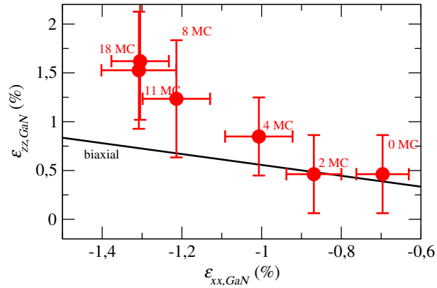
FIG. 6.11 : Déformation dans le plan \varepsilon_{xx, GaN} déterminée par les mesures MAD, en fonction de la déformation hors du plan \varepsilon_{zz, GaN} déterminée par EDAFS, pour les échantillons synthétisés sur SiC. La droite représente le cas d'une couche de GaN en contrainte biaxiale.
