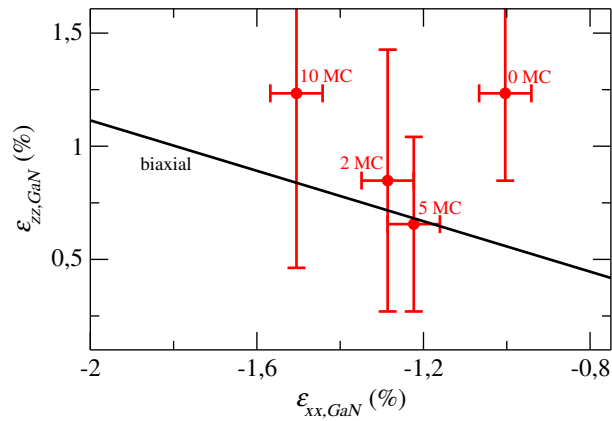
FIG. 6.12 : Déformation dans le plan \varepsilon_{xx, GaN} déterminée par les mesures MAD, en fonction des de la déformation hors du plan \varepsilon_{zz, GaN} déterminée par EDAFS, pour les échantillons synthétisés sur substrats AlN/saphir. La droite représente le cas d'une couche de GaN en contrainte biaxiale.
