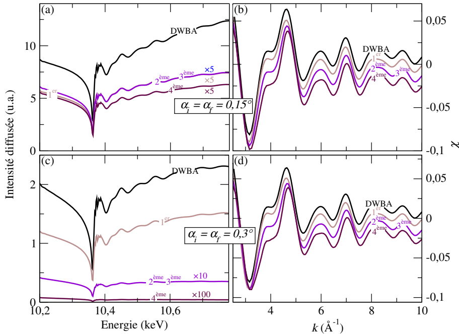
FIG. 2.34 : Spectres DAFS calculées en fonction de l'énergie au voisinage de la réflexion (3030) pour chacun des quatre chemins, pour un îlot pyramidal de GaN déposés sur une multicouche (GaN + AlN + substrat SiC). Les deux cas correspondent à \alpha_i = \alpha_f = 0,15^\circ et \alpha_i = \alpha_f = 0,3^\circ .
