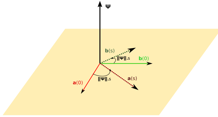
FIG. D.1: Rotation à vitesse constante autour de \Psi de la base (\mathbf{a}, \mathbf{b}) .
