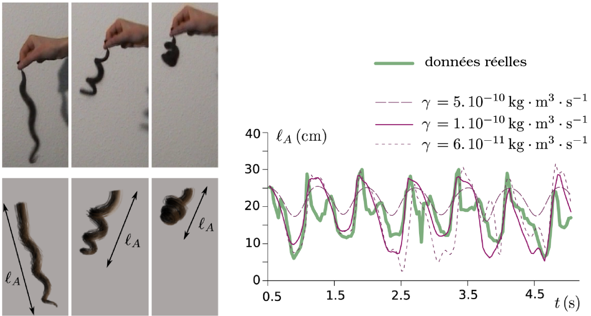
FIG. 7.9: Ajustement de \gamma sur un mouvement oscillatoire vertical d'une mèche bouclée et disciplinée. À gauche, comparaison entre l'expérience réelle (en haut) et virtuelle (en bas). À droite, on compare la longueur apparente \ell_A de la mèche entre les données réelles et les données simulées, pour différentes valeurs de \gamma . Dans ce cas précis, des résultats qualitativement similaires sont obtenus en choisissant \gamma = 1.10^{-10} \text{ kg} \cdot \text{m}^3 \cdot \text{s}^{-1} .
