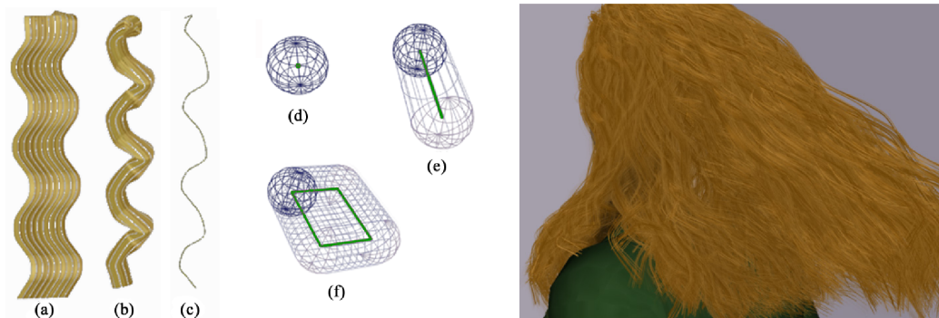
FIG. 1.35: Représentation par niveaux de détail de la chevelure [WLL + 03]. À gauche : (a) bande de cheveux 2D, (b) groupe de cheveux 3D, (c) cheveu individuel, et algorithmes de balayage de sphères pour la détection de collision : (d) balayage sur un point, (e) balayage sur une ligne, (f) balayage sur un rectangle [WLL + 03]. À droite, cheveux longs et bouclés flottant dans le vent, représentés par différents niveaux de détail.
