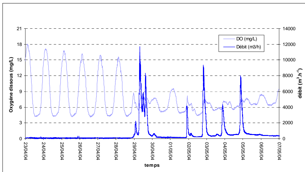
Figure 57 : Comparaison de l'oxygène dissous des eaux de rivière et du débit au niveau de l'exutoire.
