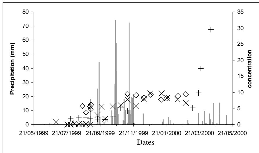
Figure 30: Evolution des concentrations de « nutriment » au pont de La Clue (x: nitrate en \text{mg.L}^{-1} , +: silicium en \mu\text{g.L}^{-1} divisé par 100 et o: oxygène en \text{mg.L}^{-1} ) au cours de l'étude annuelle (1999 – 2000).
