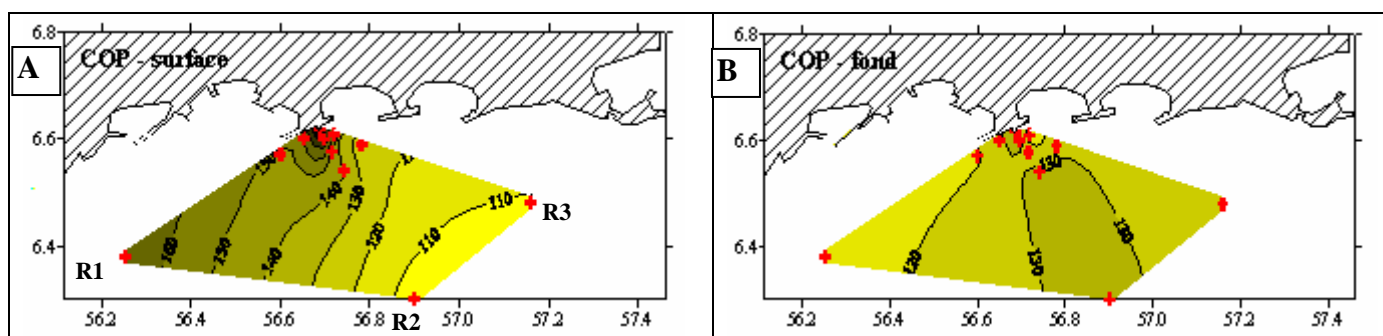
Figure 53 : Répartition du COP (en µg.L -1 ) dans la rade des Vignettes lors de la campagne de prélèvement "point zéro" (A) : COP surface, (B) : COP à 1m du fond (Ri : Radiale n° i)
