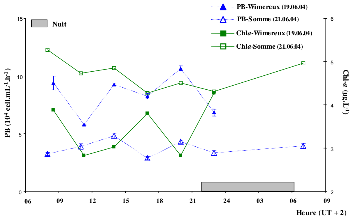
Figure III.7 : Evolution des productions bactériennes (PB) et des concentrations en chlorophylle a (Chl-a) au cours d'une dérive de masse d'eau à Wimereux (figurés pleins) et en baie de Somme (figurés vides). Les barres d'erreur correspondent aux écart-types mesurés sur les productions bactériennes.
