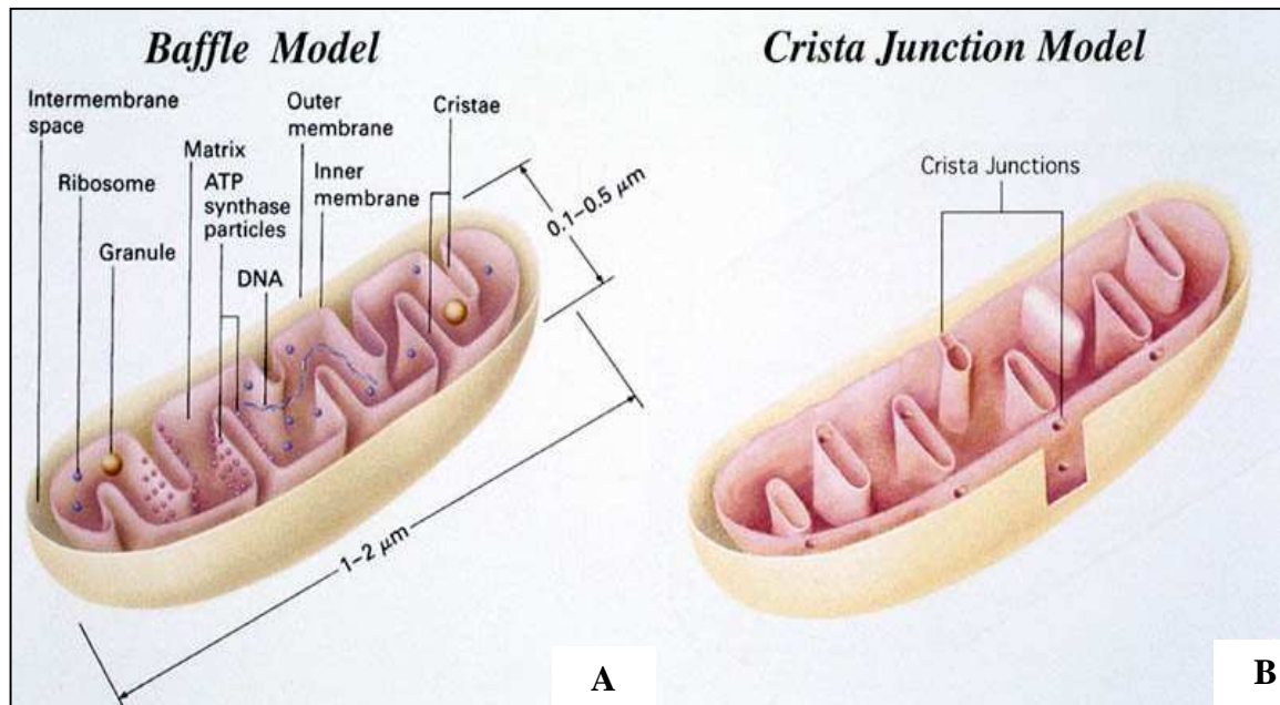
Figure 9 : Modèles de structures des membranes mitochondriales (Perkins et al. , 2000).
