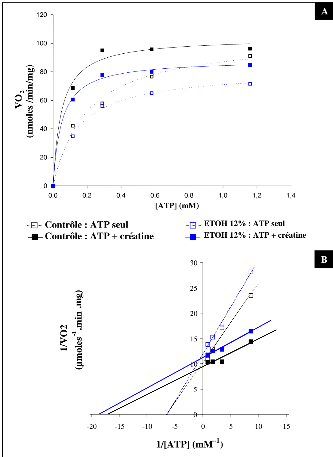
Figure 37 : Effet de l'ATP sur la respiration mitochondriale en présence ou en absence de créatine.
