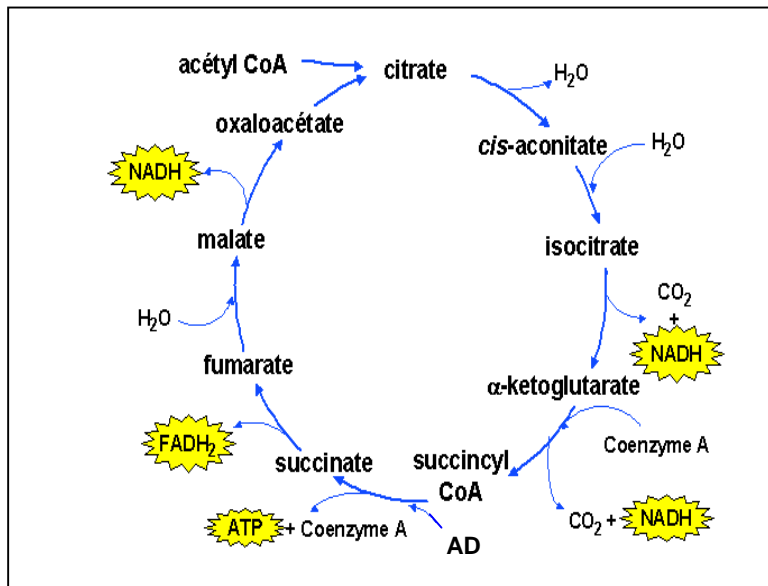
Figure 7 : Cycle de l'acide citrique.
