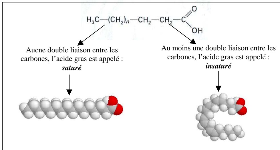
Figure 4 : Structures des acides gras saturés et des acides gras insaturés.
