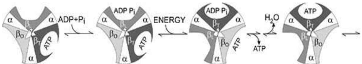
Figure 12 : Schéma du mécanisme de liaison-échange (Boyer 1993).
