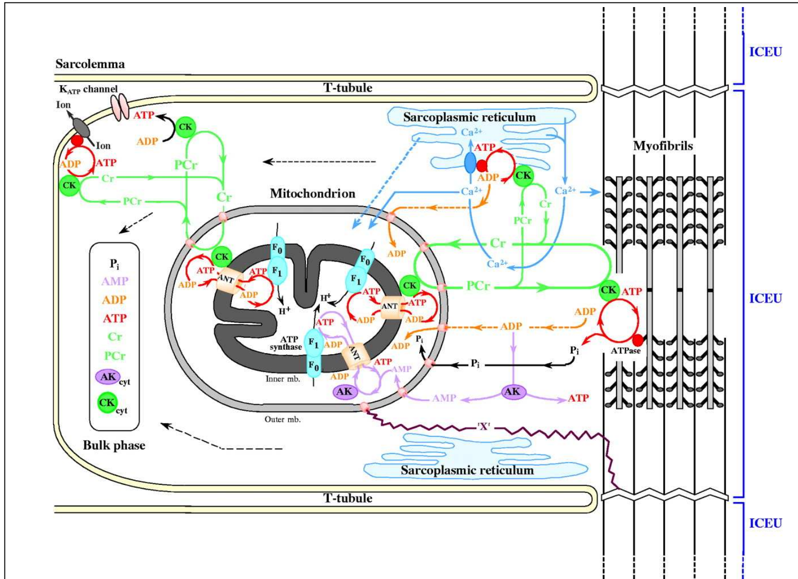
Figure 13: Organisation schématique de l'unité énergétique intracellulaire (ICEU) (Saks et al., 2001).
