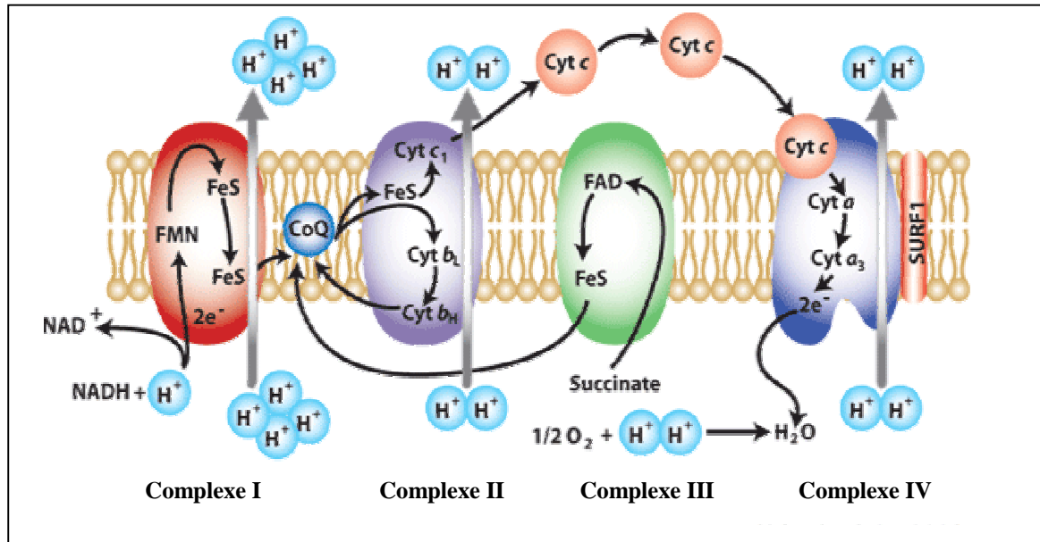
Figure 10 : Schéma de la chaîne respiratoire mitochondriale.
