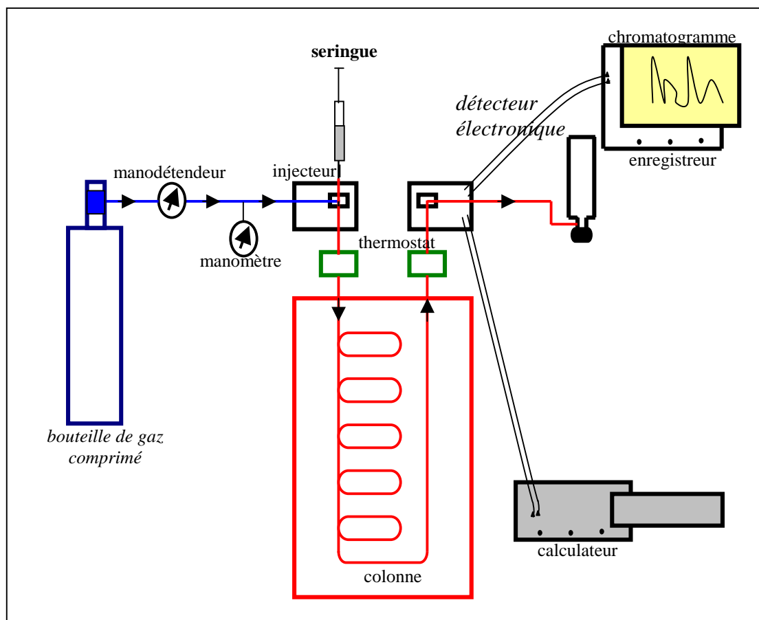
Figure 23: Représentation schématique d'un chromatographe en phase gazeuse.
