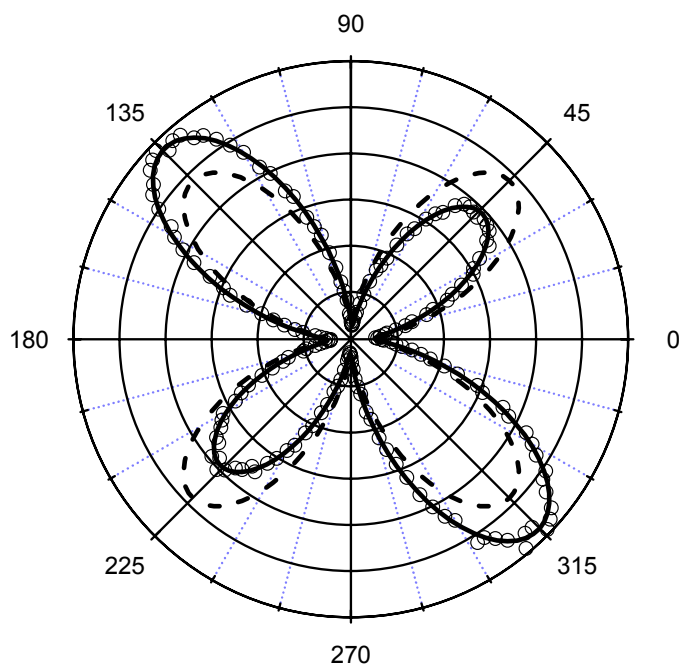
Figure 26 : Graphe polaire de l'intensité HRS polarisée verticalement en fonction de l'angle de la polarisation du champ incident ( 0^\circ =verticale) d'une solution de MT04+SDS dans un mélange eau/méthanol 5:1 (v/v). L'ajustement en trait pointillé est effectué par la relation (5.3). L'ajustement en trait plein est effectué par la relation (5.6). Cette mesure correspond au point [SDS]=0.48 mM de la Figure 22.
