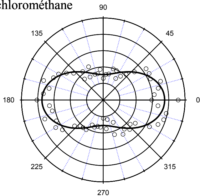
Figure 8 : Graphe polaire de l'intensité HRS du dichlorméthane polarisée verticalement en fonction de l'angle de polarisation du champ incident.
