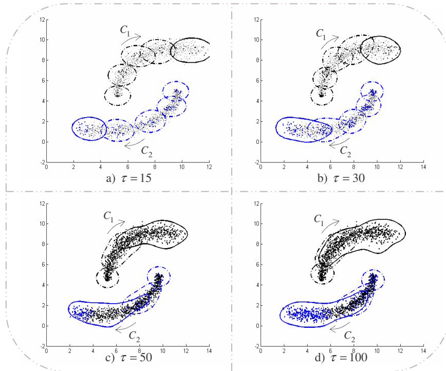
Figure 5.2.7 : Influence de \tau sur le modèle de classification du SAKM. Paramètres fixés : \lambda = 0,8 ; \nu = 0,3 ; \eta = 0,1 ; N_{\min} = 10 ; N_{\text{amb}} = 10 ; T = 333 .
