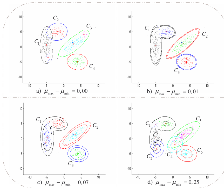
Figure 5.2.2 : Influence de \mu_{\min} et \mu_{\max} sur le modèle de classification de l'AUDyC : variation de \mu_{\max} - \mu_{\min} . Paramètres fixés : \sigma_{ini} = 0,8 ; \mu_{\min} = 0,02 ; N_p = \infty ; N_{\min} = 10 ; N_{amb} = 10 ; T = 333 .
