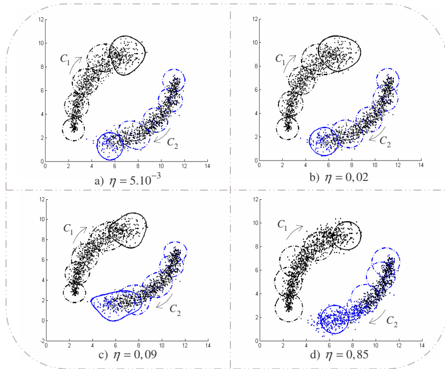
Figure 5.2.6 : Influence de \eta sur le modèle de classification du SAKM. Paramètres fixés : \lambda = 0,8 , \nu = 0,3 , \tau = 30 , N_{\min} = 10 , N_{amb} = 10 , T = 333 .
