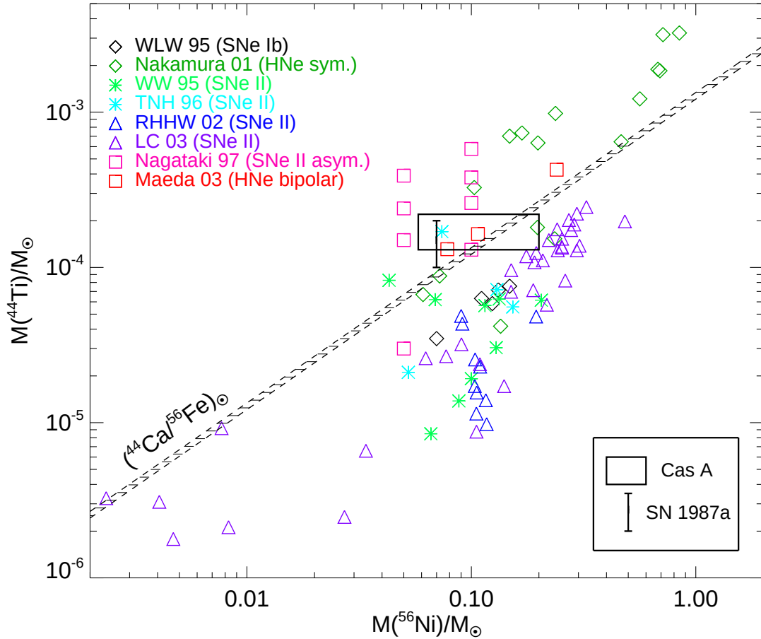
Figure 3.13 Diagramme Masse de ^{44}\text{Ti} - Masse de ^{56}\text{Ni} éjectées. Le rapport d'abondance ( ^{44}\text{Ca}/^{56}\text{Fe} ) solaire est indiqué par la zone hachurée (Anders et Grevesse 1989 ; Lodders 2003). Les différents points correspondent aux prédictions théoriques dans les supernovae gravitationnelles. Celles du modèle d'explosion bipolaire de Maeda et Nomoto (2003) pour expliquer les spectres et courbes de lumière des hypernovae observées, ainsi que celles calculées par Nagataki et al. (1998) ont été rajoutées.
