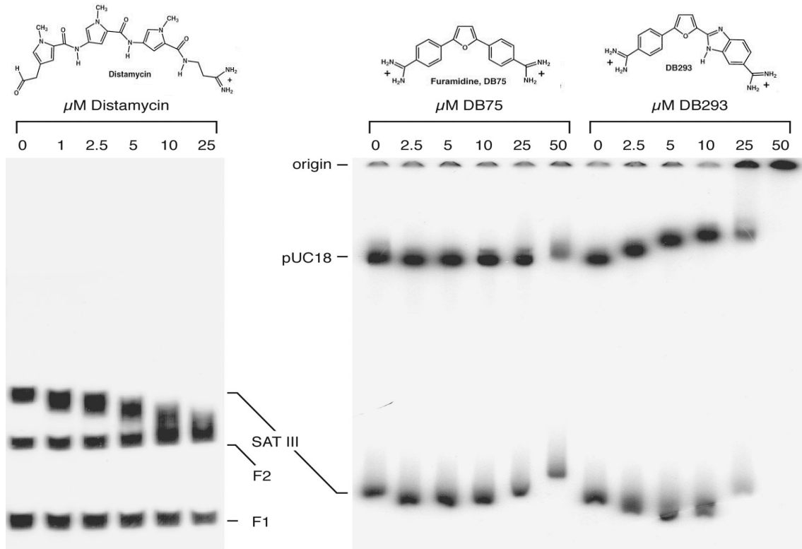
Figure 30 : Changement conformationnel d'un monomère SATIII induit par des ligands du petit sillon
