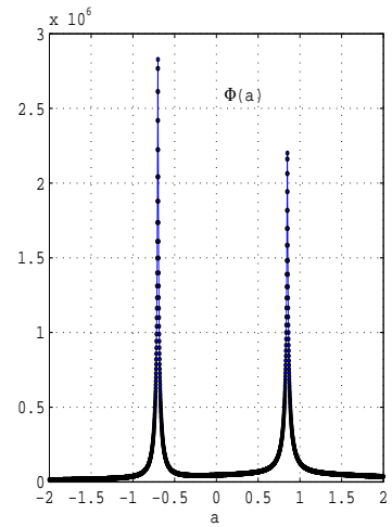
Fig. 1.17: Fonction coût
