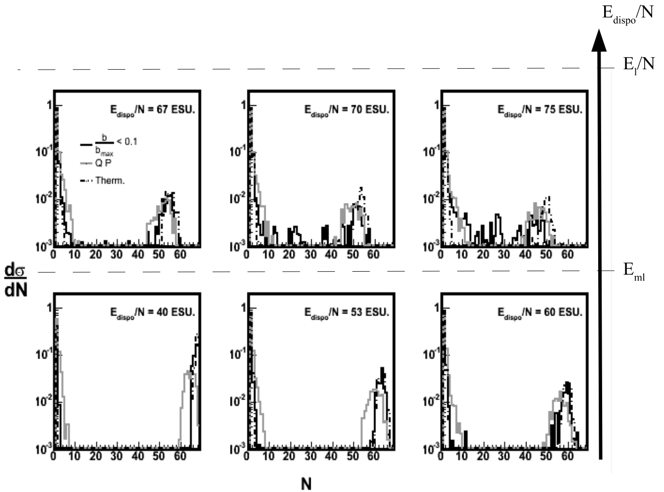
FIG. 3.9 – Distributions des tailles des fragments du système N = 68 pour les collisions centrales ( \frac{b}{b_{\text{max}}} \leq 0.1 ), pour les collisions périphériques (QP) et pour les systèmes préalablement thermalisés (Therm.). La densité de thermalisation est égale à \rho_0 . L'énergie incidente pour les collisions périphériques est égale à 120 ESU..
