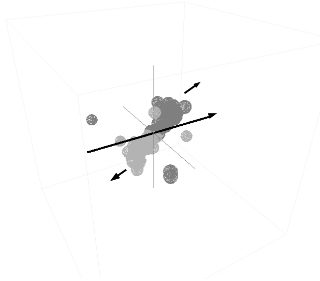
FIG. 5.11 – Cinématique d'une collision entre un projectile de ^{40}_{18}\text{Ar} (en foncé) sur une cible de ^{40}_{18}\text{Ar} (en clair) conduisant à la formation d'un col entre le quasi-projectile et la quasi-cible. L'axe de la collision est en trait plus épais.
