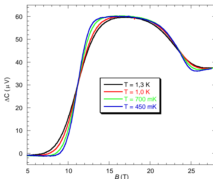
Figure VII.16 : Evolution selon la température des courbes de torque (orientation n°1, \theta = 135^\circ ).
