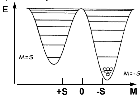
Figure IV.25 : Schéma de la population des niveaux d'énergie sous un champ magnétique important pour \text{Mn}_{12}\text{-Ac} .
