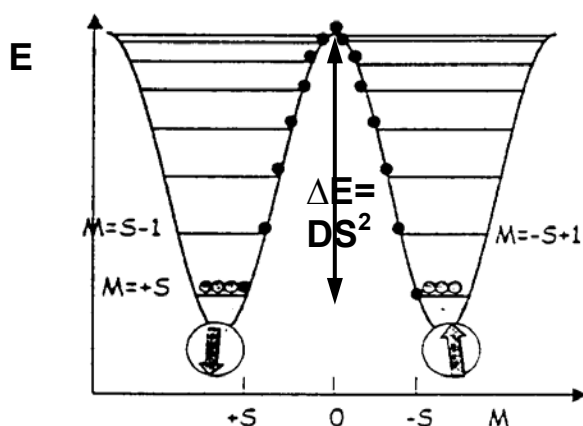
Figure IV.24 : Schéma de la levée de dégénérescence en champ nul de l'état fondamental S = 10 pour \text{Mn}_{12}\text{-ac} .
