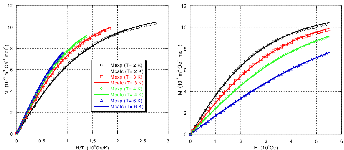
Figure VI.39 : Courbes de M = f(H/T) (à gauche) et M = f(H) (à droite) pour le complexe [Ni(imdipa)(NO 3 )] [NO 3 ]. Les cercles, carrés, triangles et losanges correspondent aux points expérimentaux, les traits pleins correspondent à l'ajustement de la loi théorique.
