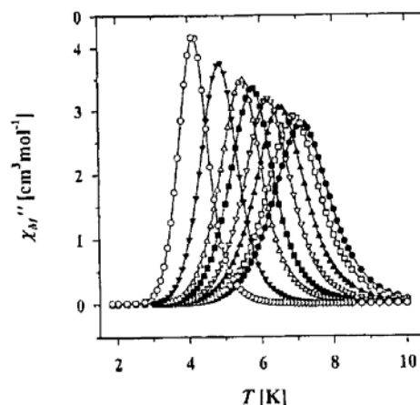
Figure IV.22 : Exemple de signal en quadrature de phase pour le composé [\text{Mn}_{12}\text{O}_{12}(\text{NO}_3)_4(\text{O}_2\text{CCH}_2\text{Bu}^\dagger)_{12}(\text{H}_2\text{O})_4] à 1(○), 10(▼), 50(△), 100(■), 250(▽), 500(▲), 1000(□) et 1500(●) Hz.
