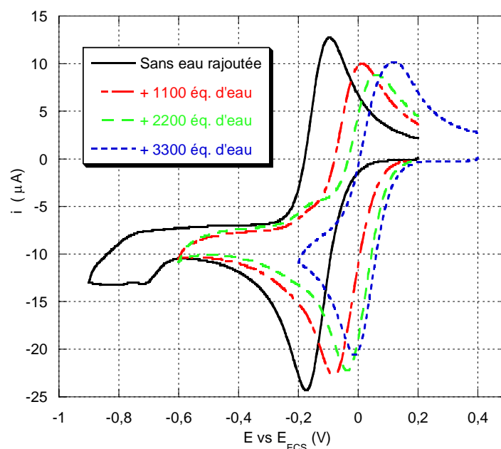
Figure II.15 : Cyclovoltammogrammes en réduction pour le complexe [\text{Fe}(\text{bispyphen})\text{Cl}]^+ , avec ajouts successifs d'eau ( 100 \mu\text{L} = 1110 \text{ équivalents} ) ( \text{CH}_3\text{CN} , c = 1 \times 10^{-3} \text{ mol L}^{-1} , [\text{N}(\text{Et})_4][\text{ClO}_4] 0,1 \text{ mol L}^{-1} , T = 20^\circ\text{C} , 100 \text{ mV s}^{-1} ). Les cyclovoltammogrammes sont corrigés de la dilution induite par l'ajout d'eau.
