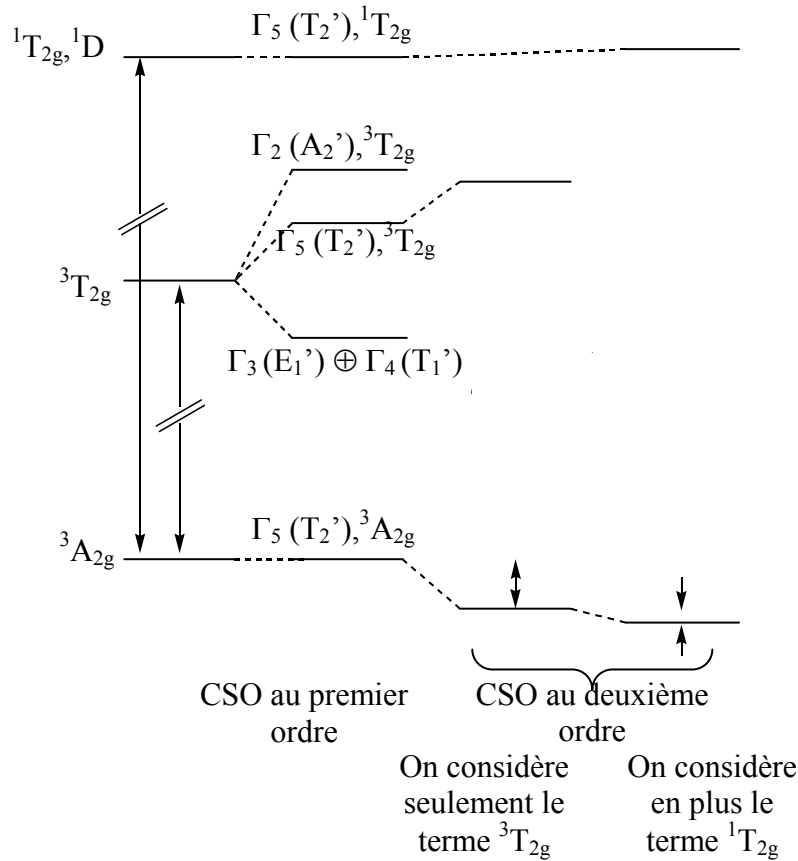
Figure V.5 : Schéma de l'action du couplage spin-orbite sur le terme fondamental ^3A_{2g} d'un ion Ni(II) en symétrie octaédrique.
