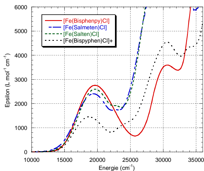
Figure II.7 : Spectres UV-Vis. des complexes mononucléaires dans l'acétonitrile ( c \approx 3 \times 10^{-4}\text{ mol L}^{-1} ).
