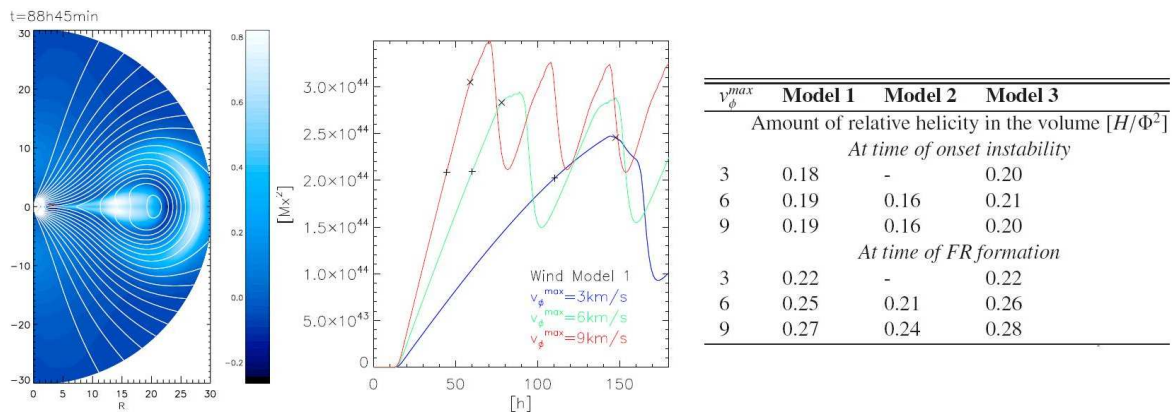
FIG. 4.12 – Simulation 2,5D de déclenchement d'une CME par cisaillement photosphérique dans la direction toroïdale (Jacobs et al. 2006). Gauche: distribution de la densité de plasma et lignes du champ magnétique. Centre: évolution de l'hélicité totale pour différentes vitesses de cisaillement. Les (+) indiquent l'instant du déclenchement de l'instabilité et les (X) le départ de la CME. Droite: valeur de la quantité totale d'hélicité pour différents modèles de vent solaire et différentes vitesses de cisaillement.
