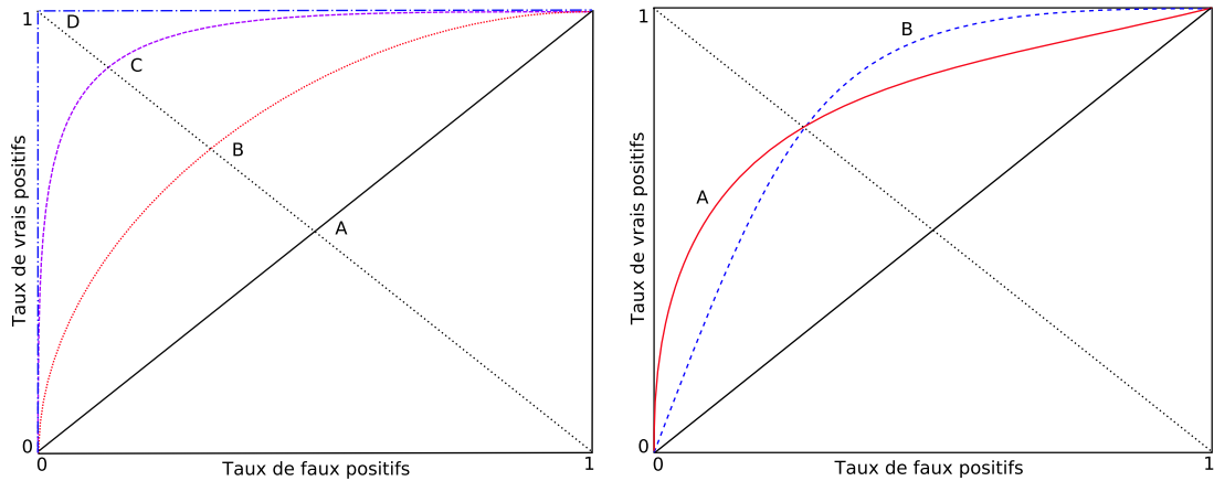
FIG. A.2 – Courbes ROC : à gauche, les courbes A, B, C et D sont respectivement associées à des classifieurs de performances croissantes. À droite, les courbes A et B ont la même aire (AUC) et la même valeur EER et sont pourtant associées à des classifieurs qui n'ont pas les mêmes qualités.
