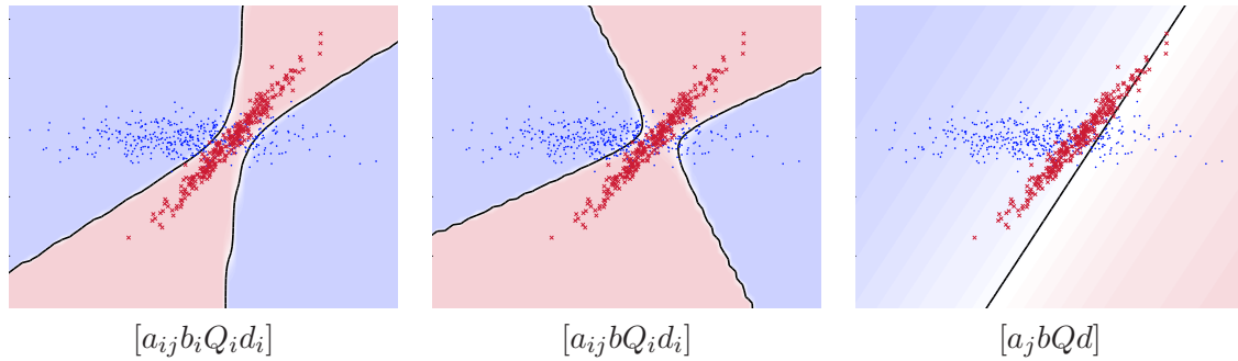
FIG. 5.2 – Frontières de décision de l’HDDA avec les modèles [a_{ij}b_i Q_i d_i] , [a_{ij}b Q_i d_i] et [a_j b Q d] sur les données simulées. Les données sont projetées sur deux des axes originaux pour la représentation uniquement.
