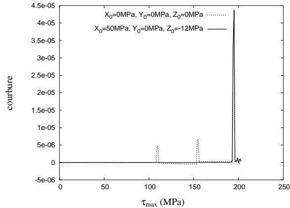
Figure II.28 - Courbure de l'évolution de \gamma_{\max}^f en fonction de \tau_{\max} pour \sigma = 225\text{MPa} et X_0 = 50\text{MPa} , Y_0 = 0\text{MPa} , Z_0 = -12\text{MPa}
