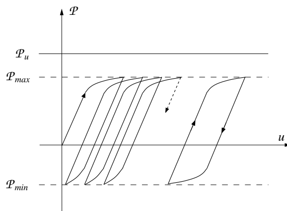
Figure I.5 - Plasticité alternée : ruine par fatigue oligocyclique
