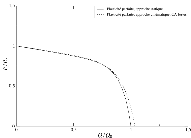
Figure IV.8 - Comparaison des approches statique et cinématique avec conditions d'admissibilité sous forme forte
