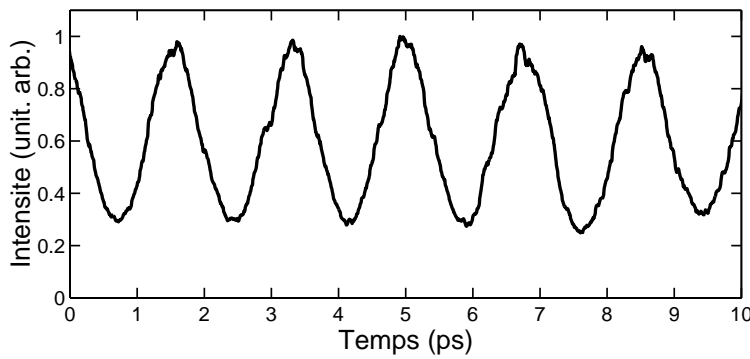
FIG. 3.34 - Fonction d'autocorrélation expérimentale pour la composante circulaire droite. P = 120 W sur chaque composante et \Omega = 0.6 THz .
