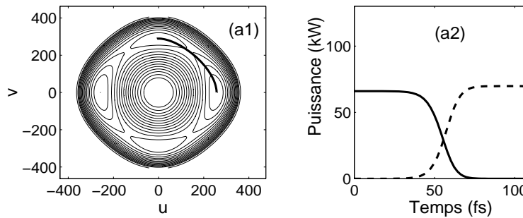
FIG. 4.5 - Parois de domaines dans le cas \rho = 0.18 . (a1) : trajectoire dans le potentiel, (a2) : profil d'intensité temporel.
