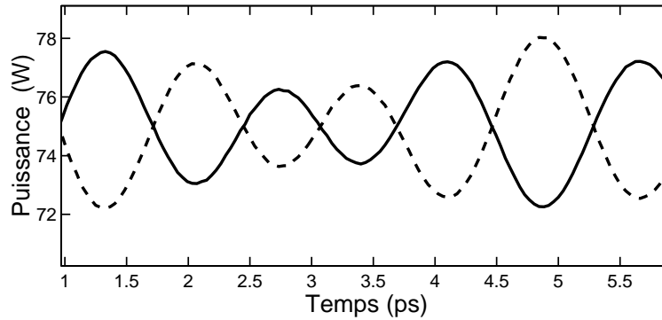
FIG. 2.13 - Intensités du mode LP_{01} (trait continu) et du mode LP_{11} (trait pointillé) pour \lambda = 626.5 \text{ nm} et pour P=Q=75 \text{ W} .
