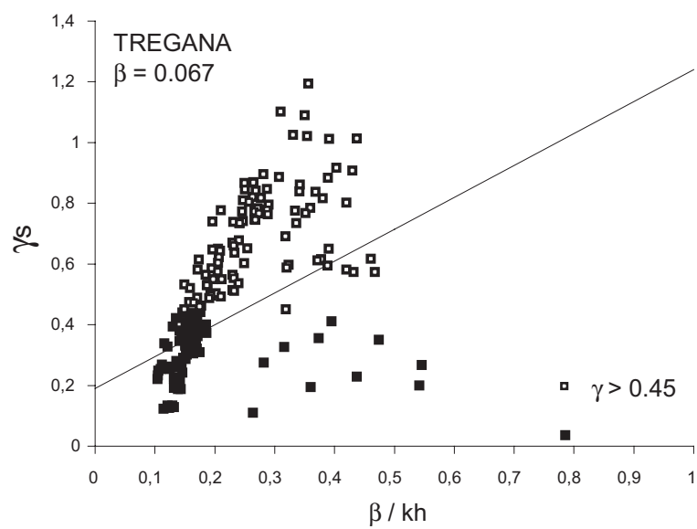
Illustration 120. Hauteur significative relative des vagues \gamma_s fonction de la pente locale normalisée \beta/kh pour les plages de Porsmilin, Corсен et Tregana. Toutes les données acquises sont représentées, les symboles blancs correspondent aux données en zone de surf.
