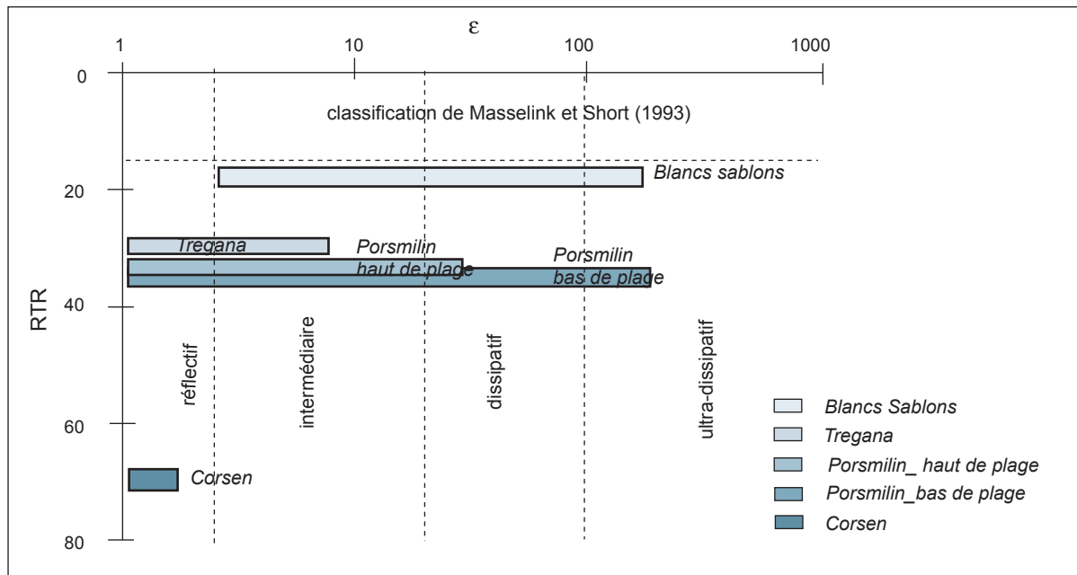
Illustration 79. Gamme des valeurs des indices RTR et \epsilon sur les plages macrotidales de la mer d'Iroise
