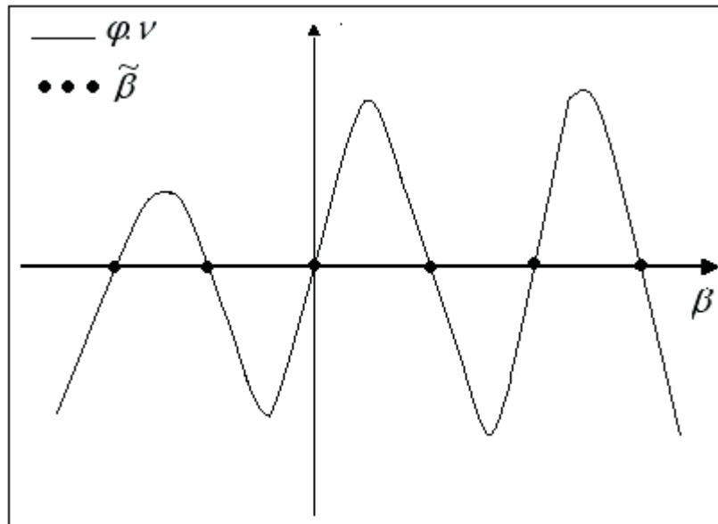
FIG. 5.2 – Cas de conditions de Neumann
