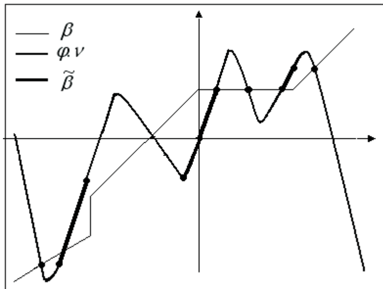
FIG. 5.3 – Cas de conditions plus générales
