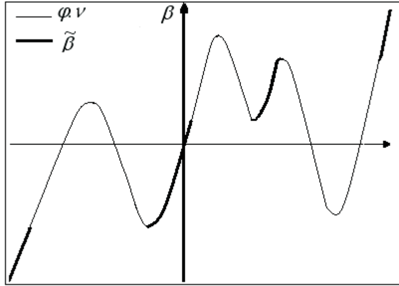
FIG. 5.1 – Cas de conditions de Dirichlet
