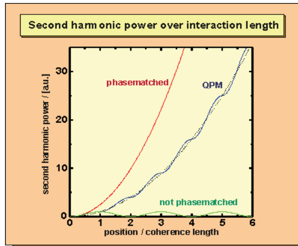
Fig.43. Dans un matériau avec accord de phase parfait, l'intensité du SH généré varie quadratiquement avec l'épaisseur du matériau non-linéaire traversé (courbe rouge). S'il n'y a pas d'accord de phase, l'intensité du faisceau doublé varie avec une période caractéristique (la longueur de cohérence), les minima correspondent aux franges d'interférence destructives entre les ondes engendrées en différents points du milieu traversé (courbe verte). Dans le cas de quasi-accord de phase (courbe bleue), la structure spécifique du matériau remet les ondes en phase, ce qui résulte en une efficacité élevée de génération de SH [109].
