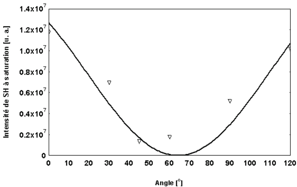
Fig.171. Intensité du signal de second harmonique généré (en unités arbitraires) à saturation, dans un film mince polymère constitué de P3BT + DR1-MMA 35/65 (dissous dans du C_6H_5Cl (25 mg/25 mg/1 ml)), en fonction de la différence de phase \Delta\Phi entre les faisceaux
