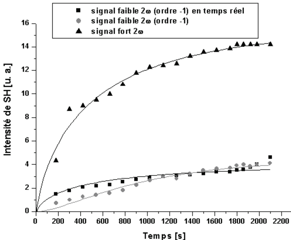
Fig.51. Ajustement théorique des mesures de dynamique pour une irradiation de l'échantillon de DR1-MMA 35/65 (470 nm épais) pendant 35 minutes. Les mesures des dynamiques des deux ordres ont été d'abord effectuées de manière classique : les triangles et cercles sont les mesures effectuées pour l'ordre (0) et (-1), respectivement ; les carrés représentent les valeurs obtenues en temps réel pour l'ordre (-1). Les courbes en continu correspondent à un ajustement théorique des données expérimentales.
