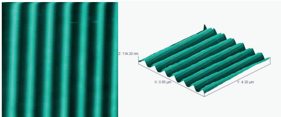
Fig.136. A gauche, image obtenue par microscopie à force atomique (AFM) d'un réseau de surface inscrit grâce au système interférentiel à deux voies. Le réseau est représentée en niveaux de bleu-noir, codant les variations topographiques ( 3,85 \mu\text{m} \times 4,20 \mu\text{m} ). A droite, le même réseau en trois dimensions.
