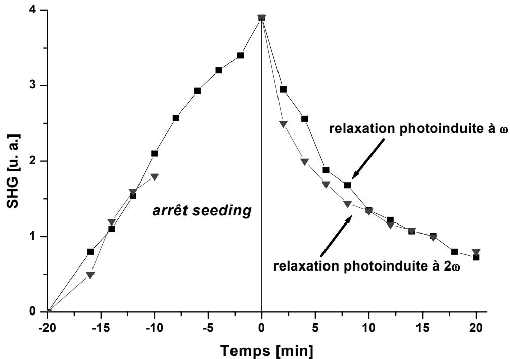
Fig.30. Relaxation photo-induite après orientation d'une couche mince de DR1-MMA 35/65, les carrés représentent la relaxation photo-induite à la fréquence fondamentale ( \omega ), les triangles, la relaxation photo-induite à la fréquence SH ( 2\omega ).
