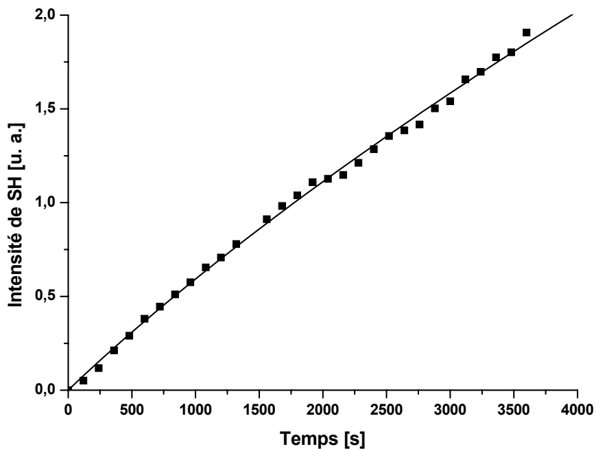
Fig.115. Dynamique de croissance du signal de SH généré dans le film de Z-183-PVK. La courbe en continu représente un ajustement monoexponentiel de la croissance du signal de deuxième harmonique généré, la saturation est atteinte à la valeur de 19,53546 ( b = 25621,378 s, c = 0,50976 ).
