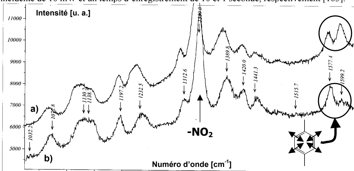
Fig.85. Spectres Raman de l'échantillon a) non-réticulé (courbe en haut) et b) réticulé et orienté par polarisation par effet Corona (courbe en bas).
