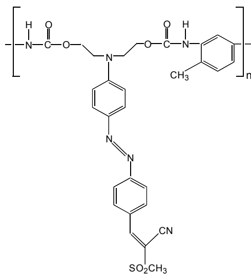
Fig.56. Représentation schématique du polymère polyuréthane greffé avec le ligand de l'azo-cyano-sulphométhyle (PU-CNMS).
