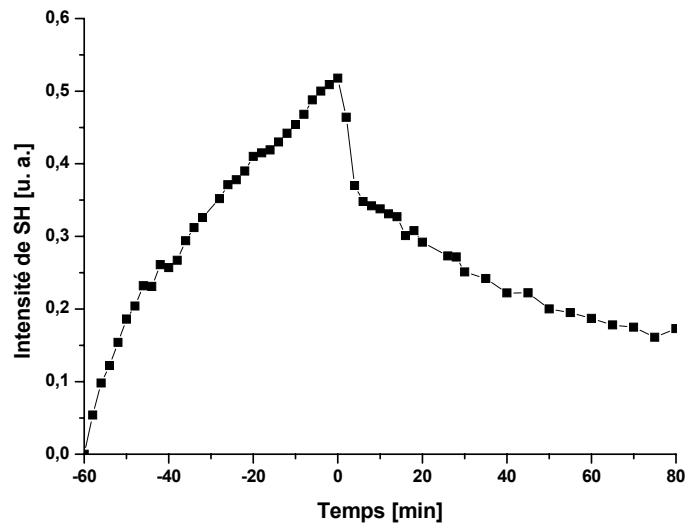
Fig.102. Amplitude du signal de deuxième harmonique généré par l'échantillon constitué de IP-1077A-PVK, en unités arbitraires, en fonction du temps. Les temps positifs correspondent à l'étude de la dépolarisation d'orientation induite auparavant, par irradiation à la fréquence fondamentale.
