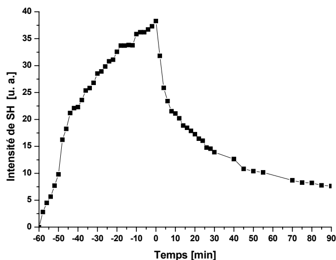
Fig.106. Dynamique de montée et de décroissance temporelle (à l'extinction de l'harmonique d'écriture) du signal de second harmonique généré par l'échantillon de PMMA dopé avec IP-1077B.
