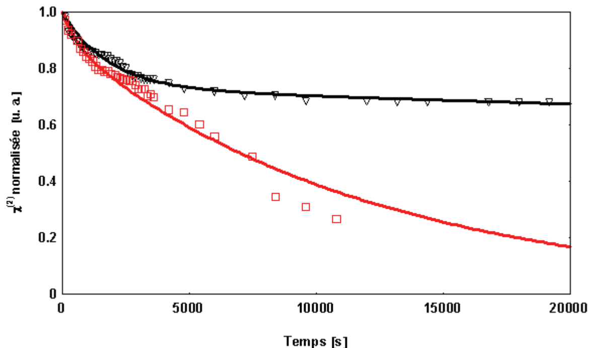
Fig.82. Dynamique de décroissance de \chi^{(2)} normalisée dans l'échantillon non-réticulé. Les triangles correspondent à la décroissance de \chi^{(2)} , sous illumination constante avec le faisceau fondamental. Les carrés correspondent à la décroissance de \chi^{(2)} , sous illumination constante avec le faisceau de second harmonique (le faisceau SH de la lecture a été coupé lors de la mesure de chaque point). Les courbes en continu sont les ajustements théoriques, à l'équation (69), des points expérimentaux.
