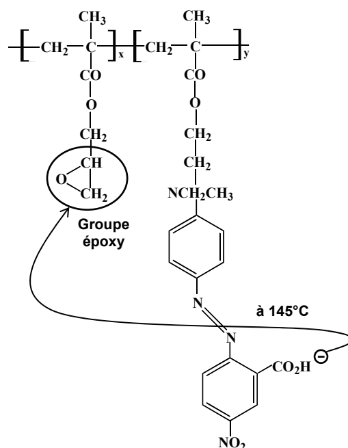
Fig.75. Structure chimique du polymère thermoréticulable ; x = \frac{2}{3} , y = \frac{1}{3} .
