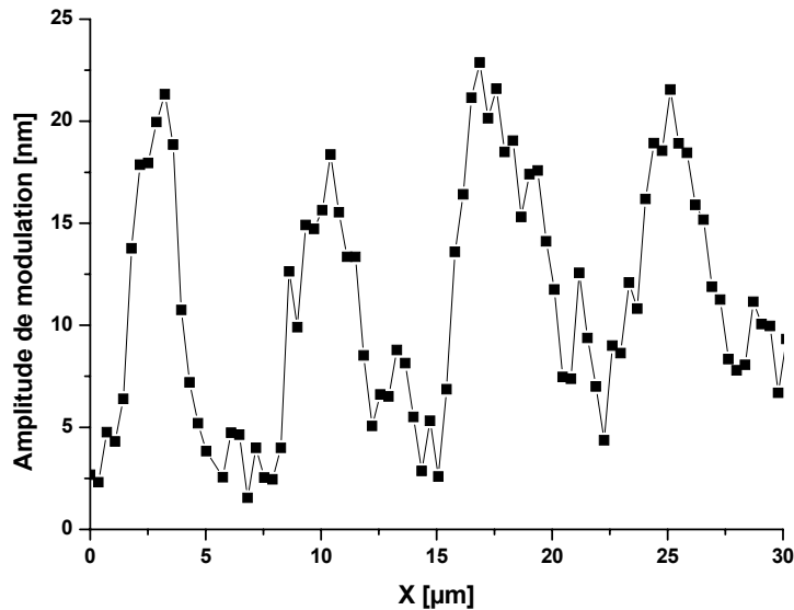
Fig.147. Profil d'un réseau de surface présente en fig.146, enregistré sur un film de DR1-MMA 35/65 de 190 nm d'épaisseur, dans une configuration p-p de polarisations des faisceaux d'écriture à \omega et 2\omega , après 16 heures d'irradiation ( I_{2\omega} = 3,956 \text{ mW/cm}^2 , I_{\omega} = 2,873 \text{ W/cm}^2 ).
