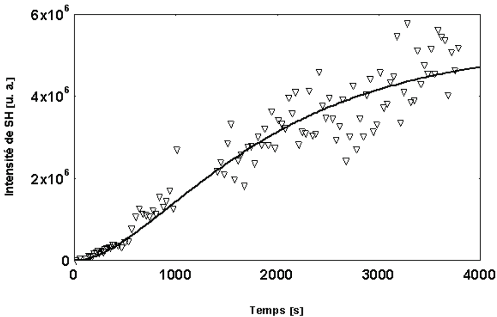
Fig.169. Croissance temporelle de l'intensité de second harmonique généré, en unités arbitraires, \Delta\Phi = 90^\circ . La courbe en continu est l'ajustement à l'équation y = a \times [1 - \exp(-x/b)]^2 . La saturation du signal est atteinte à 5,2347 \times 10^6 [u. a.], b = 1344,2 s.
