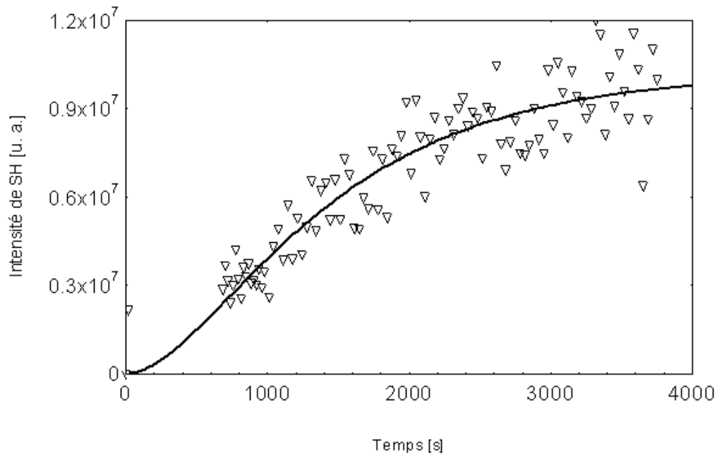
Fig.170. Croissance temporelle de l'intensité de second harmonique généré, en unités arbitraires, \Delta\Phi = 120^\circ . La courbe en continu est l'ajustement à l'équation y = a \times [1 - \exp(-x/b)]^2 . La saturation du signal est atteinte à 1,0205 \times 10^7 [u. a.], b = 1035 s.
