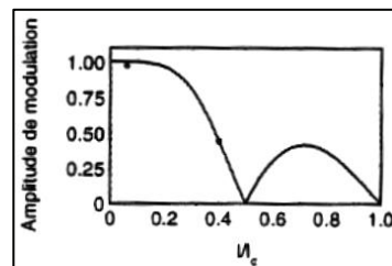
Fig.34. Amplitude de modulation en fonction du rapport de l'épaisseur de l'échantillon sur la longueur de cohérence [70].
