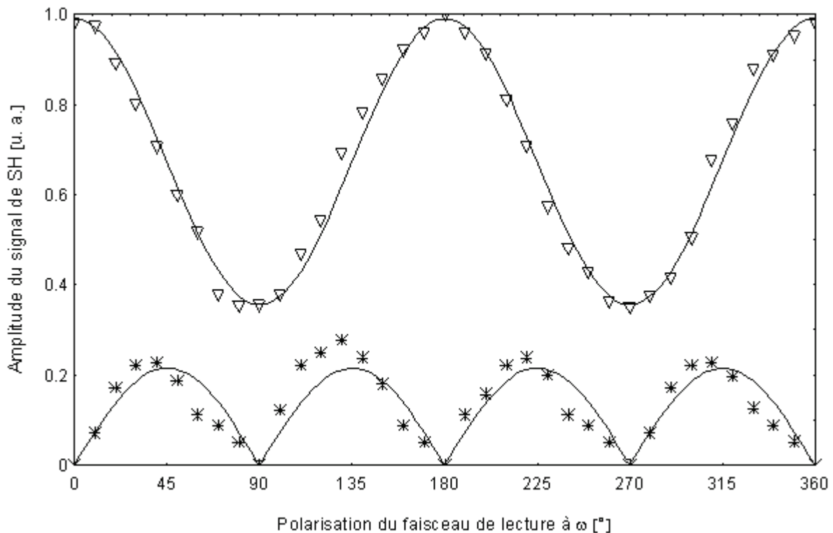
Fig.55. Amplitude du signal de SH (définie comme la racine carrée de l'intensité du signal de SH) en fonction de l'angle \theta de polarisation du faisceau de lecture. Les triangles correspondent au signal généré dans la direction parallèle à la direction de polarisation des faisceaux d'écriture (direction y , polariseur P_1 ) ; les étoiles correspondent au signal généré dans la direction perpendiculaire (direction x , polariseur P_2 ). L'échantillon est un copolymère de DR1-MMA 35/65 d'épaisseur 250 nm, placé sur un prisme et polarisé dans les conditions optimales. Les courbes continues correspondent aux ajustements théoriques obtenus à partir des équations (46-a) et (46-b).
