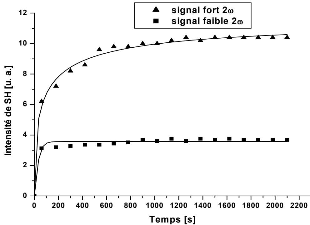
Fig.62. Seeding de l'échantillon de PU-CNMS. Les triangles indiquent l'évolution temporelle du signal vert "fort", les carrés, celle du signal vert "faible" (ordre -1, dynamique testée de façon classique). Les courbes continues sont les ajustements à l'équation y = a \times \left[ 1 - \exp\left(-\frac{x}{b}\right)^c \right]^2 . Les faisceaux d'écriture ont été fortement focalisés sur l'échantillon.
