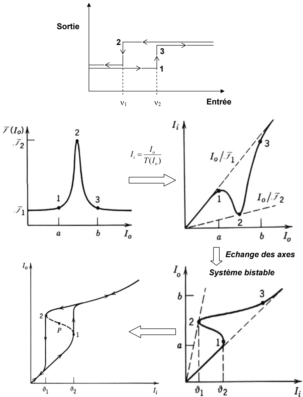
Fig.110. Cycle d'hystérésis donnant le champ transmis en fonction du champ incident, observé en faisant varier l'intensité I_i de la lumière incidente.
