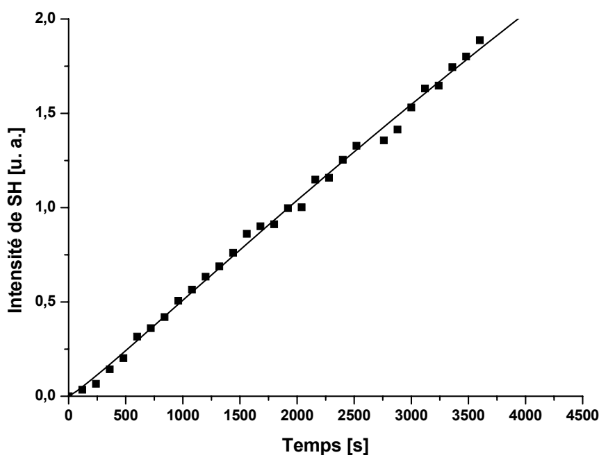
Fig.113. Dynamique de croissance du SH généré dans le film de Z-181 avec du PVK. La courbe en continu représente un ajustement monoexponentiel de la croissance du signal de deuxième harmonique généré, la saturation est atteinte à la valeur de 16,80348 ( b = 17331,78263 s, c = 0,57995 ).
