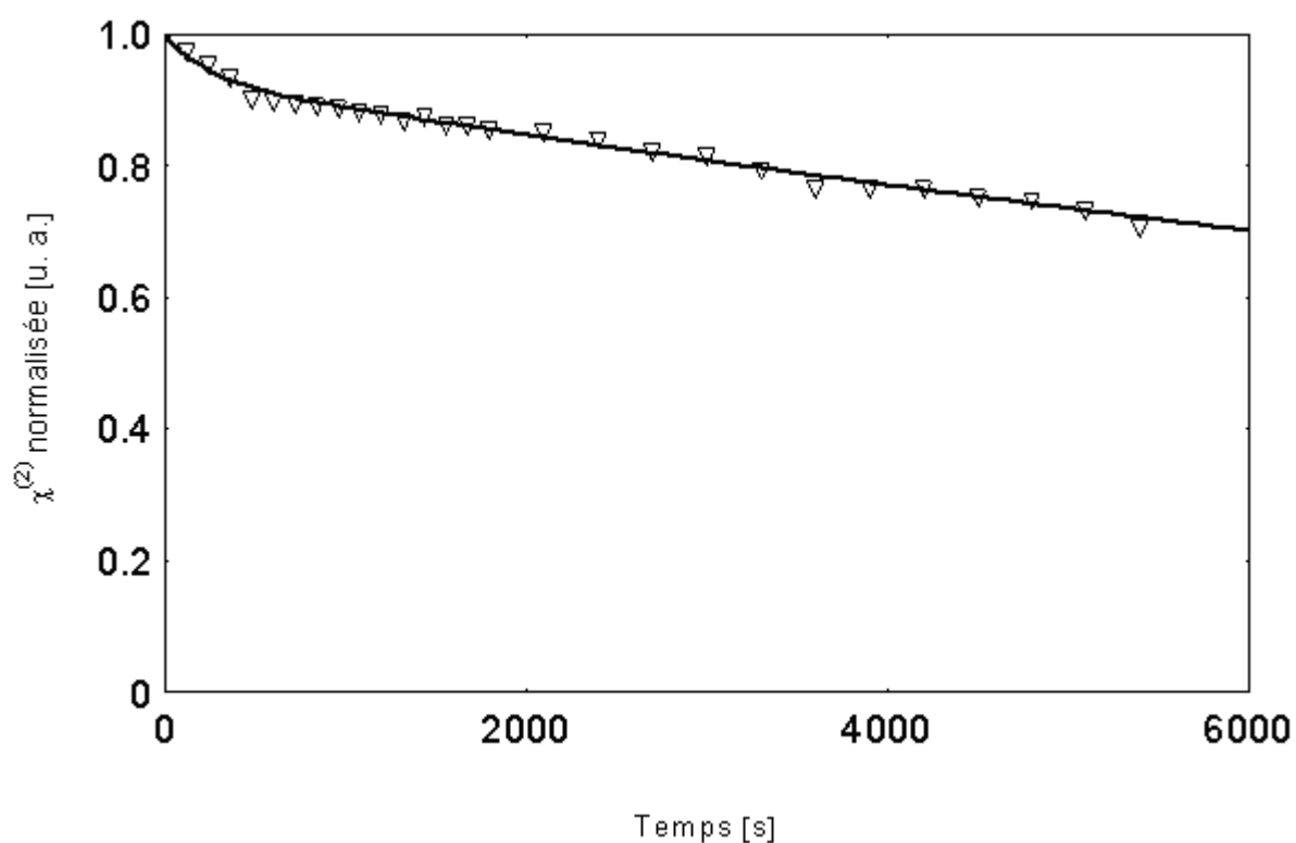
Fig.123. Décroissance de \chi^{(2)} normalisée, dans le film de Z-182-PVK. La courbe en continu est l'ajustement théorique à l'équation (69), des points expérimentaux.
