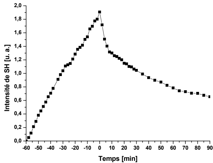
Fig.100. Dynamique temporelle du signal de deuxième harmonique observé dans le cas d'une couche mince de Z-183-PVK. Au temps zéro, la phase d'écriture a été arrêtée.
