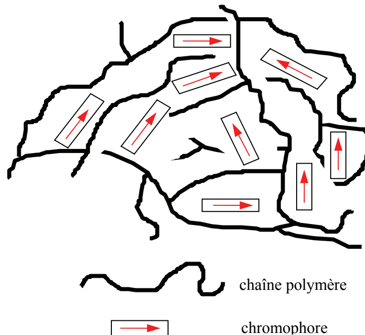
Fig.6. Structure d'un polymère dopé. Les flèches représentent les moments dipolaires des molécules du colorant.
