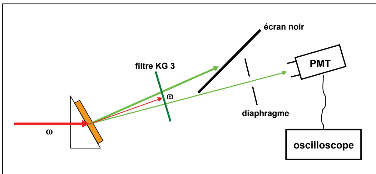
Fig.48. Montage expérimental afin de mesurer la dynamique de la génération du SH en temps réel.
