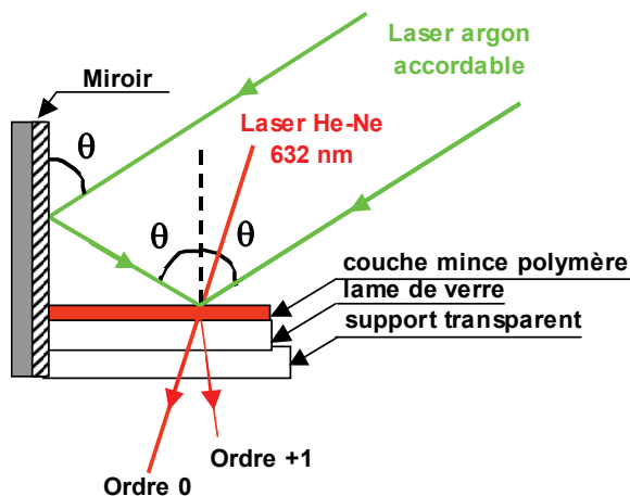
Fig.134. Dispositif d'inscription des réseaux de surface du type miroir de Lloyd. Le laser incident est un laser Ar + accordable (la longueur d'onde utilisée est placée entre 488 et 514 nm), les puissances appliquées varient de 50 à 300 mW/cm 2 .
