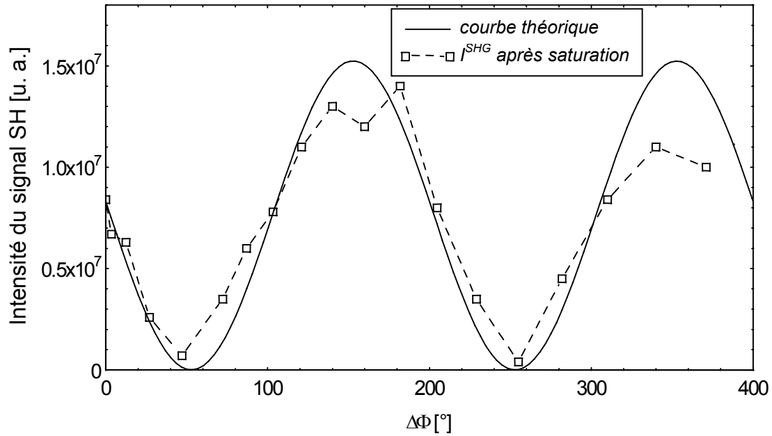
Fig.33. Dépendance de l'intensité du signal de second harmonique généré (en unités arbitraires) en fonction de la différence de phase relative \Delta\Phi entre les faisceaux d'écriture dans le cas d'un échantillon non placé sur un prisme [70]. La référence \Delta\Phi = 0 est fixée arbitrairement.
