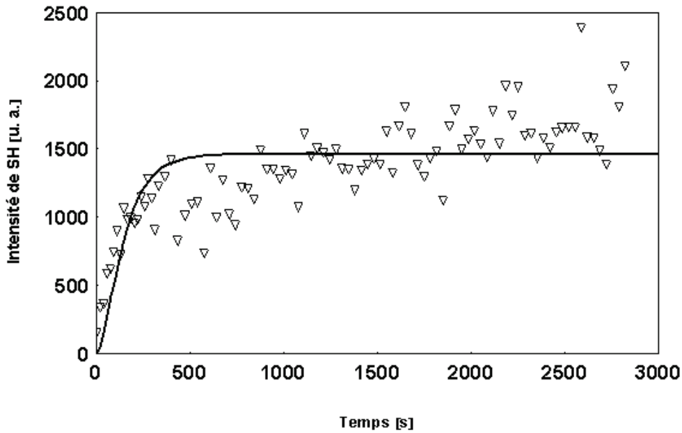
Fig.160. Croissance temporelle de la génération de second harmonique, en unités arbitraires, \Delta\Phi = 0^\circ . La courbe en continu est l'ajustement à l'équation y = a \times [1 - \exp(-x/b)]^2 . La saturation du signal est atteinte à 1461,76 [u. a.], b = 104,979 s.
