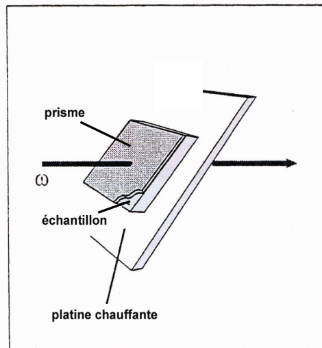
Fig.87. Dispositif d'étude d'orientation tout-optique thermo-assistée in situ . L'échantillon est placé sur un prisme, la platine chauffante est adjacente au film polymère.
