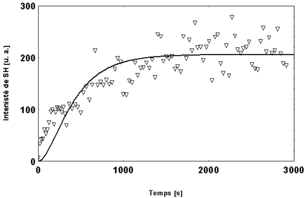
Fig.162. Croissance temporelle de la génération de second harmonique, en unités arbitraires, \Delta\Phi = 120^\circ . La courbe en continu est l'ajustement à l'équation y = a \times \left[1 - \exp\left(-\frac{x}{b}\right)\right]^2 . La saturation du signal est atteinte à 205,76 [u. a.], b = 298,9 s.
