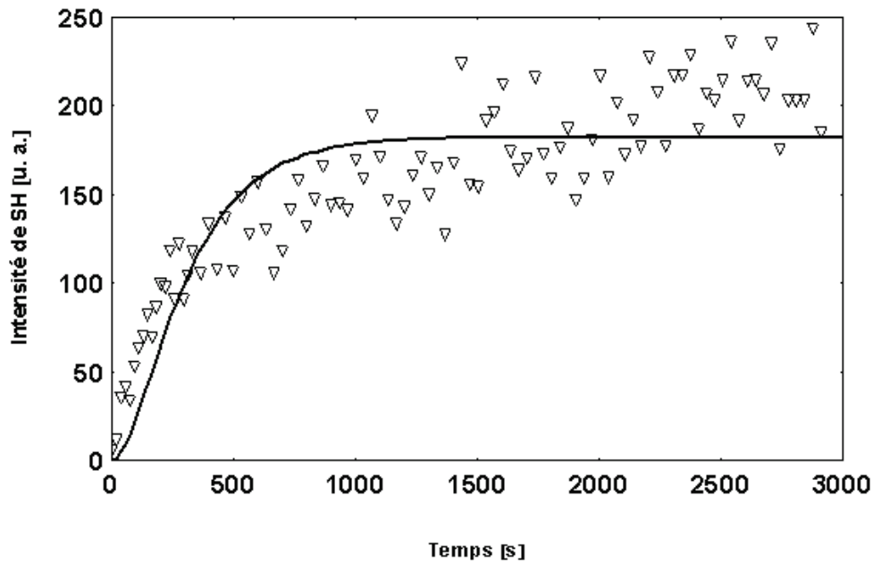
Fig.161. Croissance temporelle de la génération de second harmonique, en unités arbitraires, \Delta\Phi = 90^\circ . La courbe en continu est l'ajustement à l'équation y = a \times [1 - \exp(-x/b)]^2 . La saturation du signal est atteinte à 182,309 [u. a.], b = 220,606 s.
