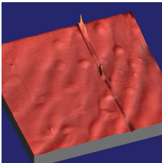
Fig.142. Image AFM d'un réseau de surface induit sur un film mince de DR1-MMA 35/65 (270 nm épais) à l'aide de faisceaux d'écriture polarisés en configuration p-p (28 heures d'irradiation). La rayure traversant la photo provient d'un artefact provenant de l'AFM. Notons également la faible modulation de surface de ce réseau (25 nm) par rapport à l'épaisseur initiale du film. Les intensités des faisceaux d'écriture étaient égales à I_{2\omega} = 1,7 \text{ mW/cm}^2 , I_{\omega} = 2,8 \text{ W/cm}^2 .
