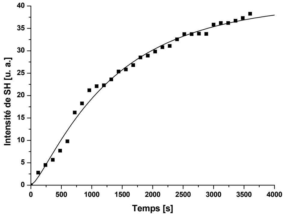
Fig.120. Dynamique de la croissance de l'intensité de second harmonique généré dans la couche composée de la molécule IP-1077B avec du PMMA. La courbe continue représente un ajustement monoexponentiel de la croissance du signal de deuxième harmonique généré ; la saturation est atteinte à la valeur de 41,01421 ( b = 820,91606 s, c = 0,74926 ).
