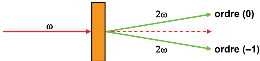
Fig.47. Phase de lecture réalisée de façon classique avec un faisceau fondamental en incidence normale sur un échantillon polarisé, dans une configuration avec un prisme.
