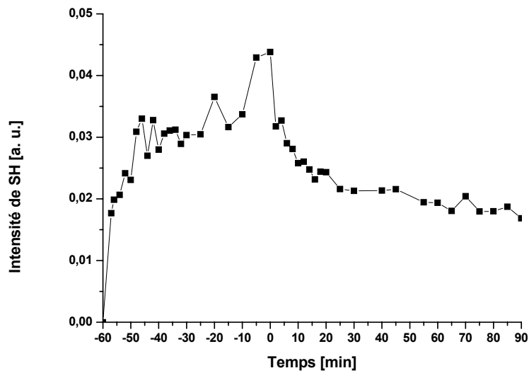
Fig.101. Etude de construction et stabilité temporelle du signal de SH photoinduit dans une couche de PVK dopée avec la molécule de Z-184-PVK. Les temps négatifs correspondent à la polarisation du matériau. Au temps zéro la phase d'écriture a été arrêtée.
