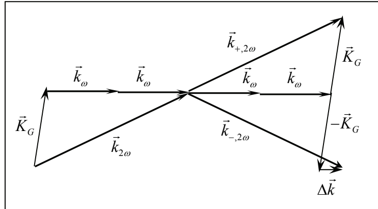
Fig.46. Schéma des vecteurs d'onde des ondes interagissant lors du processus de polarisation tout-optique dans une configuration avec un prisme. \vec{K}_G = \vec{k}_{2\omega} - 2\vec{k}_\omega est le vecteur d'onde du réseau, \vec{k}_\omega est le vecteur d'onde à la fréquence fondamentale, \vec{k}_{+,2\omega} est le vecteur d'onde à la fréquence second harmonique du signal de forte intensité, \vec{k}_{-,2\omega} est le vecteur d'onde à la fréquence second harmonique du signal de faible intensité.
