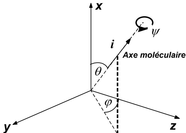
Fig.18. Représentation d'une molécule unidimensionnelle donnée dans un repère (x,y,z) . Les repères polaires sont données par les angles d'Euler (\theta, \varphi, \psi) .
