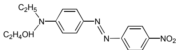
Fig.1. Disperse Red 1 (4-(N-2-hydroxyethyl)-N-ethyl)-amino-4'-nitroazobenzène), molécule unidimensionnelle de type "push-pull", \mu = 7,5 D [10], \Delta\mu = 17 D [11].
