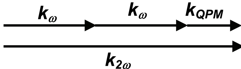
Fig.42. Schéma des vecteurs d'ondes impliqués lors de la conversion de fréquence dans un milieu avec quasi-accord de phase.
