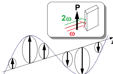
Fig.20. Représentation polaire des propriétés tensorielles de \chi^{(2)} photoinduites en fonction de des coordonnées de propagation selon l'axe z dans le cas de polarisations linéaires et parallèles des faisceaux d'écriture à \omega et 2\omega [56].
