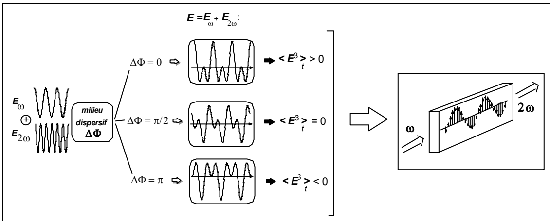
Fig.16. Allure de l'“interférence polaire” \langle E^3 \rangle_t résultant d'une superposition des champs aux fréquence fondamentale et second harmonique pour des phases relatives différentes. Il en résulte une modulation spatiale de la nonlinéarité quadratique au sein du matériau. Cette modulation possède une périodicité permettant un accord de phase nécessaire au doublement de fréquence.
