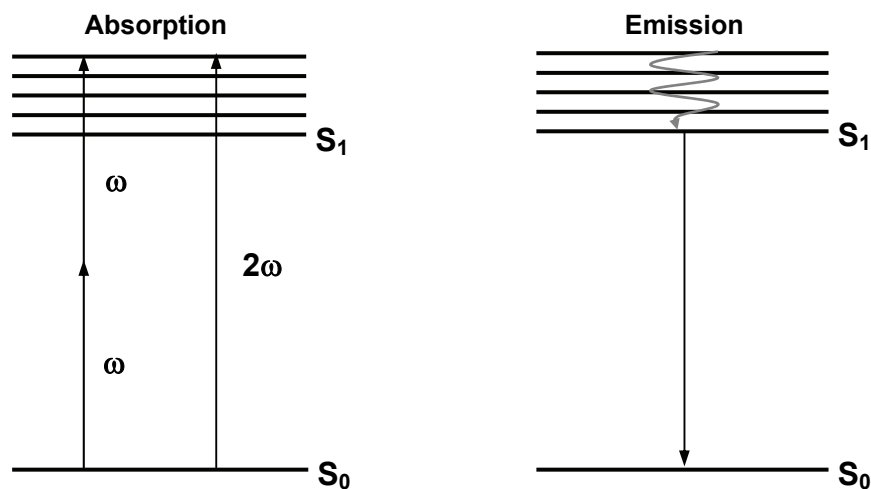
Fig.28. Schéma des niveaux énergétiques d'une molécule. L'excitation est provoquée par l'absorption d'un photon à la fréquence de second harmonique 2\omega ou de deux photons à la fréquence fondamentale \omega . Relaxation partielle avec perte de chaleur par échange avec le milieu ambiant, retour à l'état fondamental par émission lumineuse (fluorescence) en conséquence de la transition du niveau S_1 au niveau S_0 .
