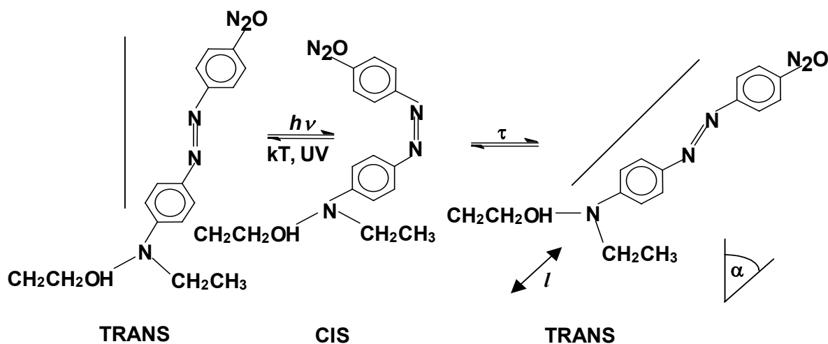
Fig.2. Illustration de la rotation axiale de la molécule via l'isomérisation trans-cis-trans de la molécule de Disperse Red 1 (symétrie C_{ov} ). A la suite de chaque cycle d'excitation-relaxation, la molécule tourne d'un certain angle \alpha , mais aussi parcourt une distance l . Le retour cis-trans est activé thermiquement.
