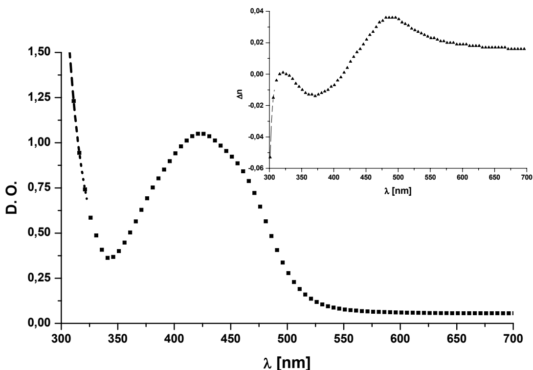
Fig.67. Spectre d'absorption du PMMA dopé avec la molécule bis-azoïque à 10 % en masse. La densité optique à 532 nm est égale à 0,098. Le pic d'absorption se trouve à 423 nm (1,511). La courbe reportée en insertion donne la variation de l'indice par rapport à sa valeur hors absorption, extrapolée à partir du spectre d'absorption par les formules de Kramers-Krönig.
