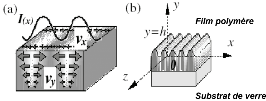
Fig.139. (a) Schéma du modèle de Fukuda et Sumaru [211]. La vitesse du transport de la matière dans les couches supérieures ( v_x ) suit les directions prévues par le modèle du gradient du champ [212]. La vitesse du transport de la matière dans les zones dans la profondeur, v_y , décroît quand on s'approche du substrat et elle est nulle au niveau du substrat ; (b) système des coordonnées utilisé [213].
