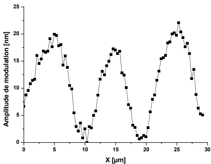
Fig.143. Profil de la section transverse d'un réseau inscrit après 28 heures d'irradiation, sur un film de DR1-MMA 35/65 d'épaisseur 270 nm (polarisation p-p ), présenté en fig.142.
