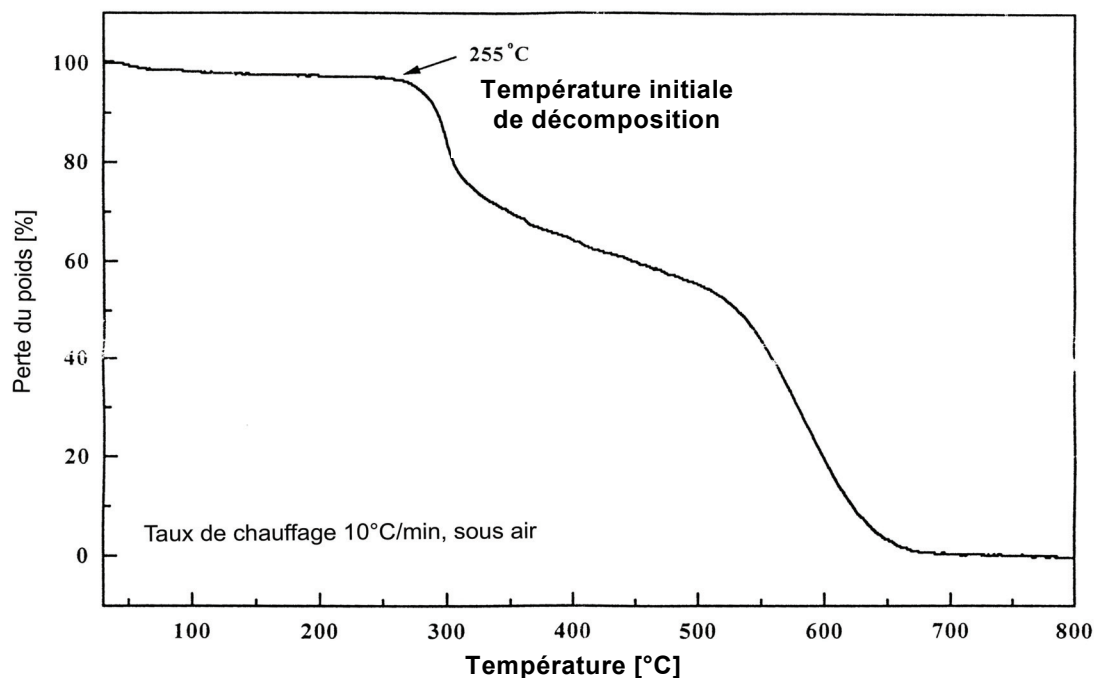
Fig.59. Etude de la stabilité thermique du polymère PU-CNMS. Le polymère commence à se décomposer à 255°C.
