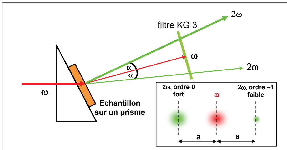
Fig.45. Configuration des faisceaux en sortie du prisme. Les tâches des faisceaux verts sont répartit symétriquement par rapport à la tâche du faisceau infrarouge.
