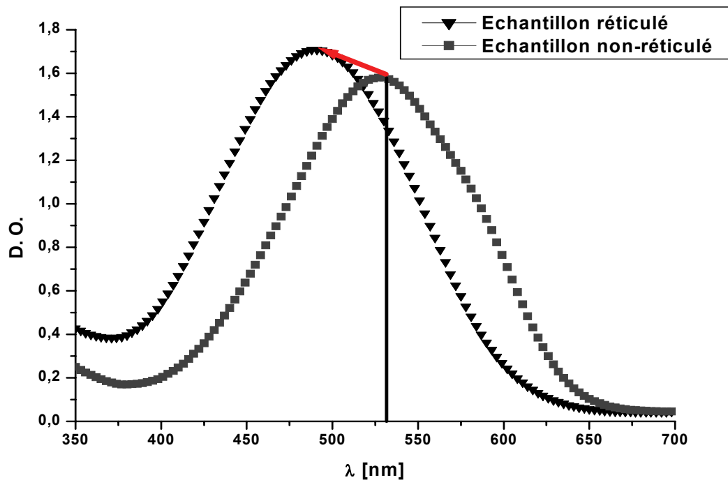
Fig.77. Spectres des échantillons non-réticulés (carrés) et réticulés (triangles). La ligne verticale indique la longueur d'onde de 532 nm. La densité optique du film non-réticulé et réticulé est respectivement égale à 1,57 et 1,35. Le blueshift est de 37 nm.
