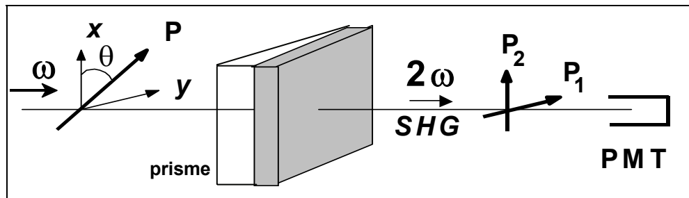
Fig.54. Etude du signal de SH généré dans la direction parallèle ( y ) et perpendiculaire ( x ) à la direction de polarisation des faisceaux d'écriture (selon l'axe y ). L'échantillon est placé sur un prisme.
