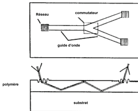
Fig.141. Couplage et découplage d'une onde guidée dans un film par un réseau de surface [208].
