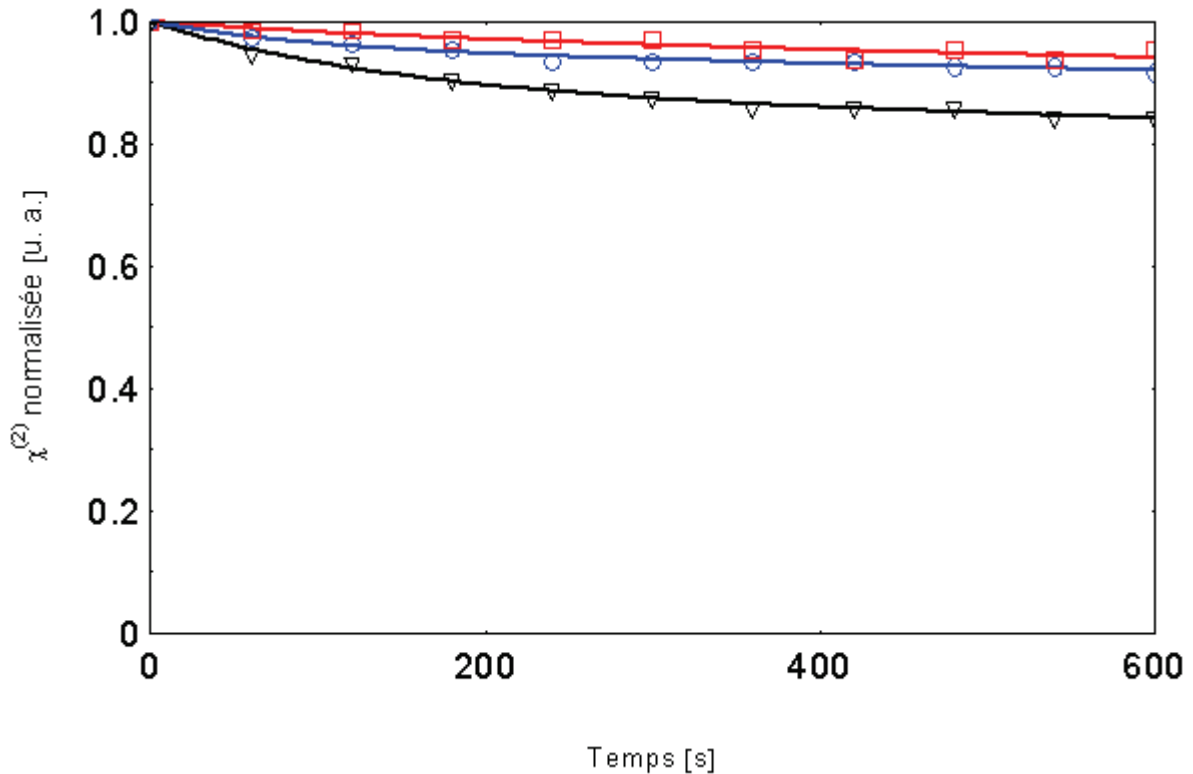
Fig.70. Relaxation in-situ par génération de second harmonique dans un film mince de Stimdiazol-PMMA dopé à 12 % en masse (les triangles et carrés, représentent, respectivement, la décroissance du signal vert fort (ordre 0) et faible (ordre -1)) et de Stimdiazol-PMMA dopé à 10% en masse (les cercles sont les résultats obtenus pour le signal vert fort (ordre 0)). La valeur de \chi^{(2)} a été normalisée à sa valeur maximale. Les courbes continues sont les ajustements à l'équation (69).
