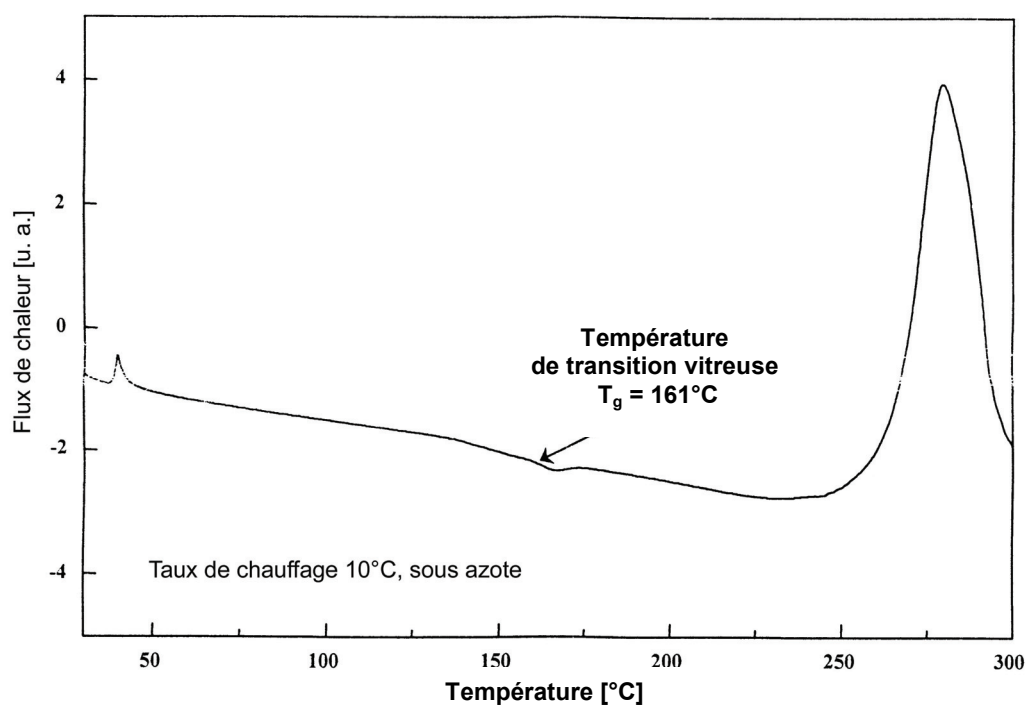
Fig.58. Thermogramme du polymère PU-CNMS. La température de transition vitreuse est égale à 161°C.
