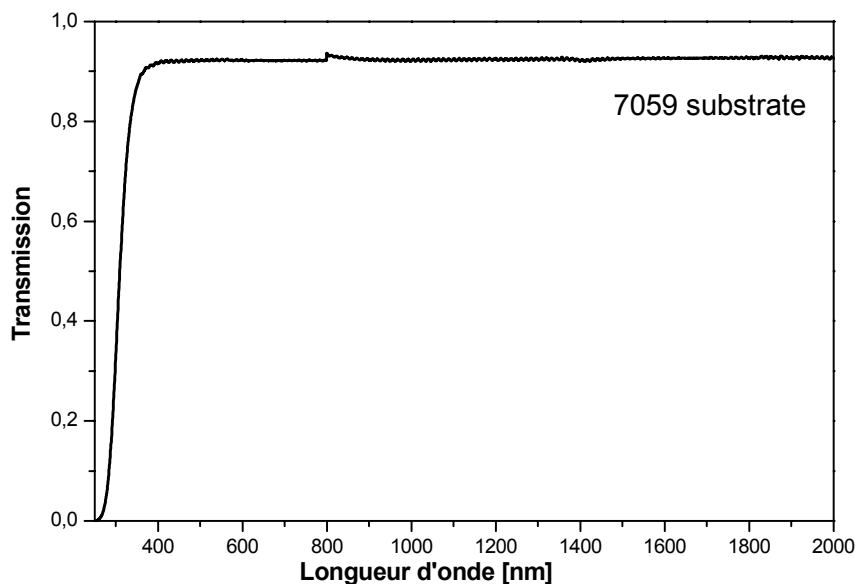
Fig.76. Spectre de transmission du substrat de verre Corning 7059.
