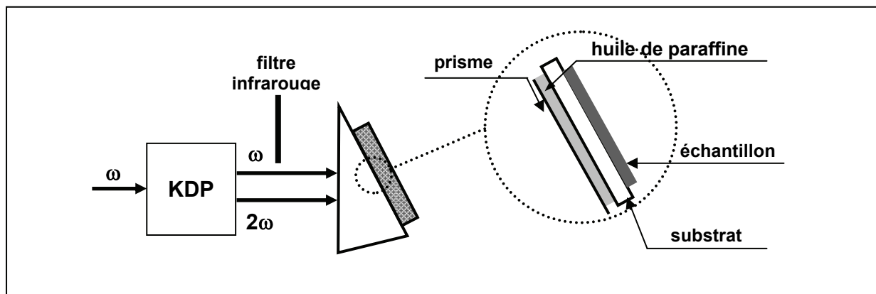
Fig.36. Nouvelle configuration du dispositif expérimental.
