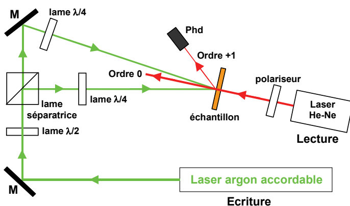
Fig.135. Montage interférentiel d'inscription à deux voies ; M – miroir, Phd – photodiode pour l'enregistrement de l'intensité de l'ordre +1 diffracté par le réseau.
