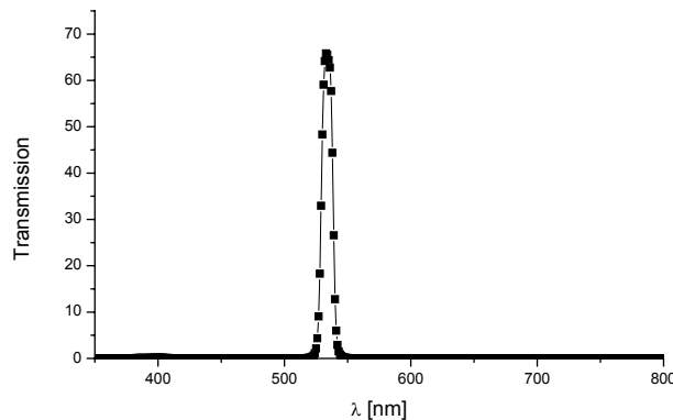
Fig.26. Spectre de transmission du filtre interférentiel utilisé. On sélectionne une bande étroite autour de la longueur d'onde 532 nm.
