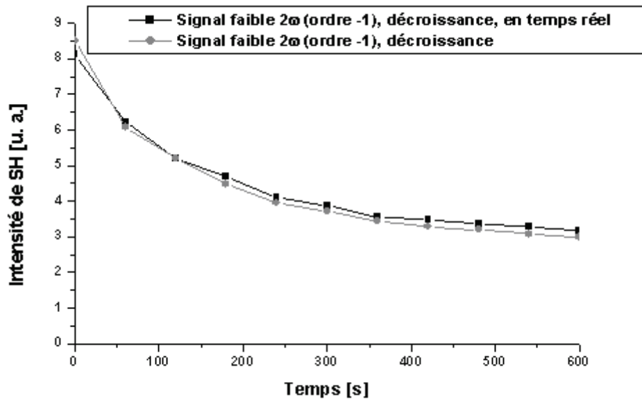
Fig.50. Dépolarisation de l'orientation induite par irradiation à la fréquence fondamentale, dans le cas du faisceau vert correspondant à l'ordre -1 , et dans le cas de croissance testée en temps réel et de croissance testée de manière classique (les périodes d'écriture et de lecture alternés). Les faisceaux ont été fortement focalisés sur l'échantillon placé sur le prisme. Au temps zéro la phase d'écriture a été arrêtée.
