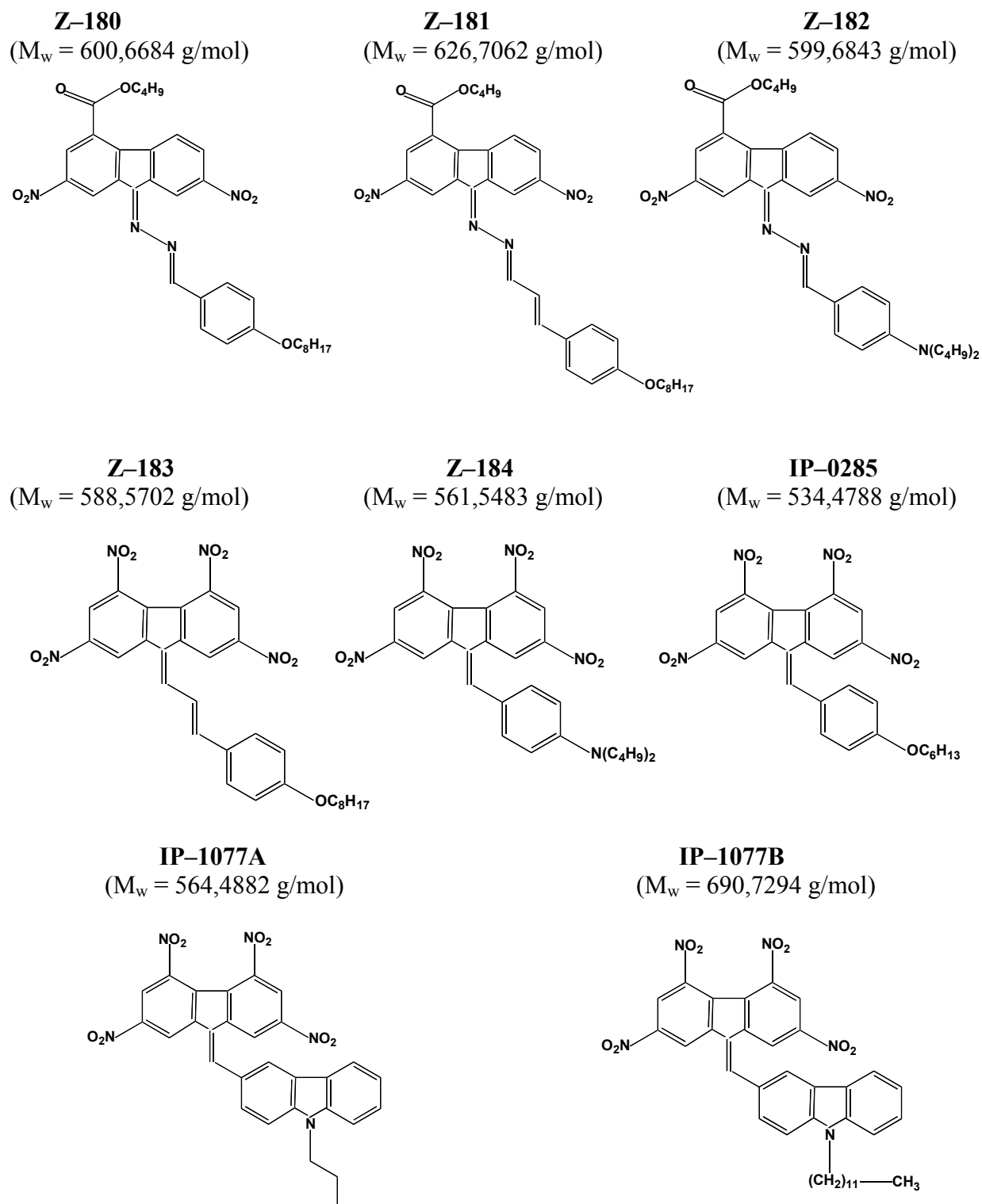
Fig.94. Structure chimique planaire des composés étudiés.
