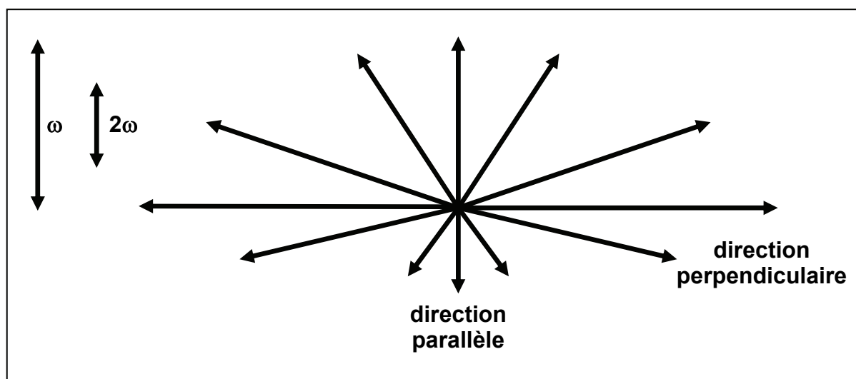
Fig.21. Distribution orientationnelle moléculaire après le processus de polarisation tout-optique. La différence dans le nombre des molécules orientées dans le sens positif et négatif est plus grande dans la direction parallèle à la polarisation des faisceaux d'écriture (on observe une noncentrosymétrie). Dans la direction perpendiculaire, le nombre des molécules alignées avec un sens positif et négatif reste le même (i.e. est centrosymétrique) [68].
