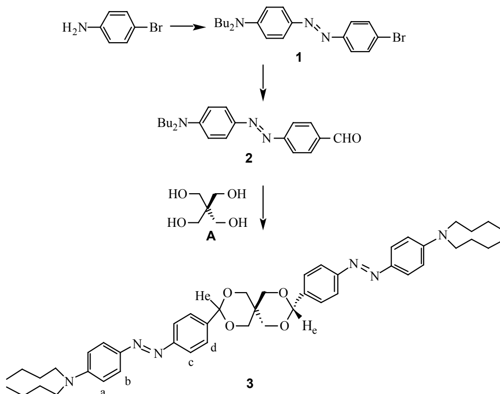
Fig.66. Réaction de condensation permettant la synthèse du composé étudié [137].
