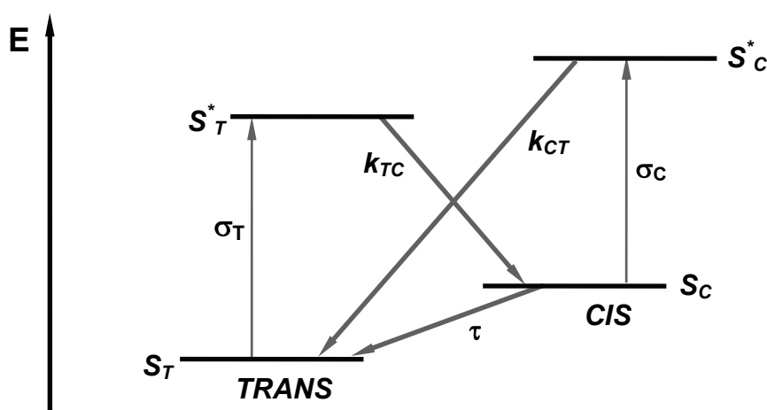
Fig.3. Diagramme d'énergie d'une molécule de type azobenzène (Disperse Red 1) impliquant les états trans et cis de la molécule ; S_T, S_C – les états fondamentaux, S_T^*, S_C^* – les états excités des isomères trans et cis , \sigma_T, \sigma_C – les section efficaces d'absorption des isomères trans et cis , k_{TC}, k_{CT} – les constantes de désexcitation, respectivement, de l'état trans à cis et de cis à trans , \tau – la constante de relaxation thermique cis-trans .
