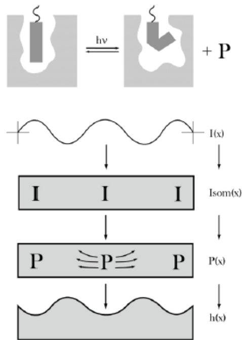
Fig.138. Représentation schématique du mécanisme de formation des réseaux de surface, impliquant les gradients de pression interne ; p est la pression, I représente l'intensité de la lumière, x est un point dans le matériau polymère [208].
