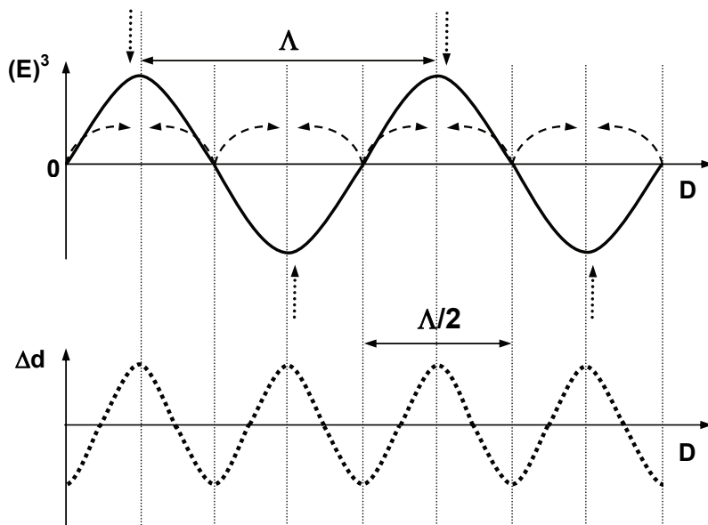
Fig.150. Formation d'un réseau de surface par le processus d'orientation tout-optique. La courbe en trait continu représente la modulation de la moyenne temporelle au cube \langle E^3 \rangle_t du champ E(t) = E_{\omega}(t) + E_{2\omega}(t) qui est une superposition cohérente de deux faisceaux aux fréquences fondamentale et second harmonique, avec une période \Lambda . Les flèches verticales en pointillé indiquent l'orientation antiparallèle ; ici pour une polarisation s-s des faisceaux d'écriture, que les molécules prennent dans le but de minimiser leur interaction avec le champ incident excitant. Les flèches courbées en pointillé indiquent la direction du transport de masse qui se produit lorsque la distribution orientationnelle moléculaire est stationnaire. La courbe en pointillée représente la modulation de surface de l'échantillon ( \Delta d ), avec une période \Lambda/2 , due au transport de matière photoinduit.
