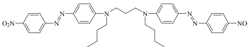
Fig.71. Structure moléculaire du composé bis-azoïque étudié. L'angle entre les deux branches contenant la liaison double azoïque possède une valeur moyenne d'environ 60^\circ (la molécule n'est pas linéaire) [140].
