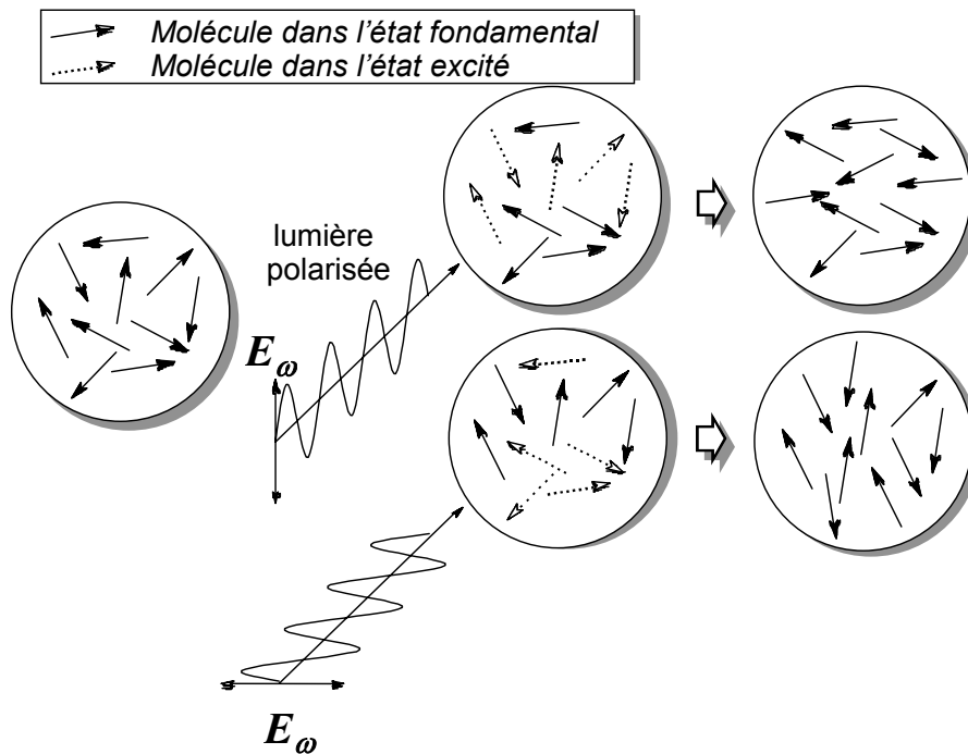
Fig.5. Induction optique d'anisotropie (biréfringence et dichroïsme).
