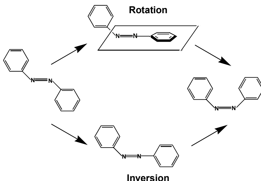
Fig.4. Mécanismes possibles de photoisomérisation : rotation et inversion.
