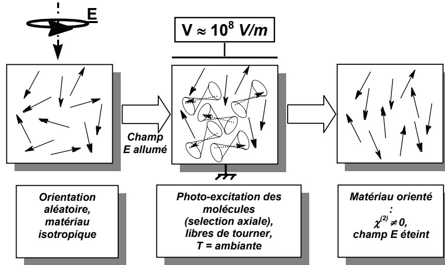
Fig.12. Procédure d'orientation par champ électrique photo-assistée. Les flèches représentent les moments dipolaires des molécules; les flèches en trait plein et pointillé représentent, respectivement, les états fondamentaux et excités de la molécule. La photo-excitation à l'aide d'une lumière polarisée circulairement permet la rotation des molécules, représentées comme des sabliers. Seules les molécules excitées tournent.
