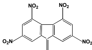
Fig.104. Le groupe accepteur de la molécule IP-1077A, de faible solubilité.
