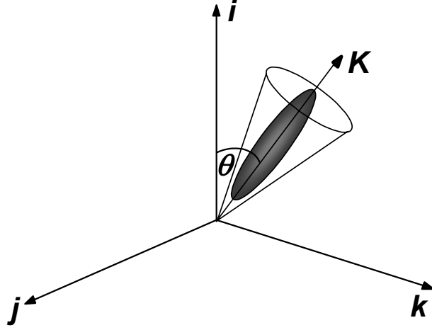
Fig.14. Représentation de l'axe d'une molécule de type bâtonnet (unidimensionnelle) dans le référentiel (i,j,k) .
