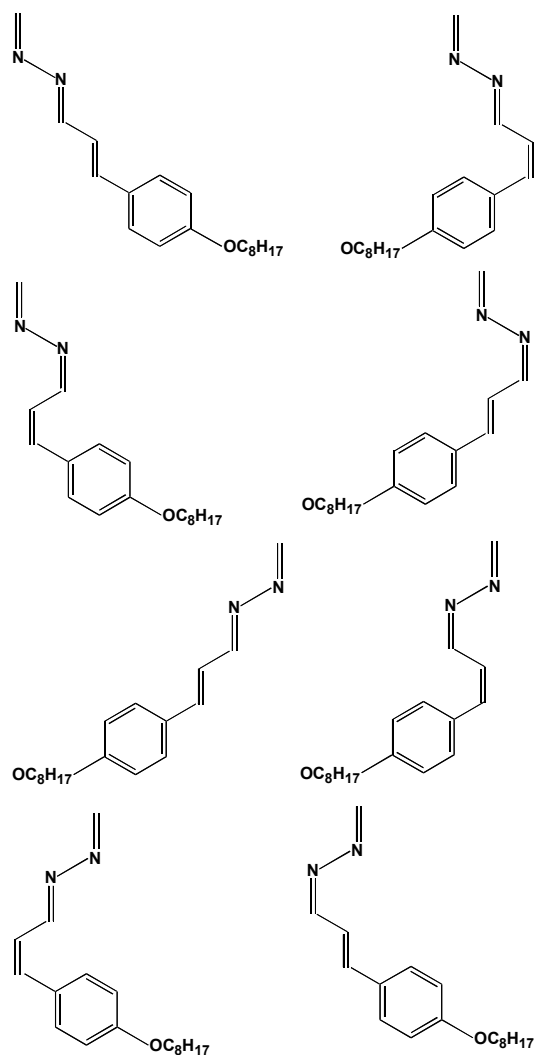
Fig.108. Isomères stériques possibles de la molécule Z-181.
