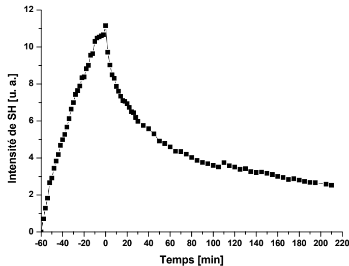
Fig.103. Dynamique d'évolution du signal de deuxième harmonique généré par l'échantillon constitué de IP-1077B-PVK. Au temps zéro la phase d'écriture a été arrêtée. Les temps négatifs sont associés à l'étude de la croissance de la susceptibilité \chi^{(2)} induite, les temps positifs – à l'étude de sa stabilité dans le temps.
