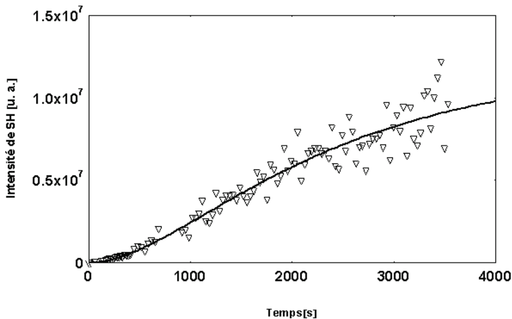
Fig.165. Croissance temporelle de l'intensité de second harmonique généré, en unités arbitraires, \Delta\Phi = 0^\circ . La courbe en continu est l'ajustement à l'équation y = a \times \left[1 - \exp\left(-\frac{x}{b}\right)\right]^2 . La saturation du signal est atteinte à 1,17802 \times 10^7 [u. a.], b = 1648,85 s.
