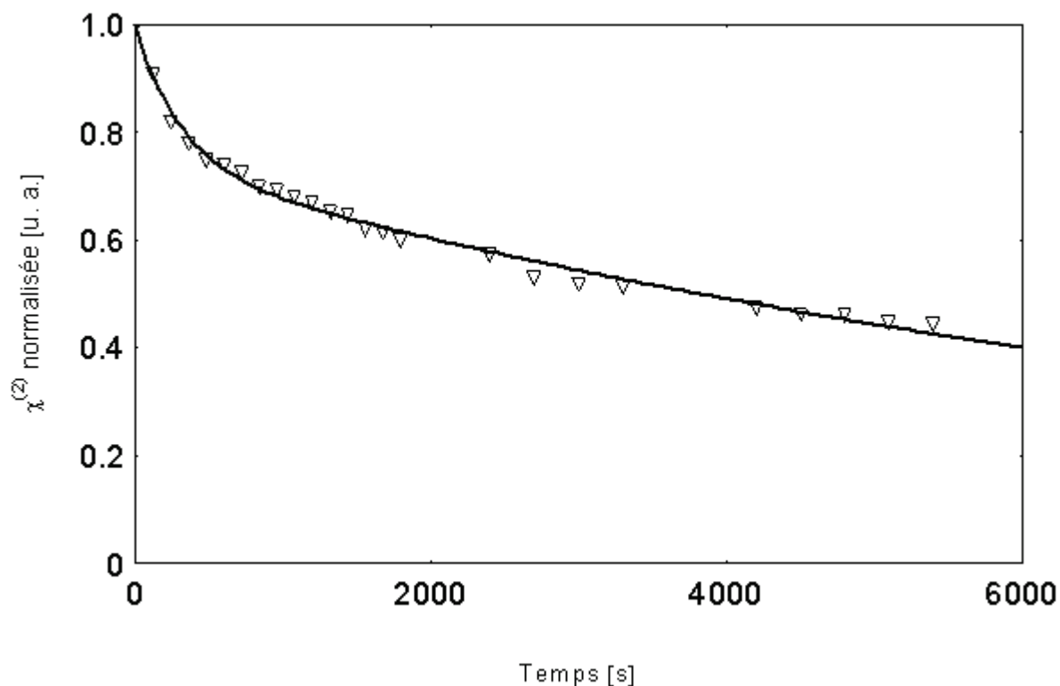
Fig.129. Décroissance de \chi^{(2)} normalisée, dans le film de IP-1077B-PMMA. La courbe en continu est l'ajustement théorique à l'équation (69), des mesures expérimentales.
