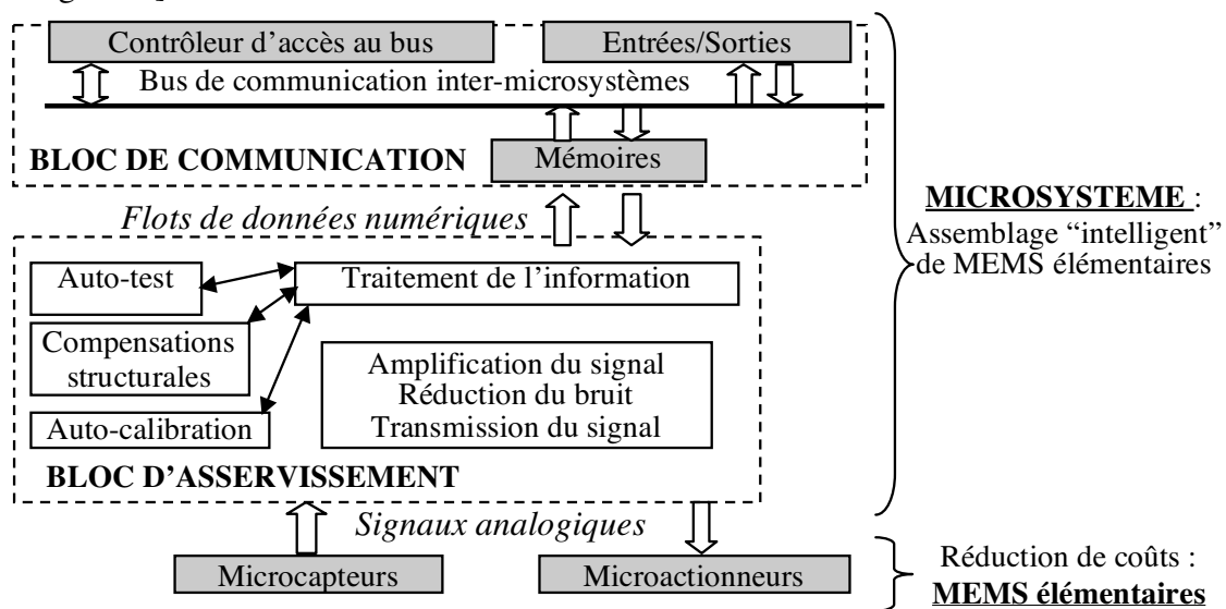
Figure 5.3 - Schéma fonctionnel d'un microsysteme
