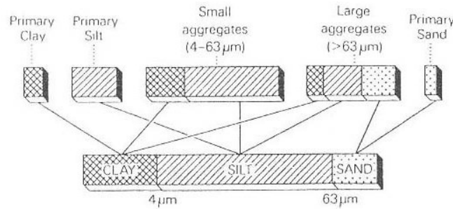
FIG. 1.25: Un exemple schématique pour illustrer l'estimation de la proportion en agrégats parmi les sédiments érodés à partir des relations développées par Foster et al. (1985) d'après Walling (1990)
