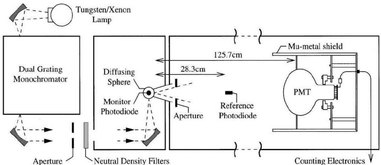
FIG. 6.2 – Montage créant une source contrôlée pour la calibration d'un PMT [BILLER + 99].
