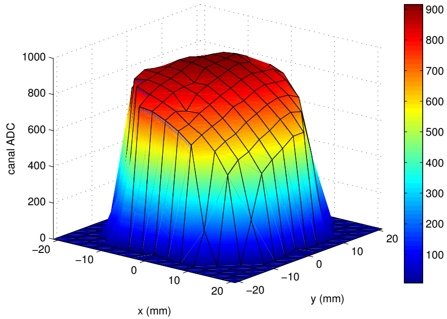
FIG. C.2 – Réponse du PMT-filtre vue en trois dimensions et dans les mêmes conditions que la figure C.1
