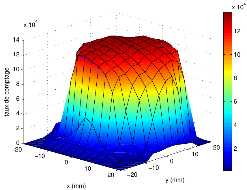
FIG. 6.11 – Réponse du PMT-filtre vue en trois dimensions et à haut gain, normalisée à la puissance lumineuse reçue par la photodiode.
