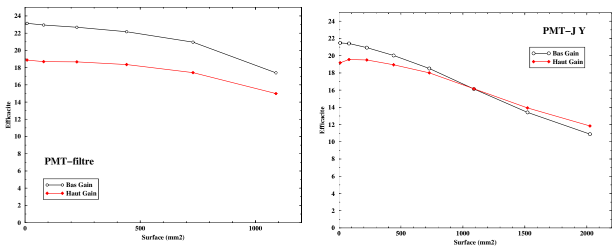
FIG. C.12 – Variation de l'efficacite du PMT-filtre (à droite) et du PMT-JY (à gauche), en fonction de la surface détectrice effective.
