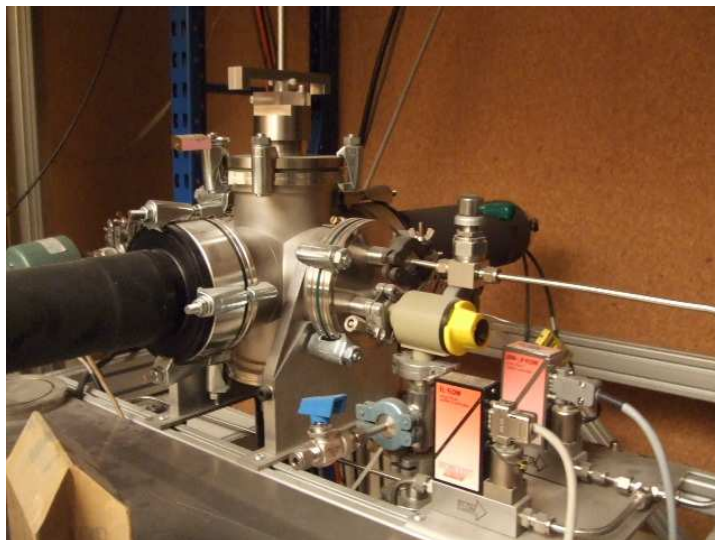
FIG. D.2 – Enceinte de fluorescence. Au premier plan, on distingue le tuyau d'arrivée du gaz. La vanne jaune permet soit de relier la croix à une pompe et d'y faire le vide, soit de faire une rentrée d'air. Contre le mur se trouve le PMT-filtre.
