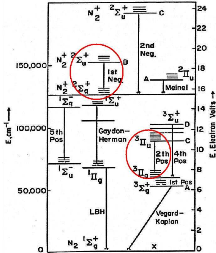
FIG. 2.1 – Diagramme des niveaux d'énergie de l'azote moléculaire. Les ensembles de transition entourés correspondent aux désexcitations produisant de la fluorescence, ce sont les systèmes 1N et 2P. Les niveaux notés X, A, B... sont les états électroniques, X marquant le fondamental. Les petits niveaux ajoutés aux états électroniques sont les dégénérescences en niveaux vibrationnels. [BUNNER64]
