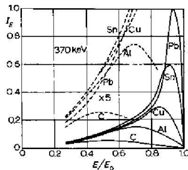
FIG. 4.13 – Spectre de la perte d'énergie d'électrons de 370 keV diffusés dans plusieurs matériaux, dont le plomb. On constate que les électrons de basse énergie y perdent environ 10 % de leur énergie [SIEGBAHN].
