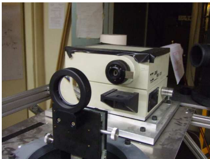
FIG. D.3 – Montage optique : la lentille se trouve au premier plan, et le spectromètre au second. Naturellement, la lentille et le chemin optique sont dans le noir pendant les mesures. La fente d'entrée du spectromètre est ouverte à 2 mm. On distingue le PMT-JY à la sortie du spectromètre.
