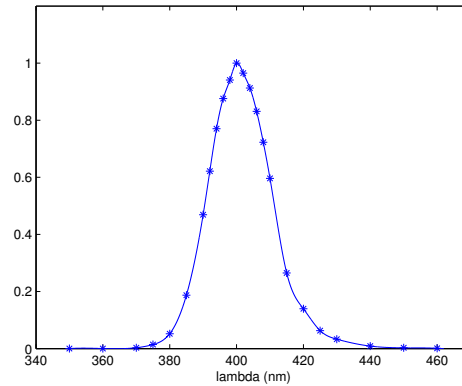
FIG. 6.17 – Courbe d’intensité d’une LED ETG-3UV400-30 en fonction de la longueur d’onde. Ces LED ont une puissance de 12 mW, ce qui permet une plus forte illumination. Celle-ci est nécessaire pour mesurer le rendement des deux sphères. Le spectre est normalisé à l’intensité la plus élevée. Il a été obtenu en mesurant l’intensité de la lumière de la matrice de LED en sortie du spectromètre, dont les fentes étaient ouvertes au maximum (2 mm).
