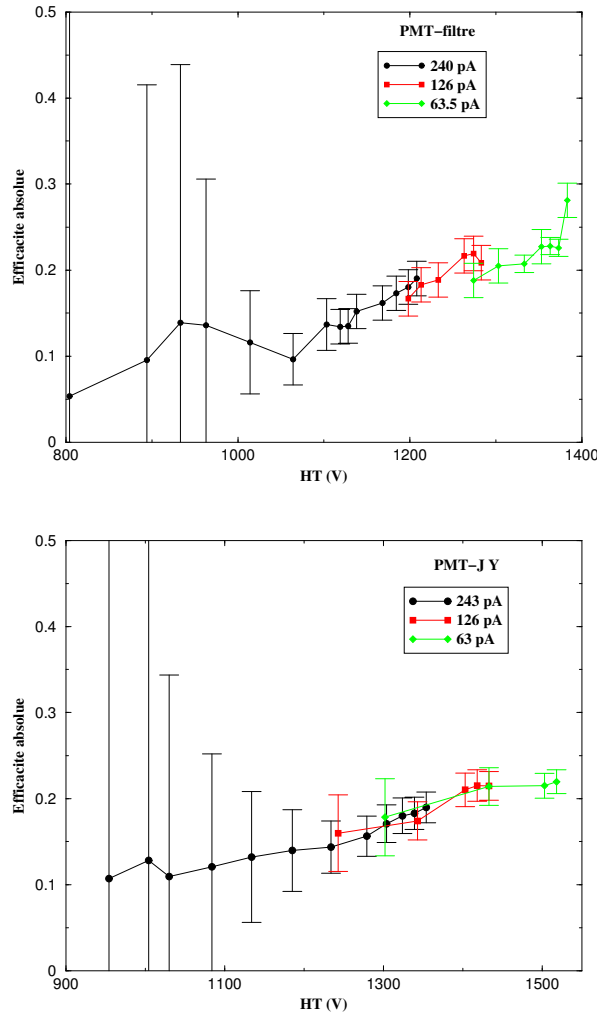
FIG. C.9 – Variation de l'efficacité de chaque PMT en fonction de la haute tension appliquée.
