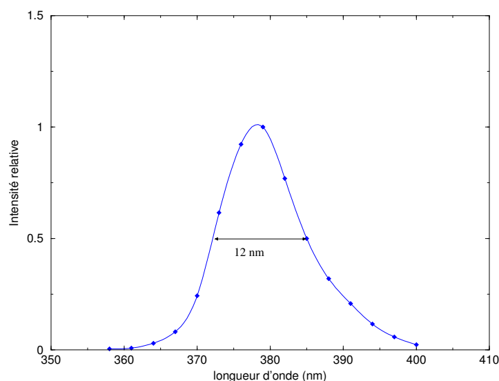
FIG. 6.4 – Spectre d’intensité relative de la LED RLT370-10 utilisée pour la calibration, mesuré avec le spectromètre. Les fentes d’entrée et de sortie sont ouvertes à 2 mm et contribuent pour 6 nm à la largeur observée. La largeur réelle de la LED est donc de 10 nm.
