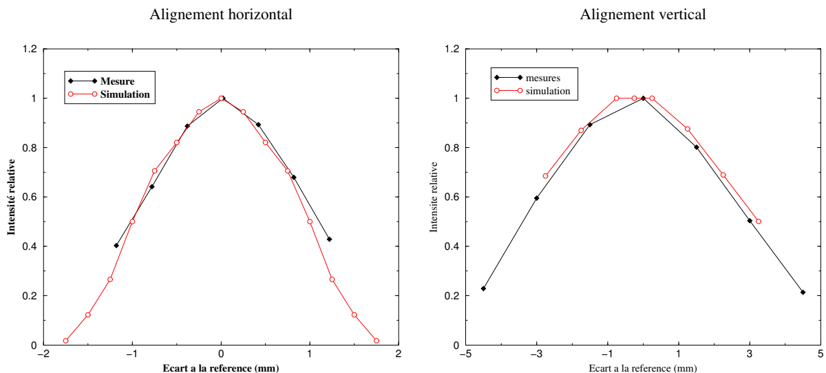
FIG. 5.2 – Résultats des mesures successives effectués pour aligner précisément la lentille transversalement (à gauche) et verticalement (à droite) sur le trajet des photons. L'origine de l'axe horizontal vient d'une position de référence, marquée sur l'axe de la vis micrométrique. Les mesures de la figure de droite (courbe noire) sont tout à fait compatibles avec la simulation (courbe rouge).
