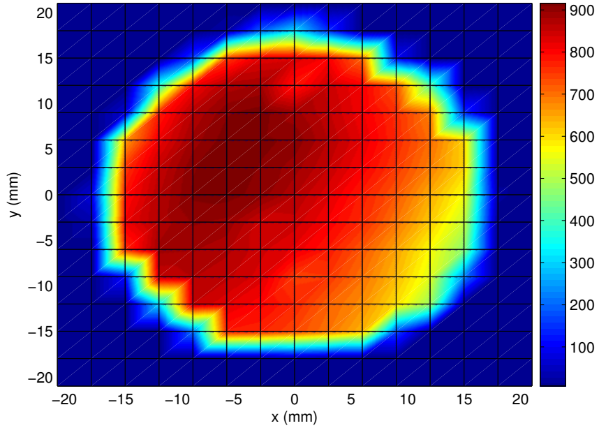
FIG. C.1 – Topographie du PMT-filtre à bas gain. La normalisation par rapport au flux lumineux mesuré par la photodiode est déjà effectuée.
