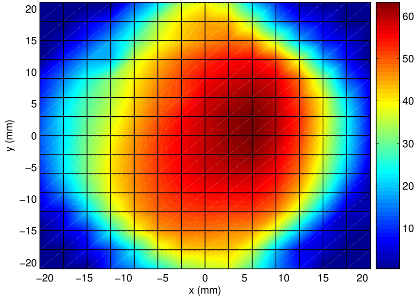
FIG. C.3 – Topographie du PMT-JY à bas gain, normalisée au flux lumineux détecté par la photodiode.
