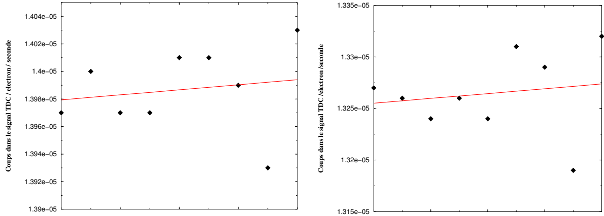
FIG. 7.2 – Variation des mesures intégrales à 1.1 MeV (à gauche) et à 1.5 MeV (à droite). L'ordonnée est directement proportionnelle au rendement de fluorescence. Les pentes de régression sont compatibles avec une constante (pente horizontale).
