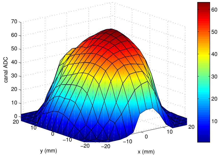
FIG. C.4 – Réponse du PMT-JY vue en trois dimensions, dans les mêmes conditions que sur la figure C.3
