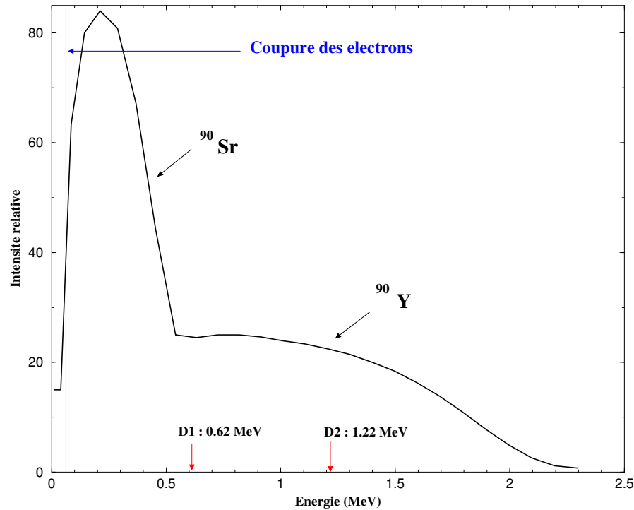
FIG. 4.2 – Spectre \beta du strontium et de l'yttrium. L'énergie maximale est 2.28 MeV. (référence : [HANSEN + 83])
