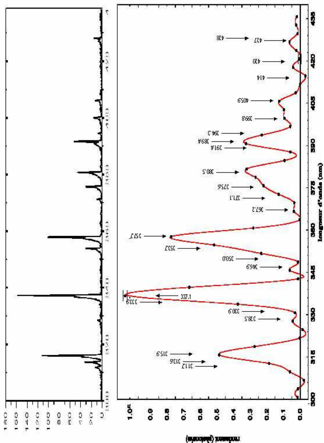
FIG. 7.8 – Dans la partie inférieure, spectre de fluorescence mesuré à pression atmosphérique, avec des fentes ouvertes à 2 mm. Il y a une mesure tous les 3 nm. La partie supérieure montre, à titre de comparaison, le spectre mesuré par Ulrich [air] à plus basse énergie.
