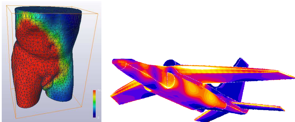
(a) Hyperthermie (échauffement local des tissus) RF (27MHz) pour le traitement de tumeurs profondes. Module du champ électrique. (b) Illumination (excitation) d'un avion par une onde plane 100Mhz. Répartition de la densité de courant.
