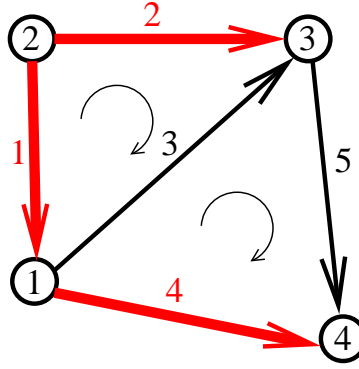
FIG. 4.2 – Sous-graphe \mathcal{S}^{H,i} (voir figure 4.1). Un arbre couvrant est en trait fort rouge. Pour les deux cycles indépendants, l'orientation est représentée.
