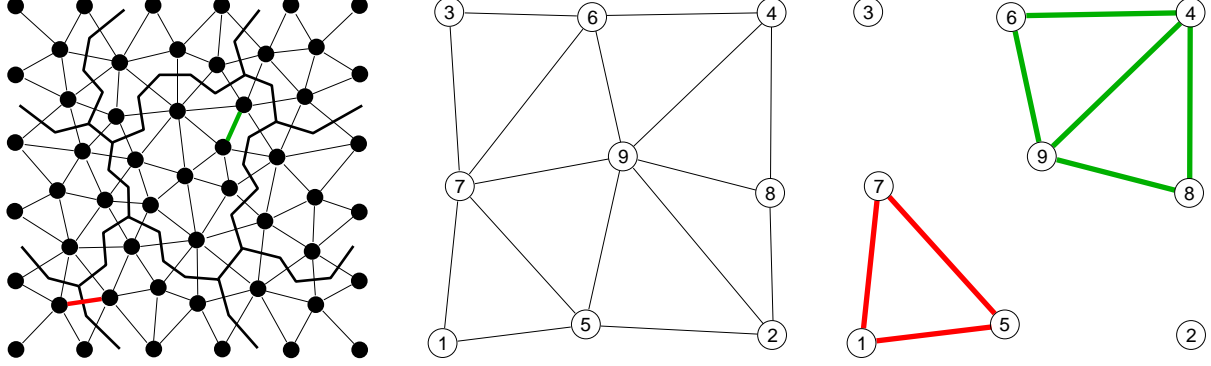
FIG. 4.1 – Partition, graph grossier et les sous-graphes \mathcal{S}^{H,i} et \mathcal{S}^{H,j} .
