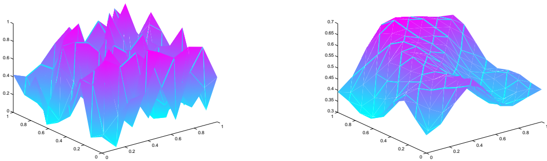
FIG. 2.1 – Erreur initiale et lissée après 2 itérations de Gauss-Seidel.
