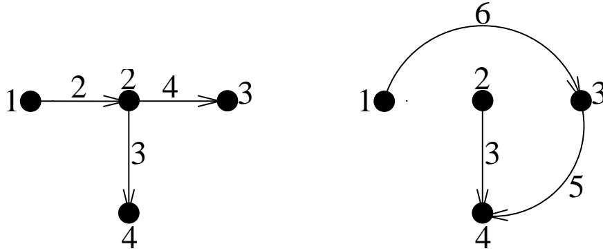
FIG. 1.5 – Deux arbres couvrants pour le graphe de la figure 1.4(b).
