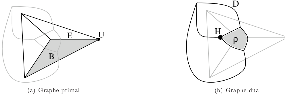
FIG. 1.10 – Graphes primal et dual - Grandeurs physiques associées aux composantes des graphes.
