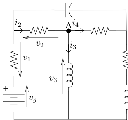
FIG. 1.3 – Exemple de réseau électrique.
