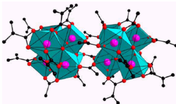
Figura 2.1.6: Representação do cluster [\text{Zr}_6\text{O}_4(\text{OH})_4(\text{OMc})_7(\text{OAc})_5]_2 , com estrutura semelhante ao da figura anterior. [extraído de SCHUBERT, 2004]
