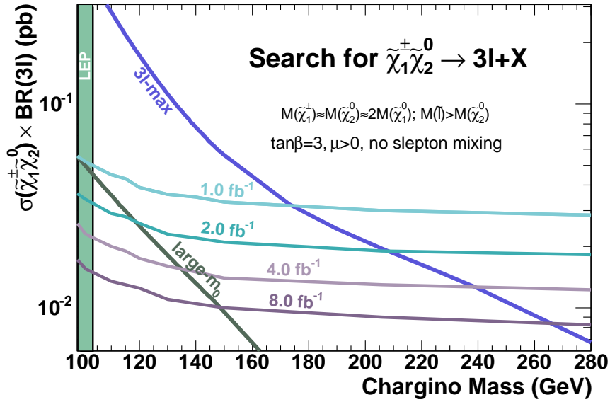
FIG. 7.16 – Limites attendues pour \sigma(p\bar{p} \rightarrow \tilde{\chi}_1^\pm \tilde{\chi}_2^0) \times BR(3l) en fonction de la masse du premier chargino pour des luminosités de 1, 2, 4 et 8 \text{fb}^{-1} . Cette dernière valeur correspond à la luminosité attendue par expérience à la fin de la phase II.
