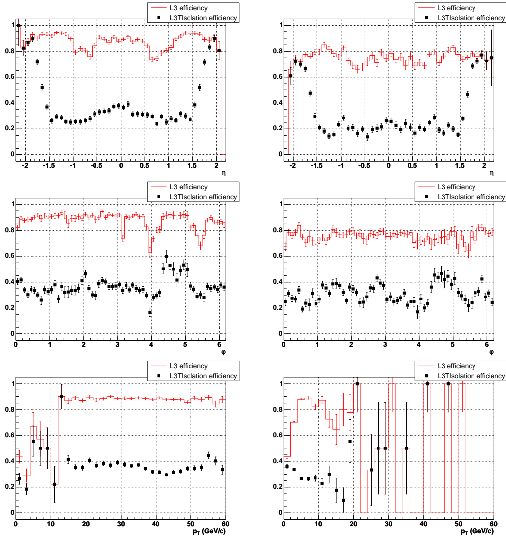
FIG. 5.15 – Efficacités en considérant les lots Z (gauche) et J/\psi (droite). De haut en bas sont présentées les efficacités en fonction de \eta , \phi et p_T du muon reco. L'efficacité de l'outil Muon est illustrée par une ligne rouge est celle correspondant à l'outil ISO_MUON par des carrés noirs. Une perte de 60% en efficacité est observée pour le critère p_T^{halo} < 2.5 GeV/c.
