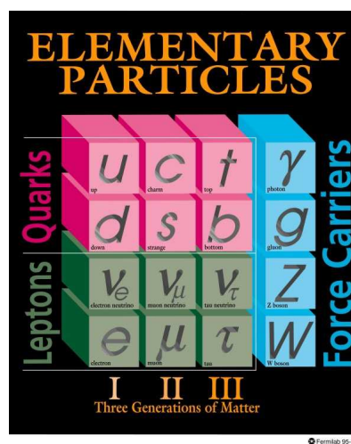
FIG. 1.1 – Particules constituantes du modèle standard. Nous distinguons les trois familles de fermions ainsi que les quatre bosons de jauge.
