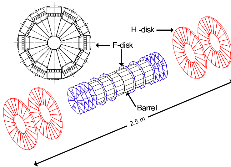
FIG. 4.4 – Vue tridimensionnelle du SMT. Nous distinguons les six tonneaux et les seize disques.
