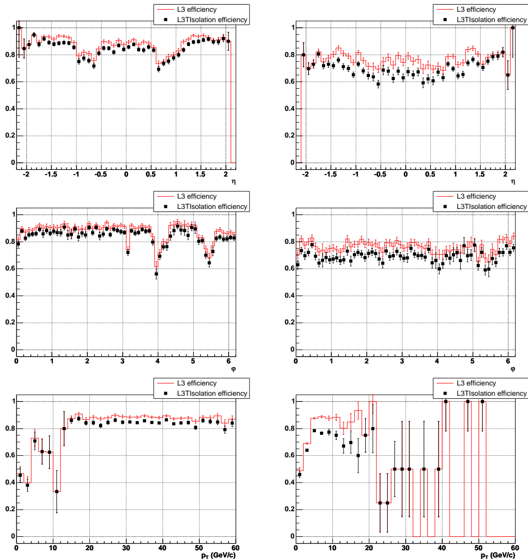
FIG. 5.13 – Efficacités en considérant les lots Z (gauche) et J/ \psi (droite). De haut en bas sont présentées les efficacités en fonction de \eta , \varphi et p_T du muon reco. L'efficacité de l'outil Muon est illustrée par une ligne rouge est celle correspondant à l'outil ISO_MUON par des carrés noirs. Des pertes d'efficacité de 4.1% et 9.4% sont respectivement observées pour les lots Z et J/ \psi en appliquant le critère E_T^{halo} < 2.5 GeV.
