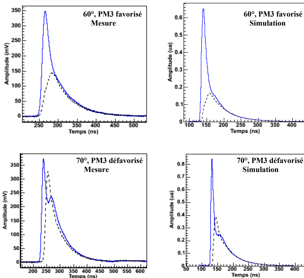
Figure B-43 : Traces moyennes mesurées (gauche) et simulées (droite) des 3 PM pour 60^\circ avec le PM3 favorisé (haut) et pour 70^\circ avec le PM3 défavorisé. Les courbes en trait plein correspondent aux traces moyennes du PM3 et celles en pointillé au PM1.
