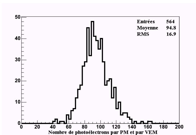
Figure B-31 : Estimation du nombre moyen de photoélectrons par VEM pour 564 photomultiplicateurs des détecteurs du réseau de surface [b-70].
