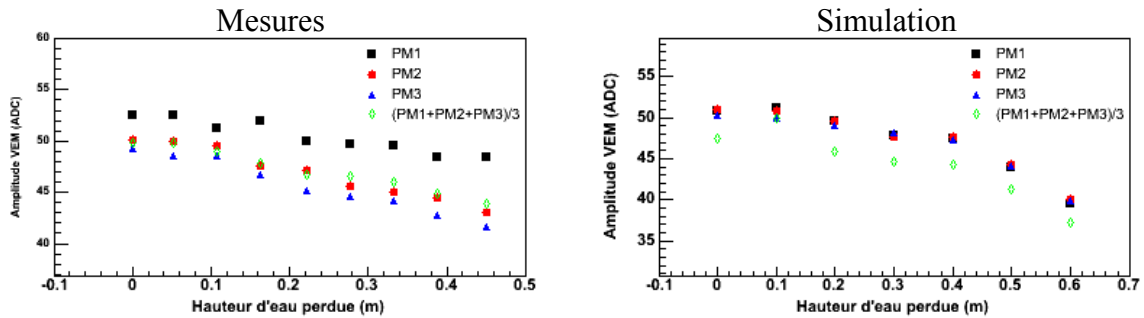
Figure B-51 : Graphes de gauche : évolution de l'amplitude d'un VEM mesurée sur le détecteur CAPISA en fonction de la hauteur d'eau perdue. Graphes de droite : prédictions de la simulation.
