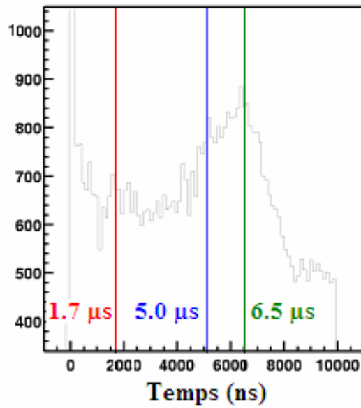
Figure A-45 : Distribution temporelle des impulsions secondaires très retardées sans la présence du pic primaire à 1 pe. Les mesures ont été faites sur le PM XP1806 n°881 à un gain de 2 \cdot 10^6 .
