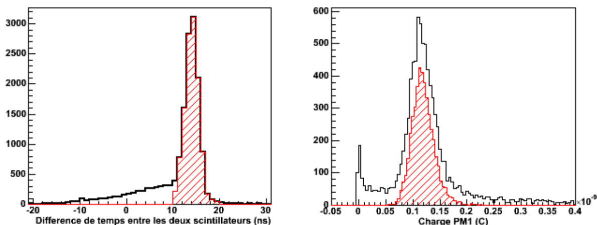
Figure B-39: Graphe de gauche : histogramme de la différence de temps entre les deux scintillateurs pour un angle de 60 °. Les événements gardés après la coupure sur la différence de temps sont en hachuré. Le temps de vol théorique des muons entre les deux scintillateurs est de 15 ns. Graphe de droite : effet de la coupure en temps sur l'histogramme en charge du PM1.
