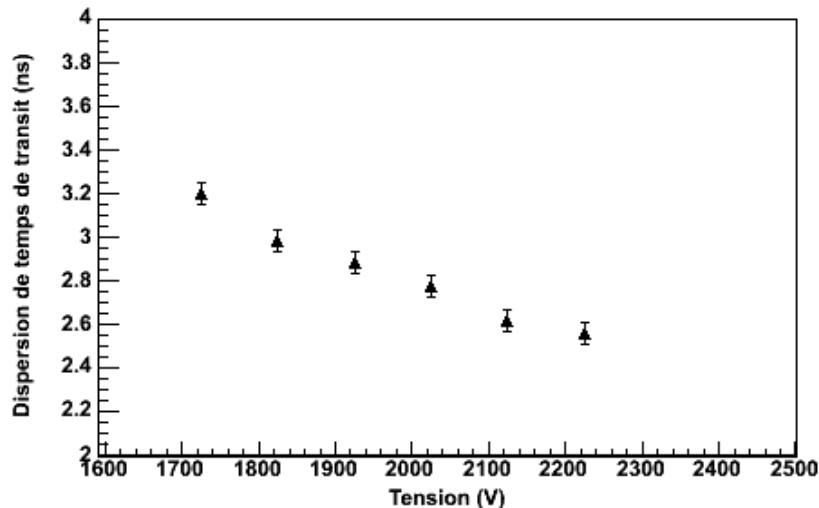
Figure A-34 : Dispersion de temps de transit (FWHM) en fonction de la tension d'alimentation pour le PM XP1806 n°810 avec une embase avec 10 Vs dans l'optique d'entrée. Les mesures ont été faites sans le diaphragme. La contribution de la source a été enlevée.
