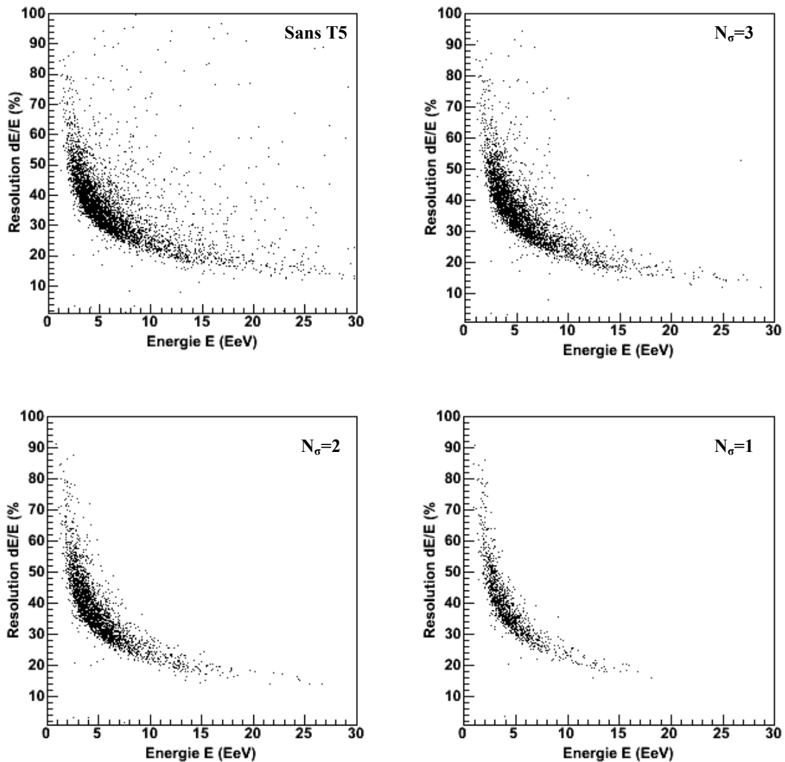
Figure B-95 : Résolution dE/E en fonction de l'énergie E (en EeV). En haut et à gauche : pas de critère de qualité. En haut, à droite : sélection T5 avec une coupure à 3 sigmas. En bas, à gauche : sélection T5 avec une coupure à 2 sigmas. En bas, à droite : sélection T5 avec une coupure à 1 sigma.
