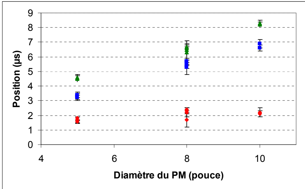
Figure A-86 : Position des 3 principaux pics de post impulsions en fonction du diamètre pour trois PM de 5 pouces (XP1803 n°851, 865 et 866), quatre PM de 8 pouces (XP1806 n°810, 816, 869 et 873) et deux PM de 10 pouces (XP1804 n°885 et 887).
