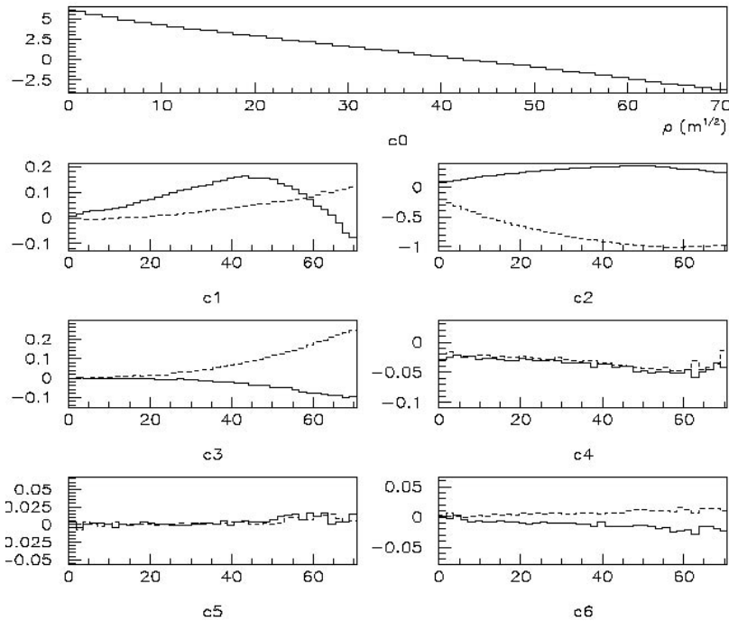
Figure B-79 : Coefficients de Fourier en \psi de \ln(N_{\mu}) en fonction de \rho = \sqrt{r} pour une gerbe initiée par un proton de 10^{20} eV, \theta=80^\circ , \varphi=90^\circ . Lignes solides : coefficients A_j . Lignes pointillées : B_j [b-83].
