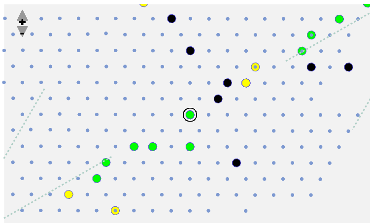
Figure B-87 : Evènement n°2261962 à 85^\circ avec environ 14 stations touchées non sélectionné par le T4 standard (4C1) et par le T4exp. Les stations T2 sont en vert, les T1 en jaune et celles qui ne fonctionnent pas en noir.
