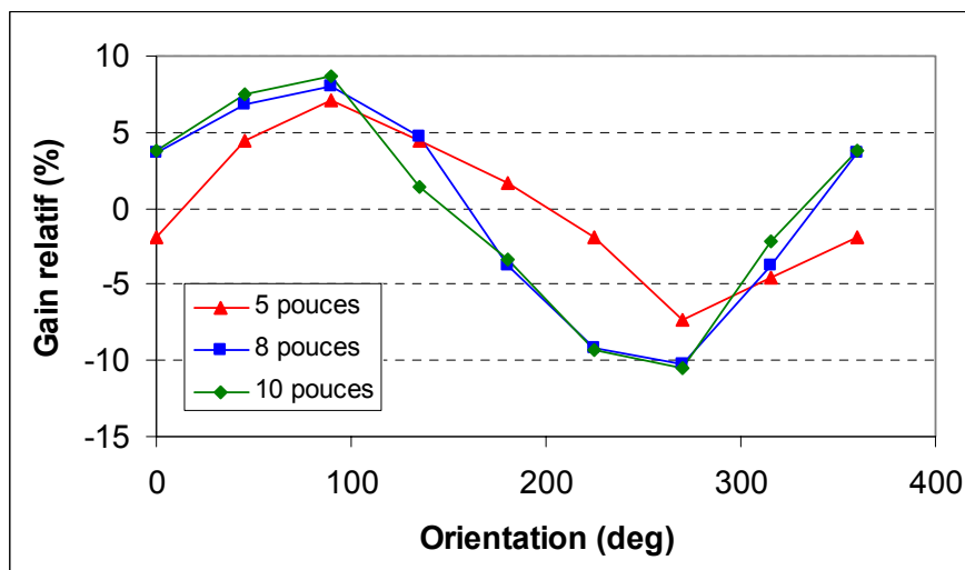
Figure A-83 : Evolution du gain relatif en fonction de l'orientation du PM. Le zéro correspond à la broche "sp" orientée vers le Nord. Le sens de rotation est celui inverse des aiguilles d'une montre.
