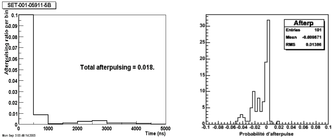
Figure A-66 : Exemple de distribution temporelle des AF II pour le XP1805 n° 5911 – Distribution des probabilités de ces post impulsions pour 100 PM.
