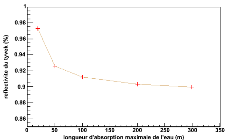
Figure B-34 : Valeurs des paramètres de la simulation (longueur d'absorption de l'eau et réfectivité du Tyvek) pour avoir un temps de décroissance du signal d'un VEM d'environ 50 ns (détecteur d'Orsay).
