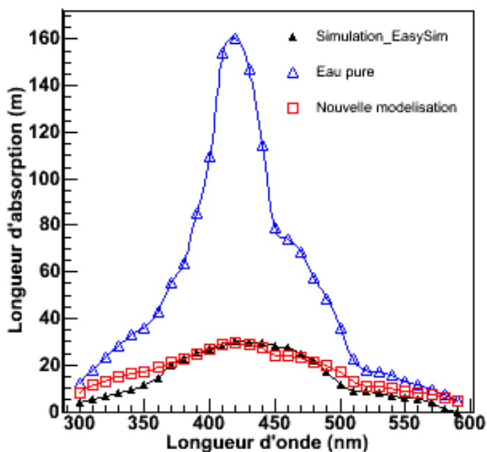
Figure B-36 : Dépendance de la longueur d'absorption de l'eau en fonction de la longueur d'onde pour l'eau pure (triangle creux, mesure R.M. Pope et E.S. Fry en 1997 [b-72]), utilisée dans la simulation EasySim (triangle plein) et pour la nouvelle modélisation (carré creux).
