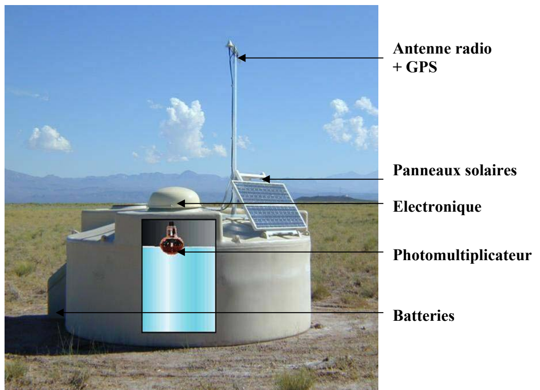
Figure B-11 : Photographie d'un détecteur du réseau de surface.
