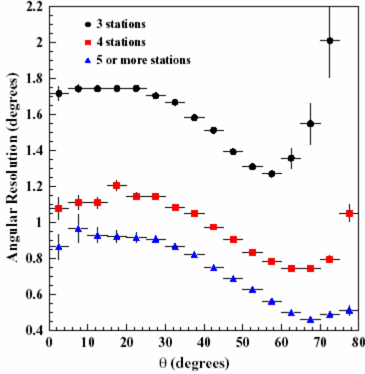
Figure B-91 : Résolution angulaire en fonction de l'angle de la gerbe pour différentes multiplicités [b-95].
