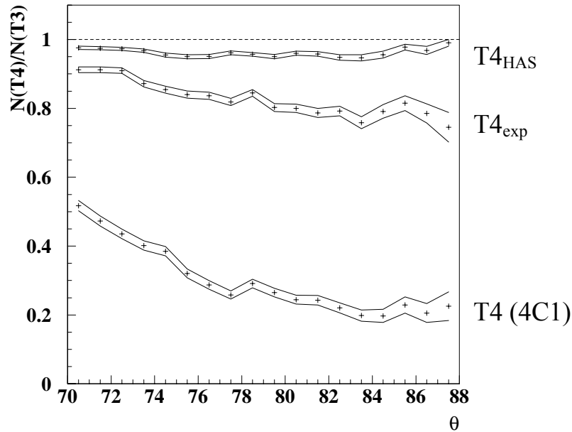
Figure B-90 : Nombre d'événements sélectionnés par les différents critères normalisés au nombre d'événements T3 (tous les événements T3 sont physiques et reconstituables).
