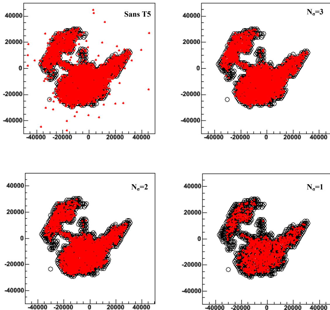
Figure B-94 : Position du cœur de tous les évènements horizontaux dans les données 2005 et 2006. En haut et à gauche : pas de critère de qualité. En haut, à droite : sélection T5 avec une coupure à 3 sigmas. En bas, à gauche : sélection T5 avec une coupure à 2 sigmas. En bas, à droite : sélection T5 avec une coupure à 1 sigma. Les cercles noirs représentent la position de toutes les stations présent en juin 2006.
