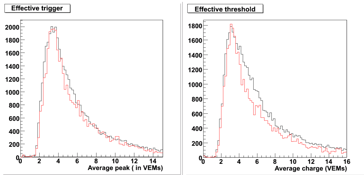
Figure B-83 : Histogrammes de l'amplitude moyenne (graphe de gauche) et de la charge moyenne (graphe de droite) pour deux sélections angulaires d'événements : 70-80^\circ (trait plein) et 80-90^\circ (pointillé).
