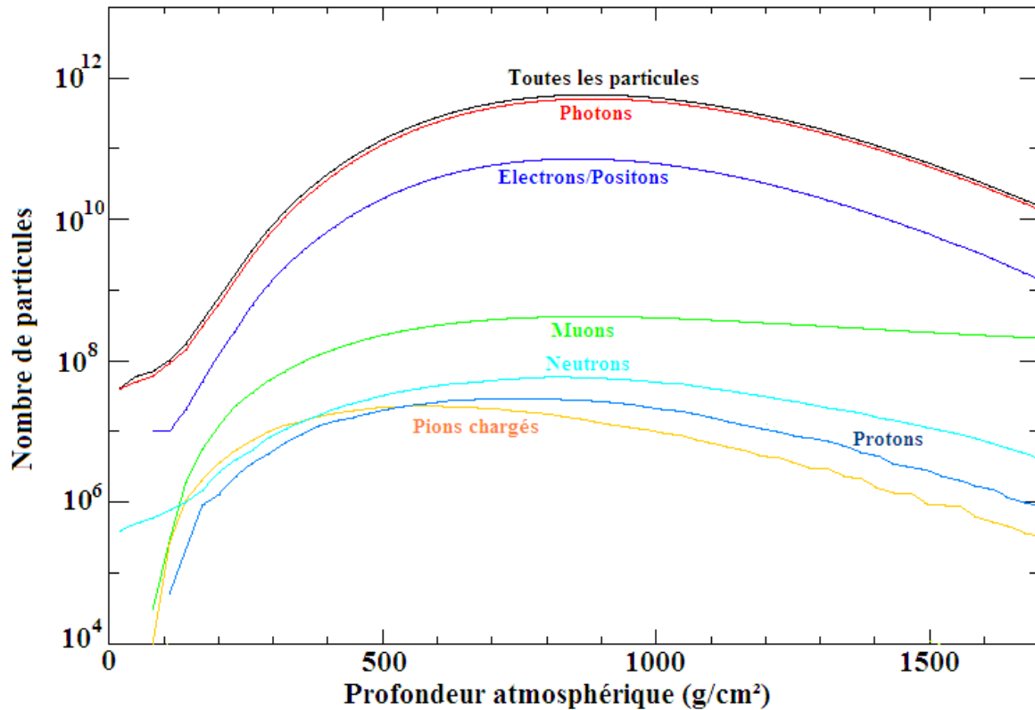
Figure B-6 : Nombre de particules en fonction de la profondeur atmosphérique traversée, pour une gerbe de proton ayant une énergie de 10^{20} eV et un angle zénithal de 60^\circ simulée avec AIRES [b-14].
