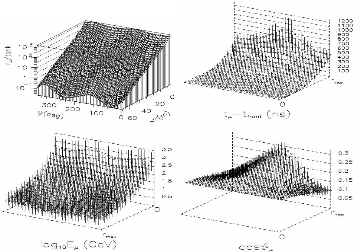
Figure B-78 : Tabulations pour une gerbe de proton à une énergie de 10^{20} eV avec \theta=80^\circ , \varphi=90^\circ en fonction \sqrt{r} et \psi . Les barres d'erreur indiquent les dispersions. En haut, à gauche : nombre moyen de muons par station. En bas, à gauche : énergie déposée en GeV (échelle logarithmique). En haut, à droite : temps d'arrivée. En bas, à droite : divergence angulaire au sol [b-83].
