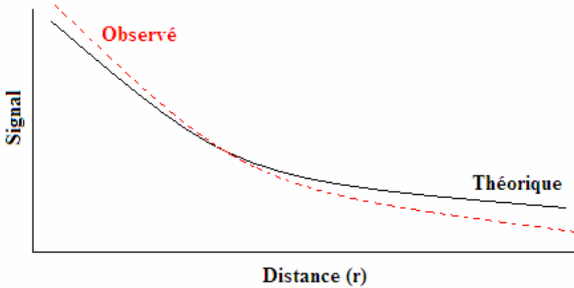
Figure B-107 : Illustration des profils moyens à un angle \psi donné observé dans les données (en pointillé) et prédit par les simulations pour un angle zénithal inférieur à 80^\circ (angle \psi=0 ).
