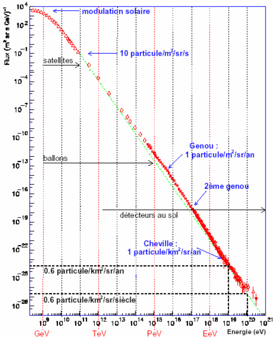
Figure B-1 : Spectre en énergie des rayons cosmiques : flux différentiel en \text{m}^{-2}.\text{s}^{-1}.\text{sr}^{-1}.\text{GeV}^{-1} en fonction de l'énergie. La ligne pointillée représente une loi de puissance avec un indice spectral de 2.7.
