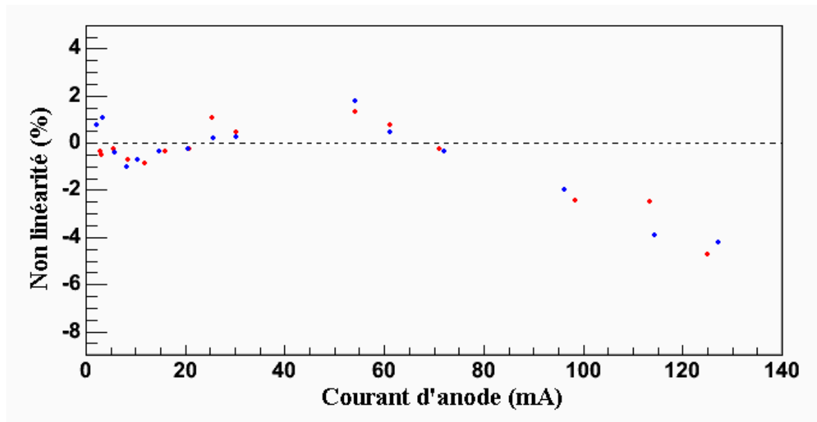
Figure A-48 : Deux courbes de linéarité en charge en fonction du courant moyen d'anode pour le PM XP1806 n°816 à un gain de 10^7 avec une embase « 20 Vs » (mesures faites à l'INFN de Turin [a-53]).
