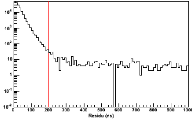
Figure B-88 : Histogrammes des résidus en temps obtenus avec des événements simulés. Le « talon » correspond aux fortuites. Pour enlever les fortuites, une coupure est appliquée à 200 ns (trait rouge).
