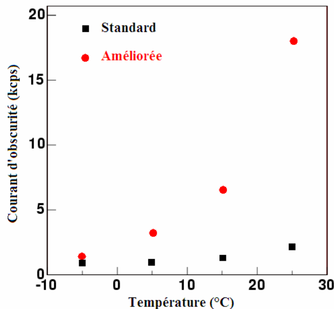
Figure A-74 : Dépendance en température du courant d'obscurité pour un PM standard (carré noir) et pour un PM avec la nouvelle photocathode (cercle rouge).
