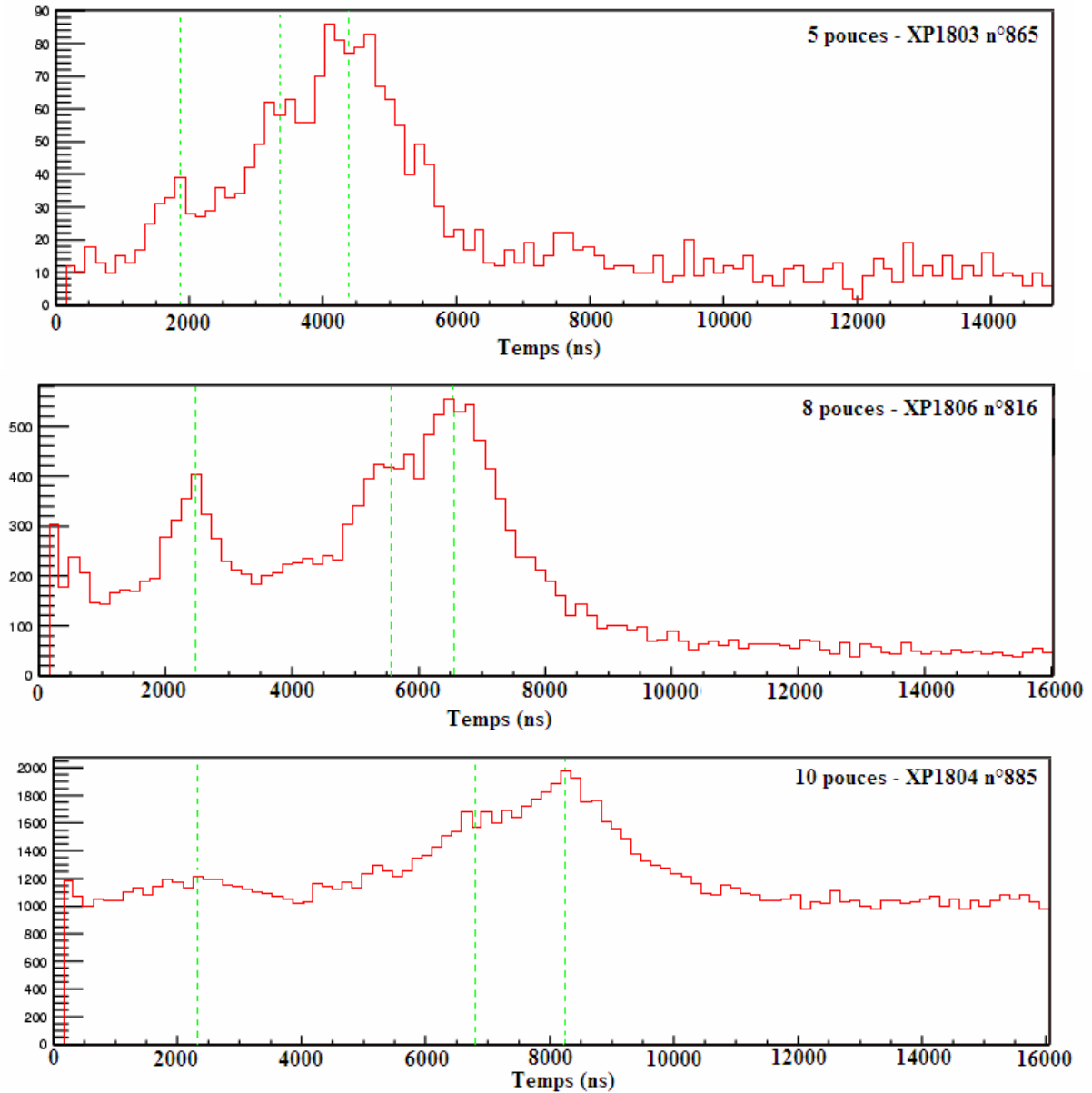
Figure A-85 : Distributions temporelles des pics secondaires pour un PM de 5 pouces (XP1803 n°865), un PM de 8 pouces (XP1806 n°810) et un PM de 10 pouces (XP1804 n°887). Les pointillés indiquent la position des 3 principaux pics.
