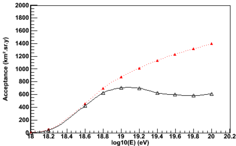
Figure B-99 : Acceptance horizontale en fonction de l'énergie pour tous les événements horizontaux sélectionnés par le T3 (pointillé) et par toute la chaîne de reconstruction (T4 + reconstruction + T5) entre le 01/01/05 et le 30/06/06.
