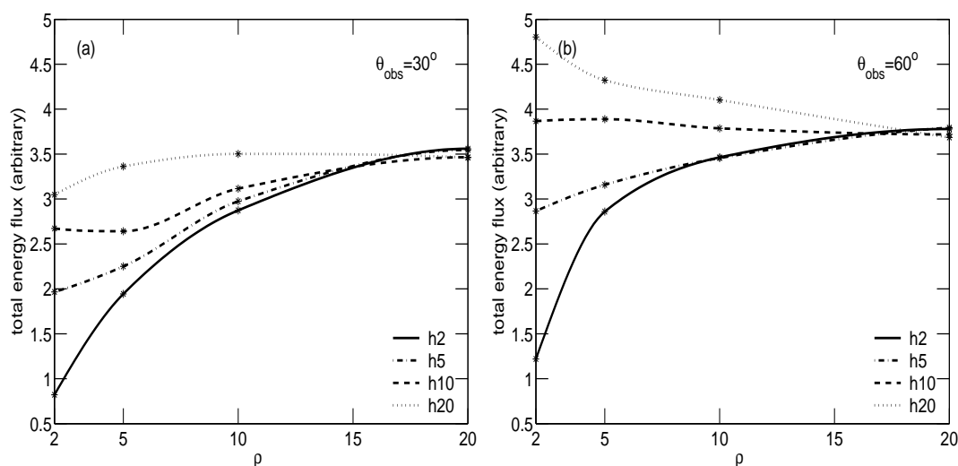
FIG. 2.12 – Flux total en énergie du modèle GR entre 1 et 30 keV, en fonction de \rho , pour différents h et un angle d'observation de 30^\circ (a) et 60^\circ (b).
