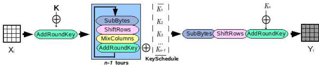
FIG. 1.6 – L'algorithmme AES
